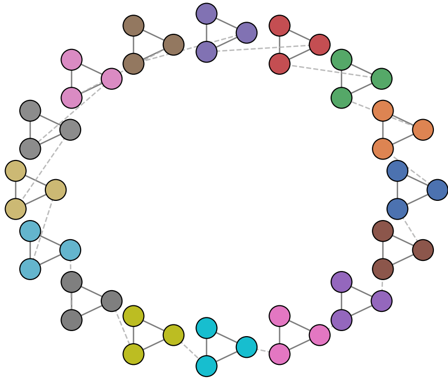
(a) Phân hoạch tự nhiên: mỗi clique một cụm Q = 0.6875
