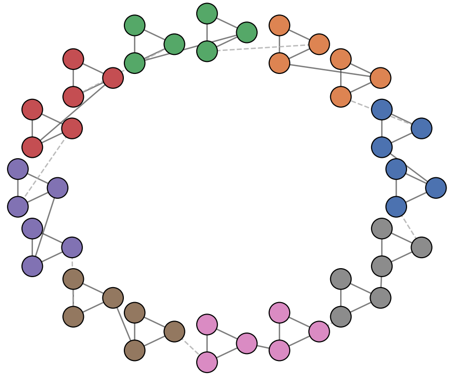
(b) Phân hoạch tối ưu modularity: gộp từng cặp clique Q = 0.7500
