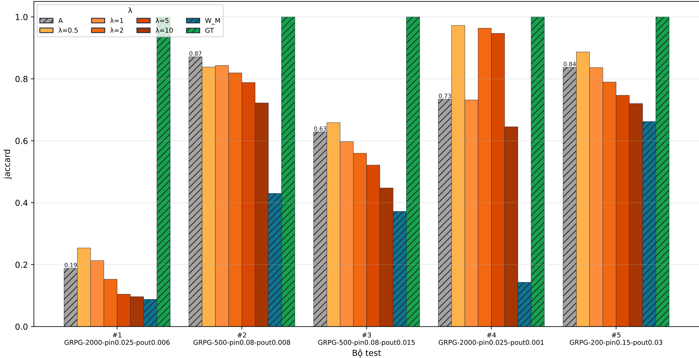
[GRPG] compare_to_GT · jaccard
