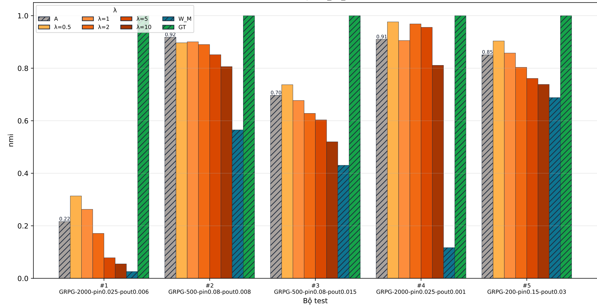
[GRPG] compare_to_GT · nmi
