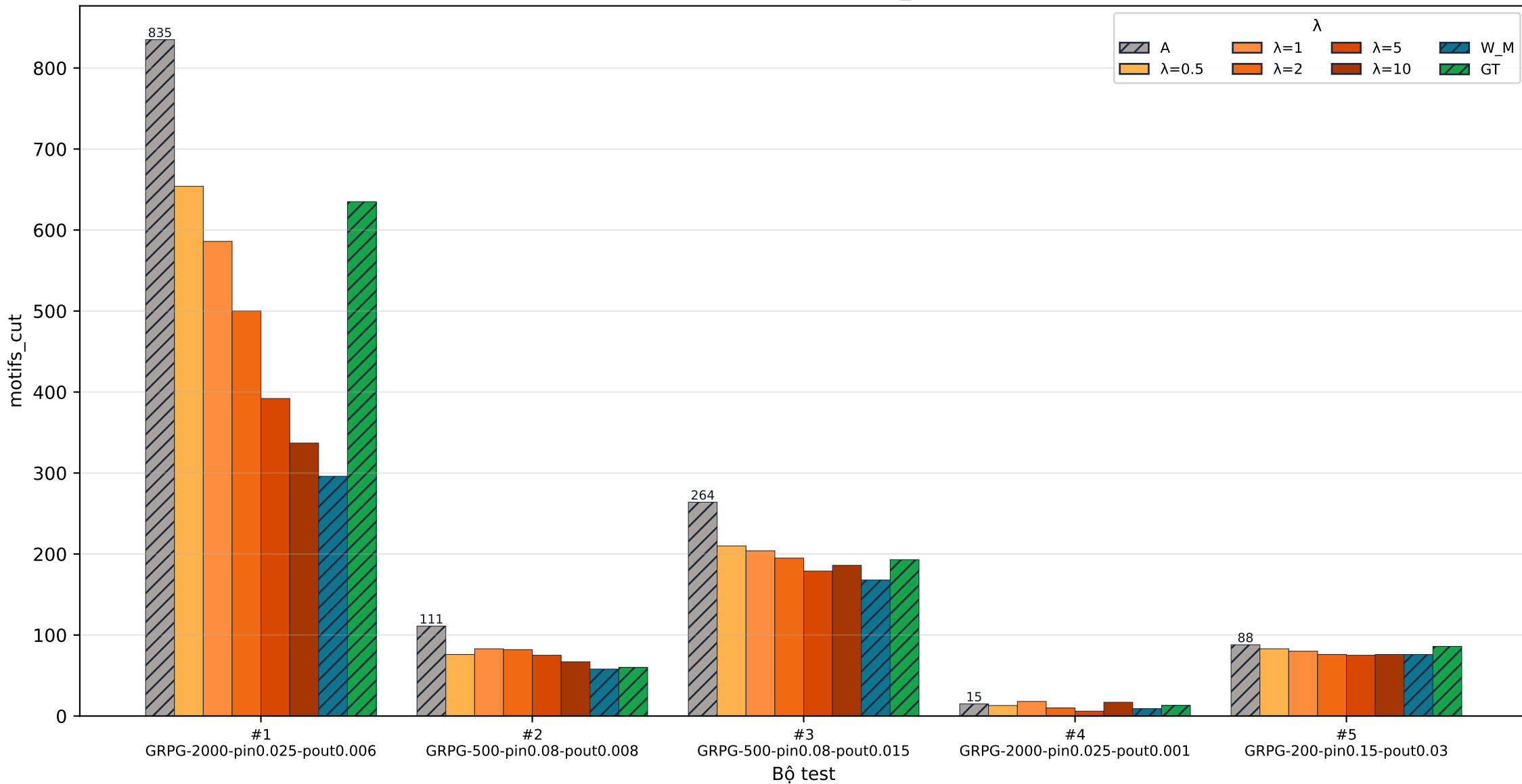
[GRPG] cut · motifs_cut
