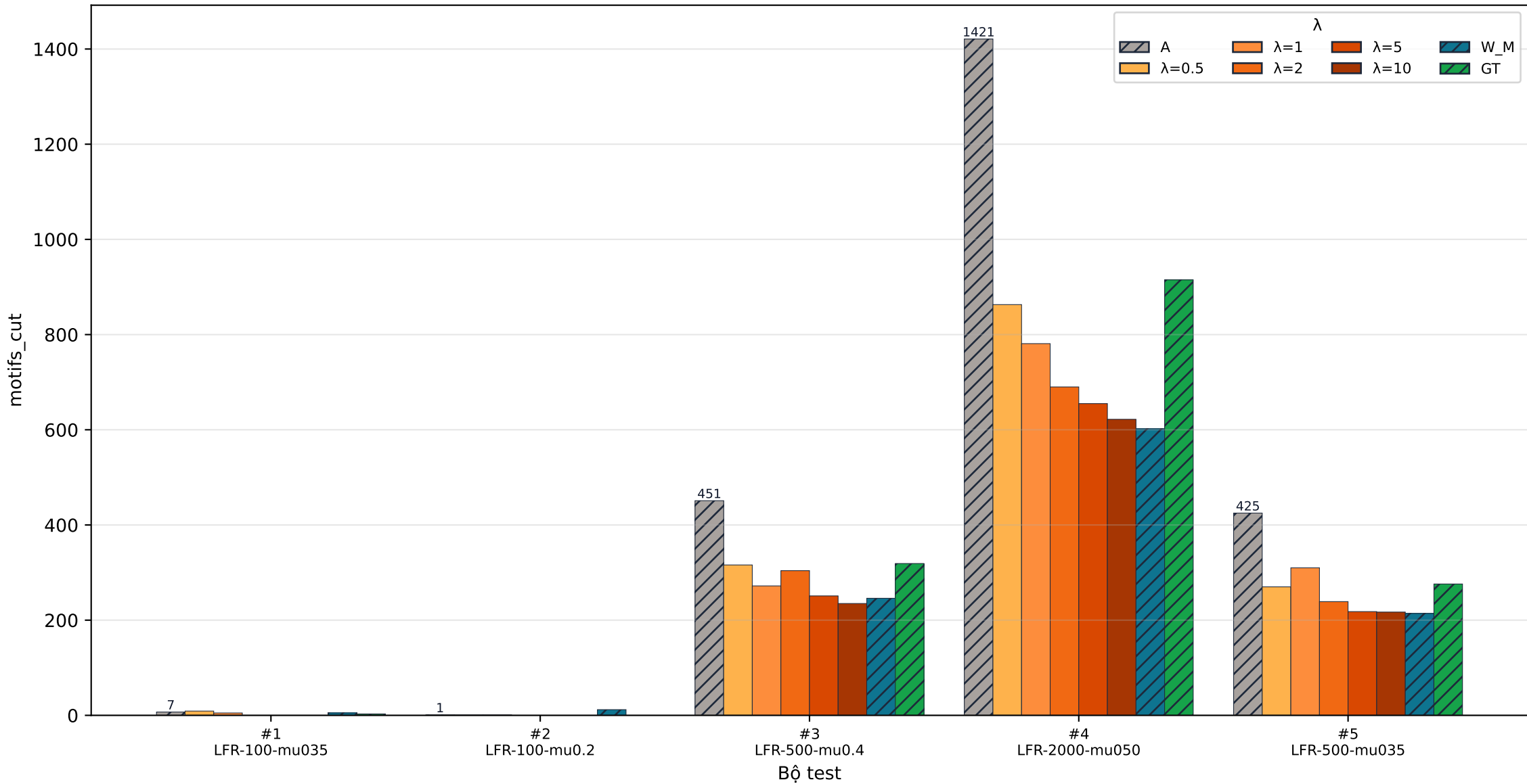
[LFR] cut · motifs_cut
