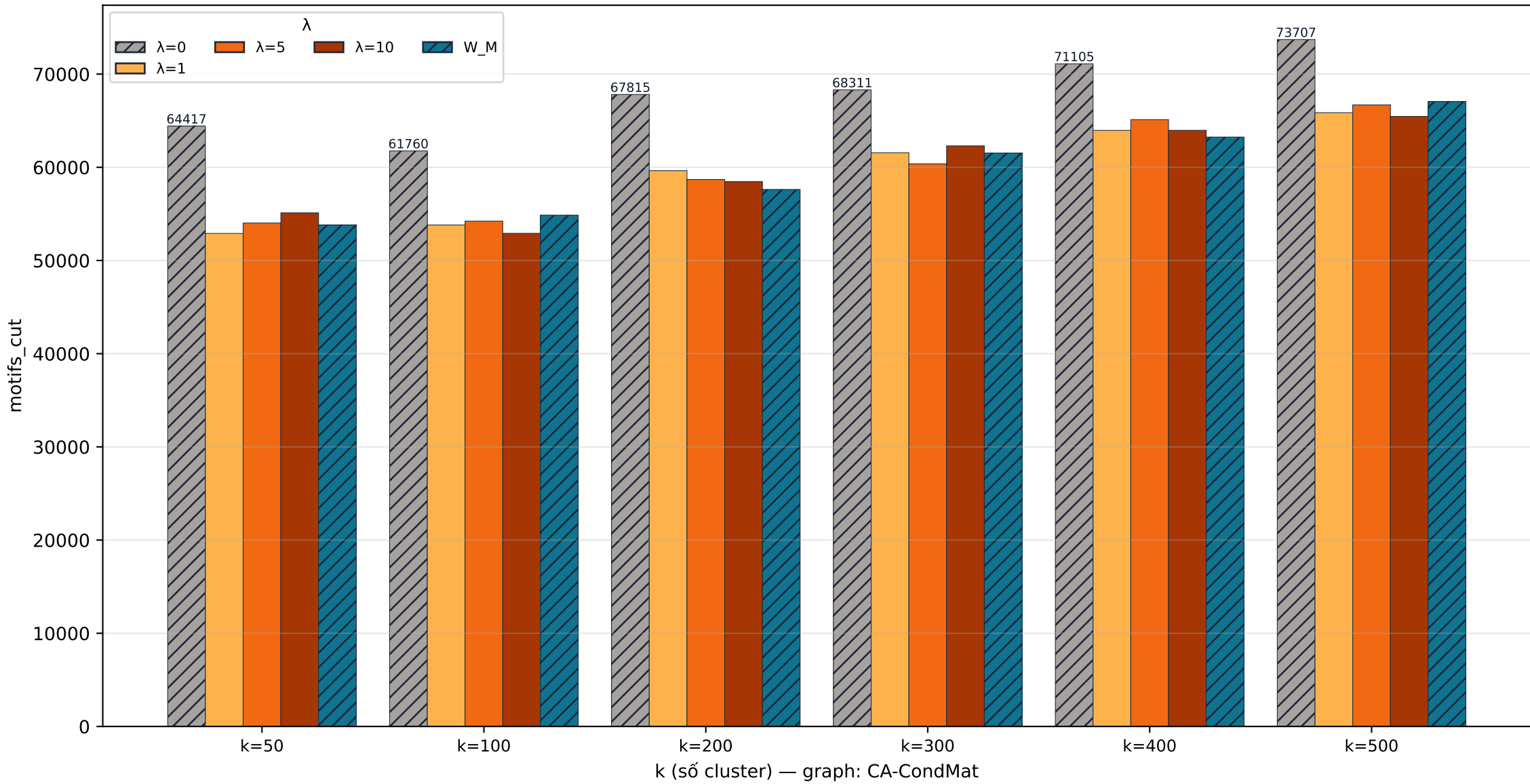
CA-CondMat cut · motifs_cut
