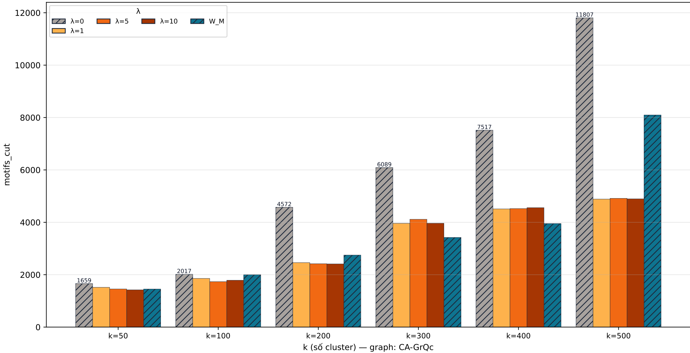
CA-GrQc cut · motifs_cut
