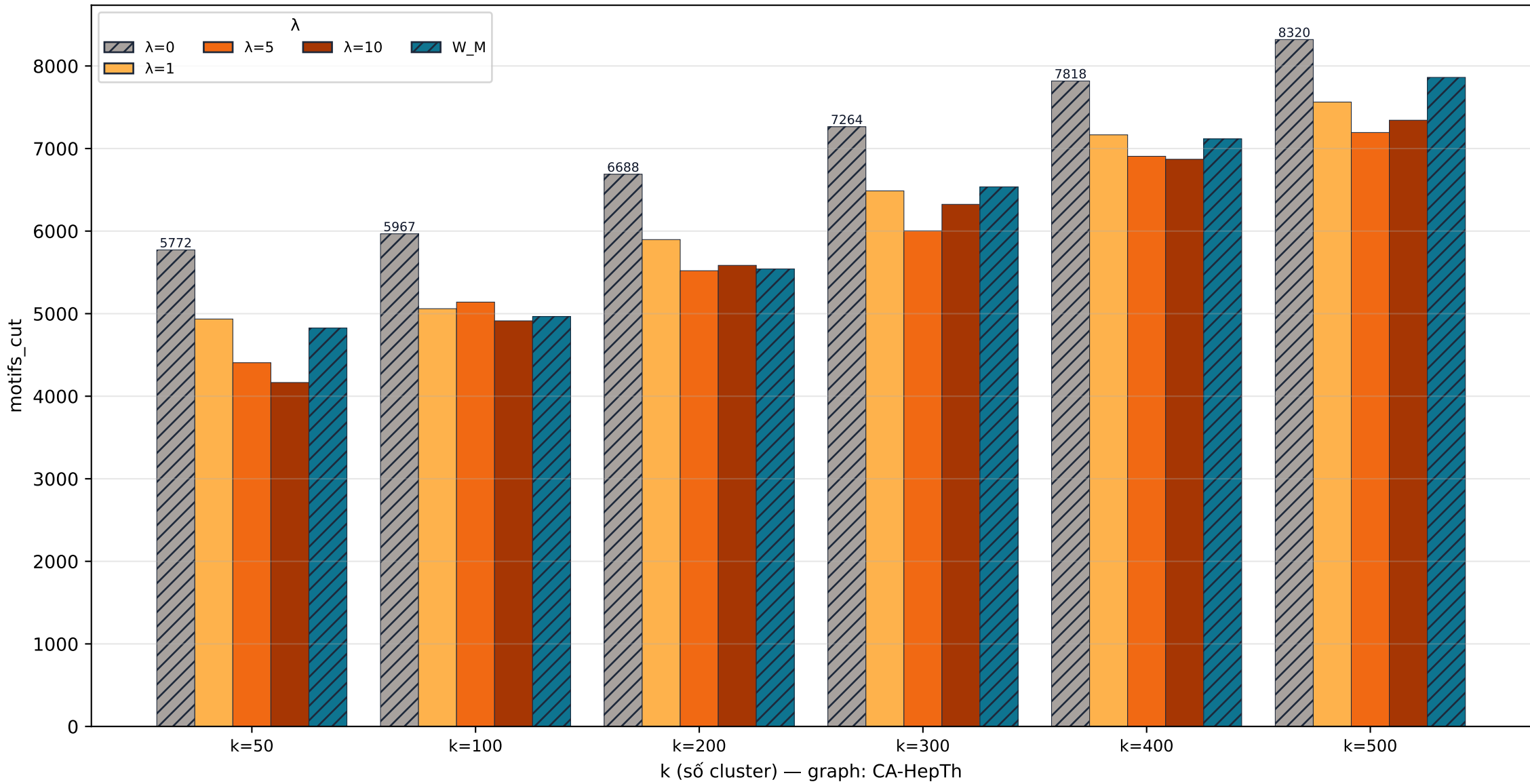
CA-HepTh cut · motifs_cut
