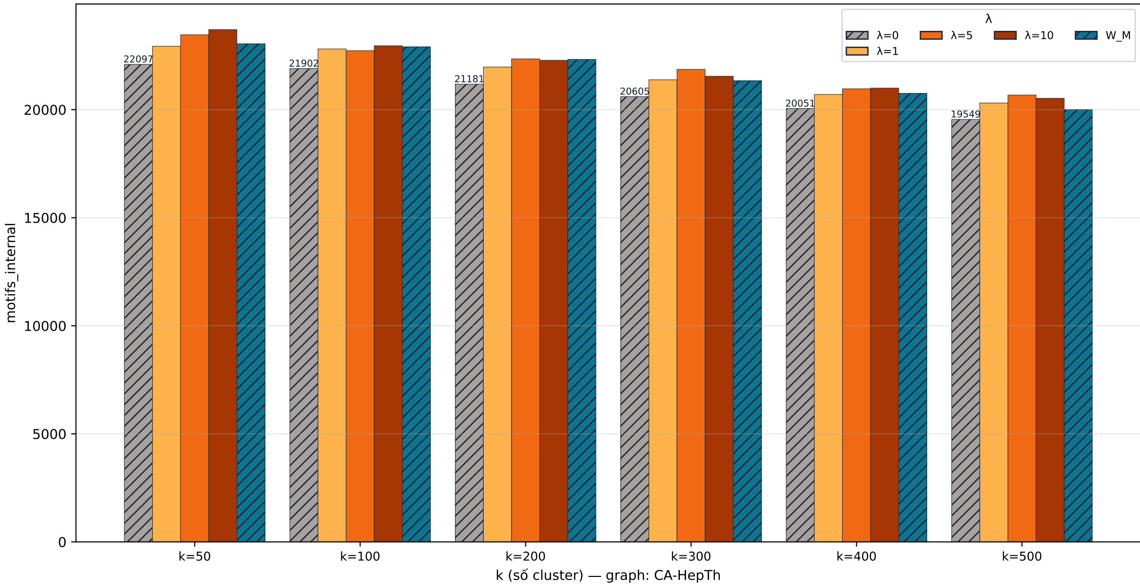
CA-HepTh cut · motifs_internal
