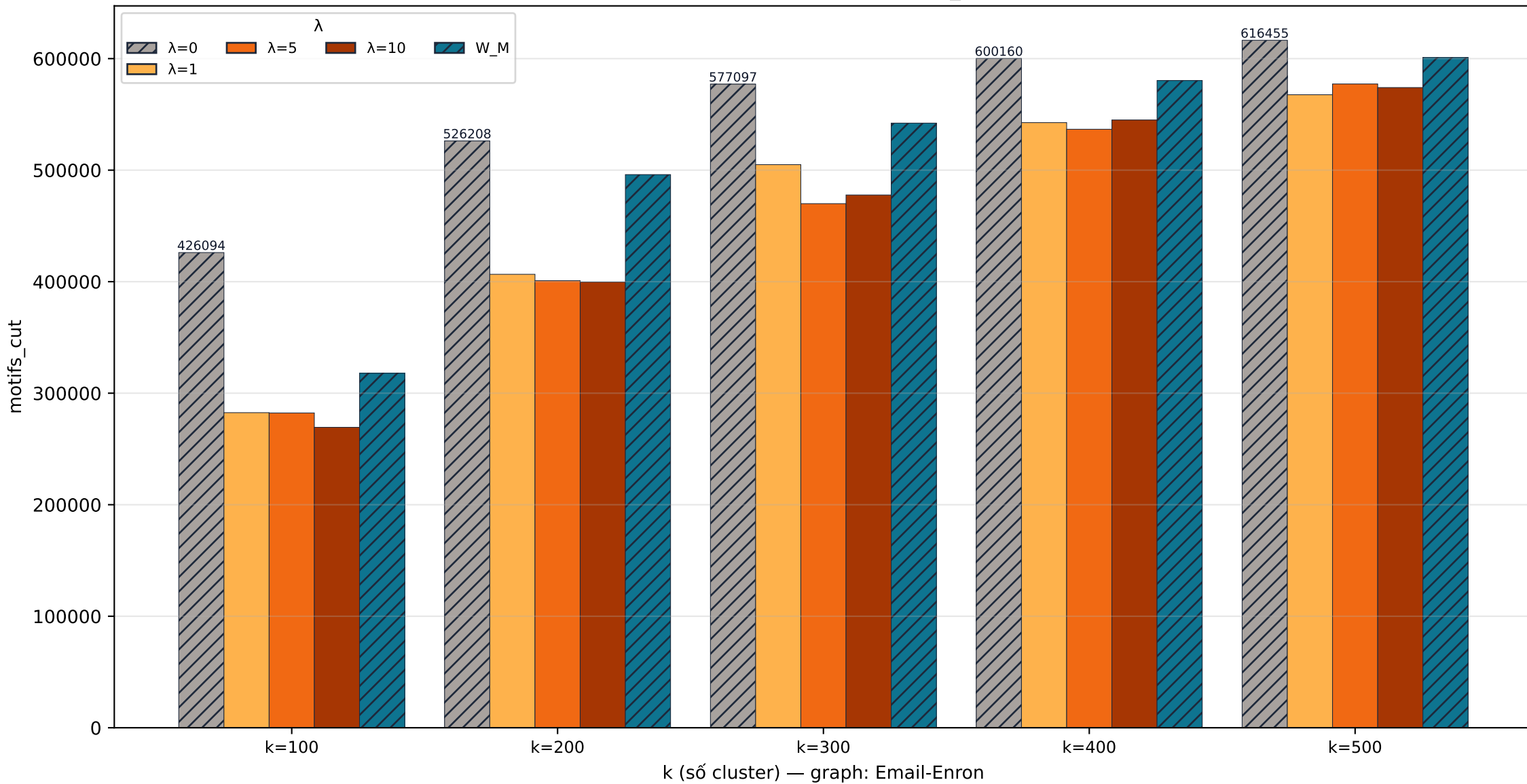
Email-Enron cut · motifs_cut
