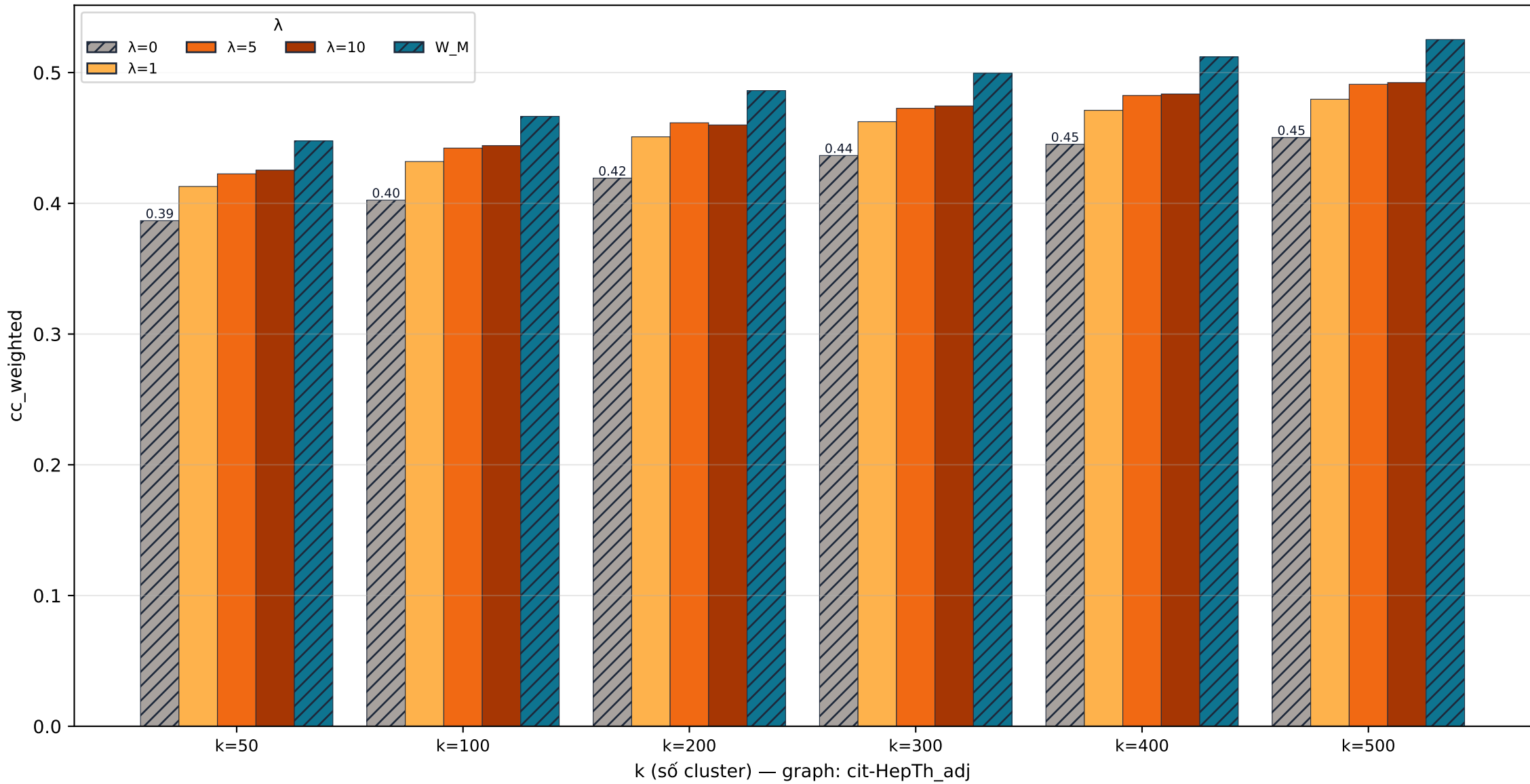
cit-HepTh_adj quality · cc_weighted
