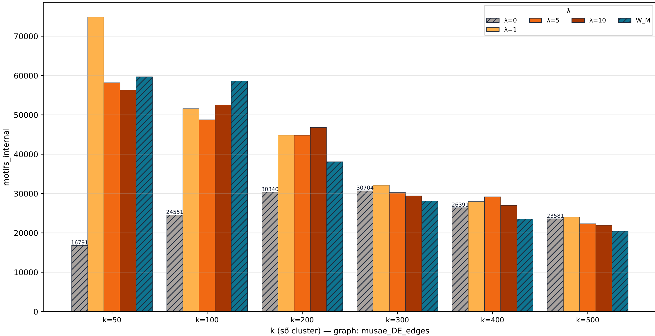
musae_DE_edges cut · motifs_internal
