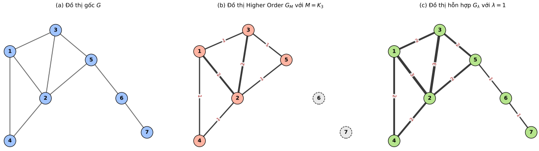
Hình 2.1: Xây dựng đồ thị hỗn hợp G_\lambda từ G và G_M với \lambda = 1 , M = K_3 .
