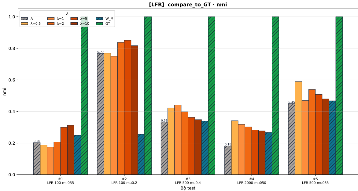
Hình 4.2: NMI so với phân hoạch chuẩn trên năm bộ LFR theo \lambda .
