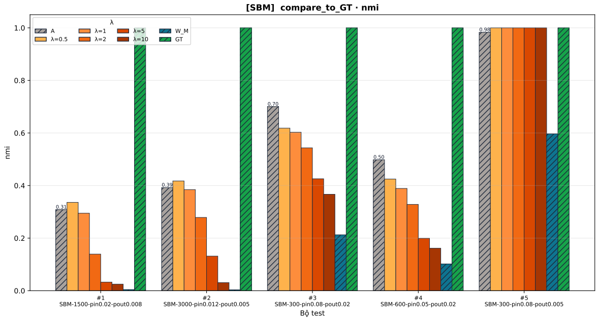
Hình 4.6: NMI so với phân hoạch chuẩn trên năm bộ SBM theo \lambda .
