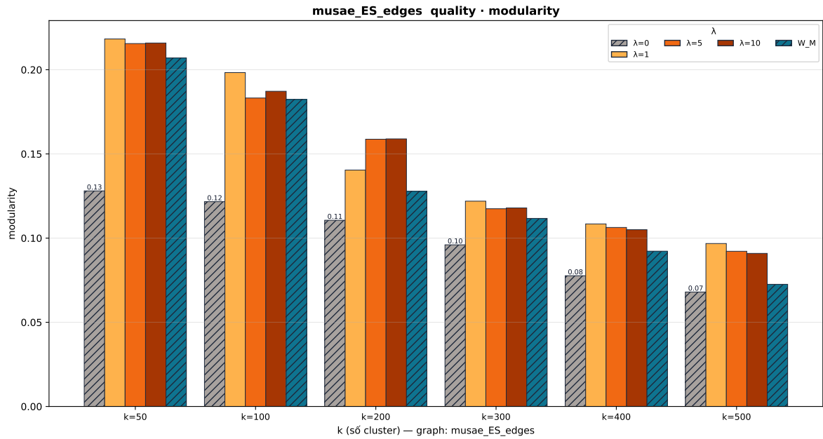
Hình 4.20: Modularity Q trên \text{musae\_ES} theo \lambda và K .
