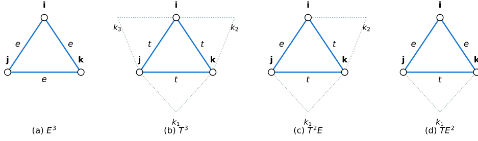
Hình 3.3: Bốn loại tam giác sinh ra trên đỉnh \{i, j, k\} qua phép chồng tăng cạnh G_E và tăng tam giác G_T : (a) E^3 ba cạnh từ G_E ; (b) T^3 ba cạnh sinh từ tam giác trong G_T với các đỉnh phụ k_1, k_2, k_3 ; (c) T^2E hai cạnh sinh từ tam giác G_T và một cạnh từ G_E ; (d) TE^2 một cạnh sinh từ tam giác G_T và hai cạnh từ G_E .
