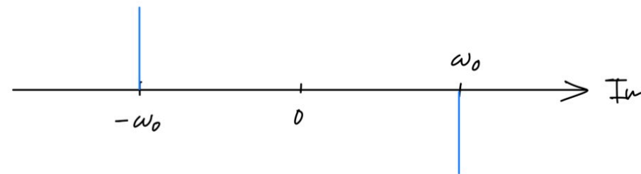
図. \sin \omega_0 t のスペクトル
