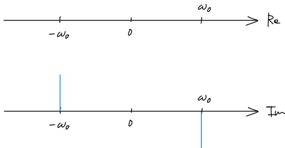
図 1. \sin \omega_0 t のスペクトル
