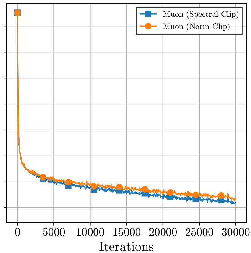
Muon
