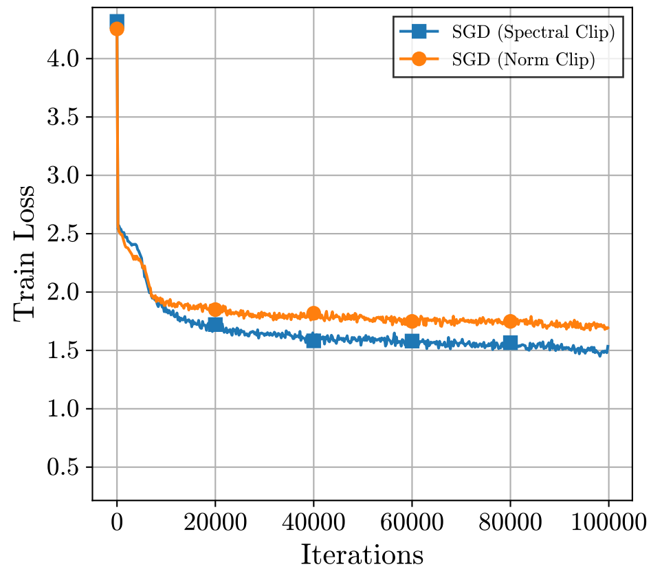
SGD
