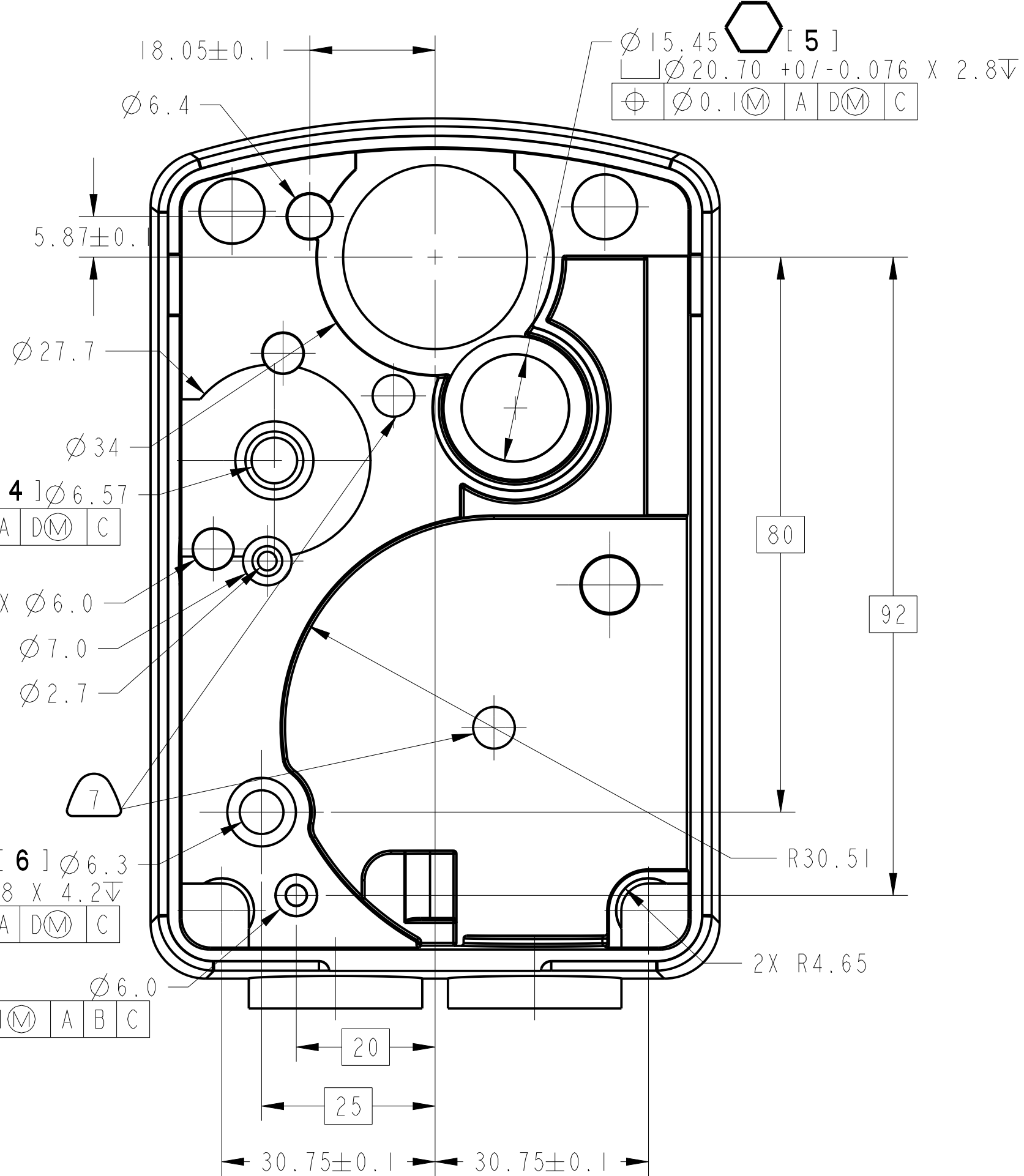
SCALE 1:1
