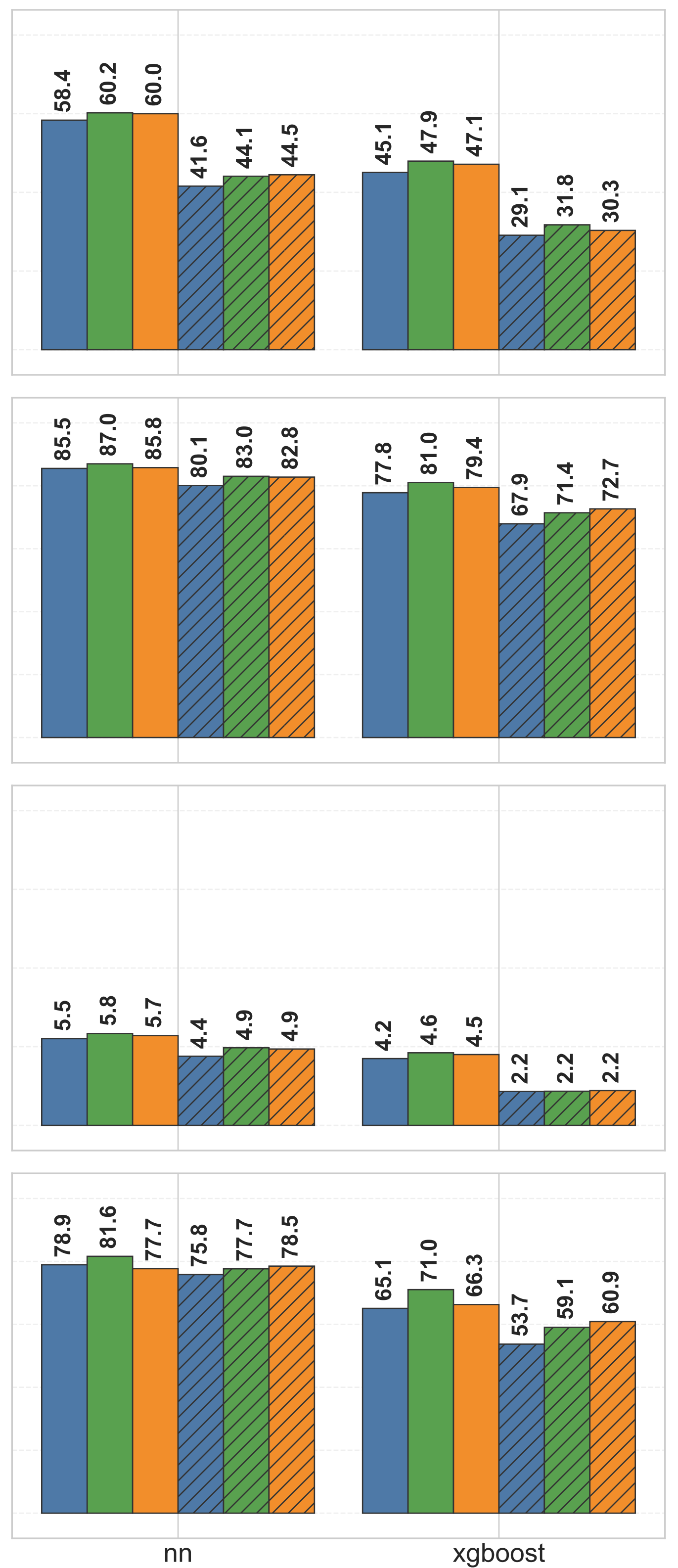
SHAP (Kernel)
