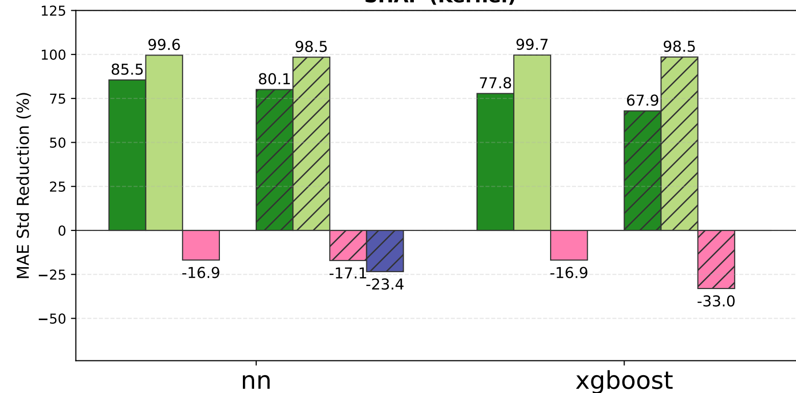
SHAP (Kernel)
