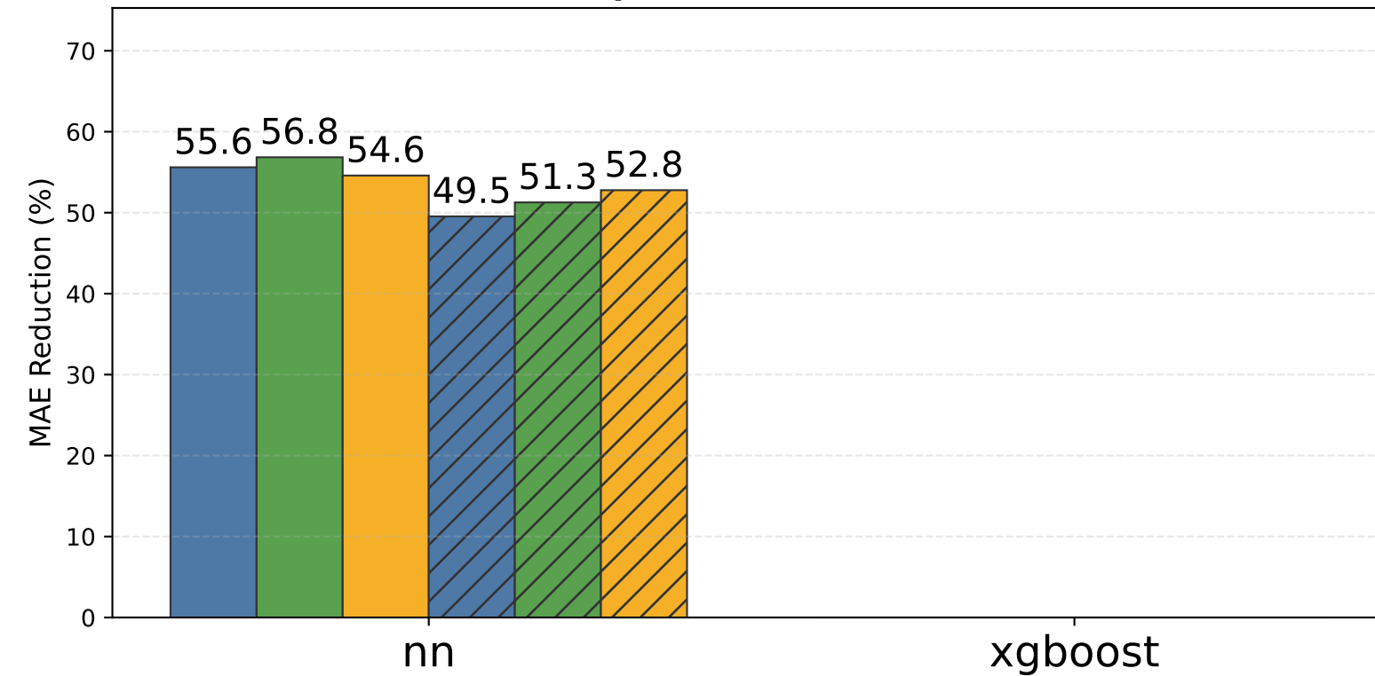
SHAP (Kernel)
