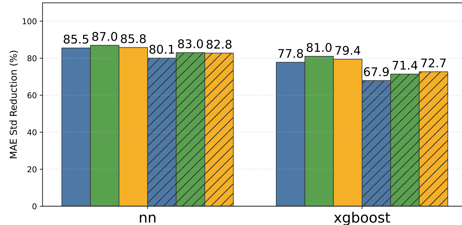
SHAP (Kernel)
