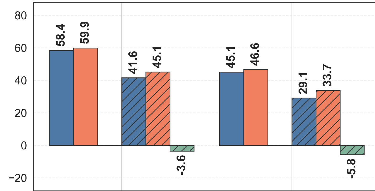
SHAP (Kernel)
