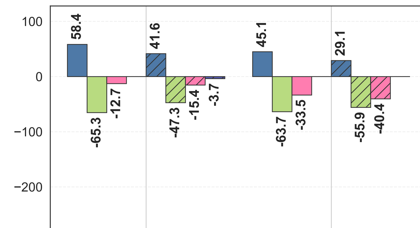
SHAP (Kernel)
