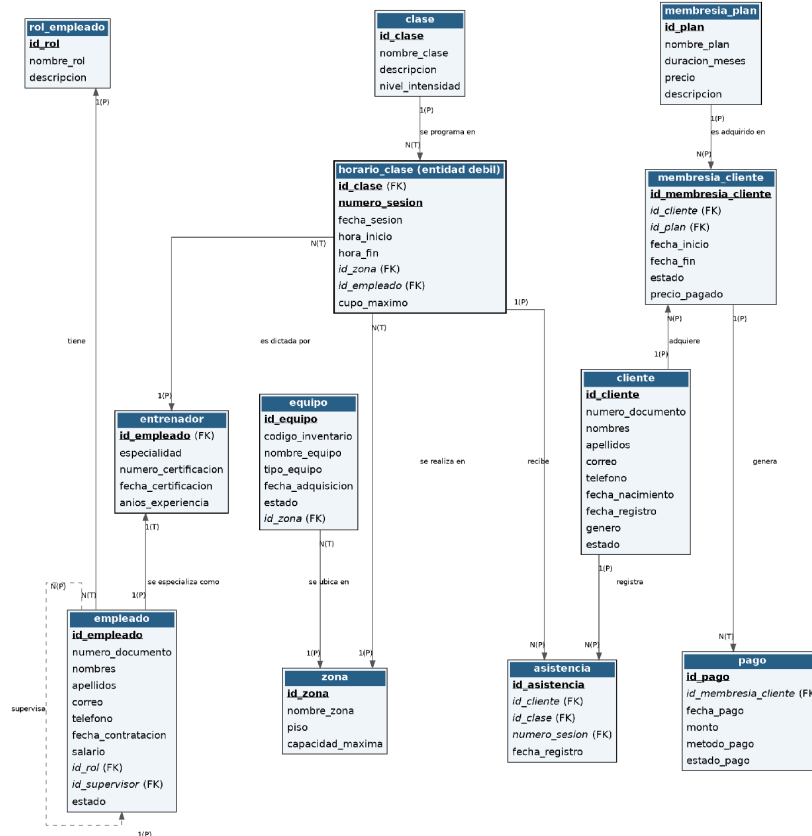
Diagrama Entidad-Relacion - GymConnect (sistema de gestion de gimnasio) Notacion: PK subrayada, FK indicada, doble borde = entidad debil, aristas con cardinalidad (1/N) y participacion (T=total, P=parcial)
