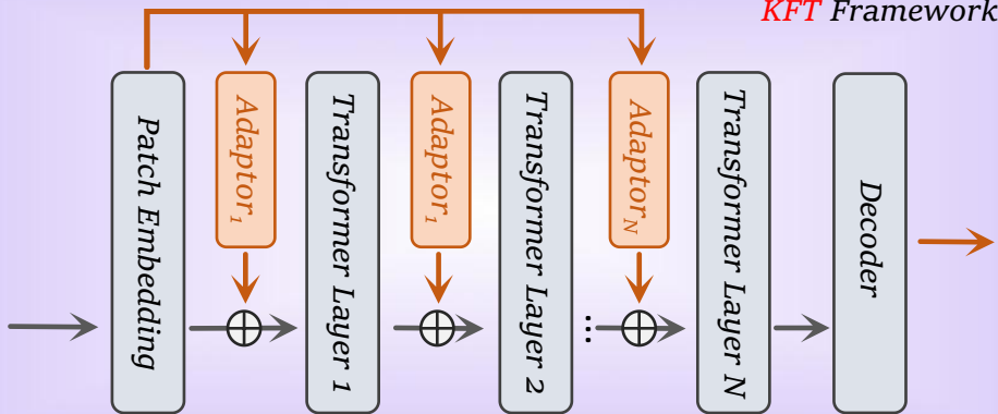
KFT Framework
