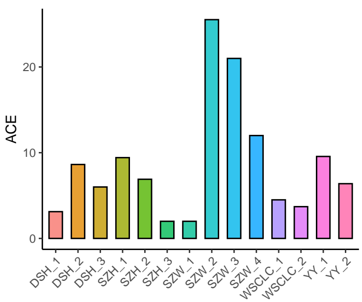
ACE Estimator
