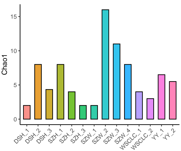
Chao1 Estimator
