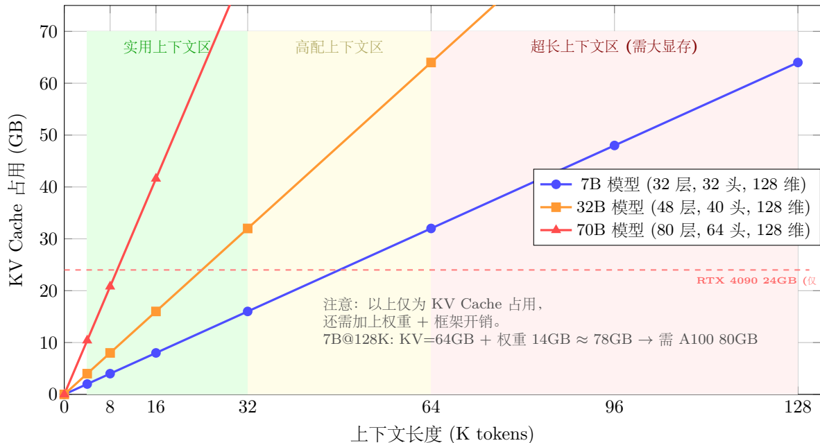
KV Cache 随上下文长度增长 (FP16 精度)
