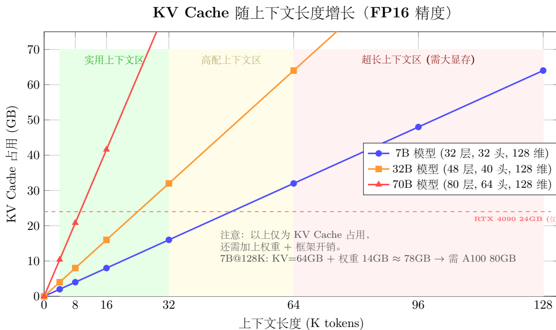
图 1: KV Cache 随上下文长度增长曲线 (FP16)。注意这仅为 KV Cache 部分，还需加上模型权重和框架开销。7B@128K 的 KV Cache 已达 64GB，足以吞没一张 RTX 4090 的全部显存。
