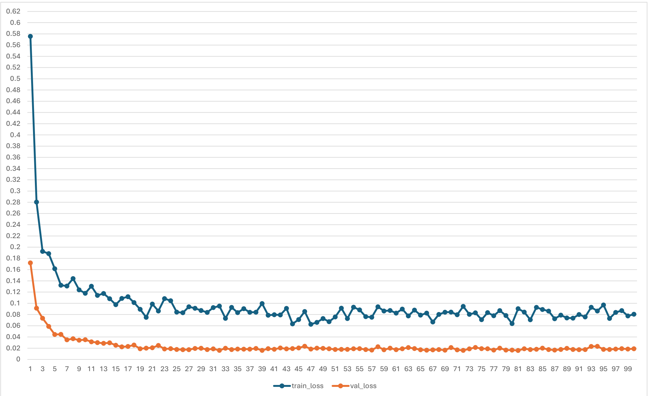
EfficientNetV2(Phase 1)
