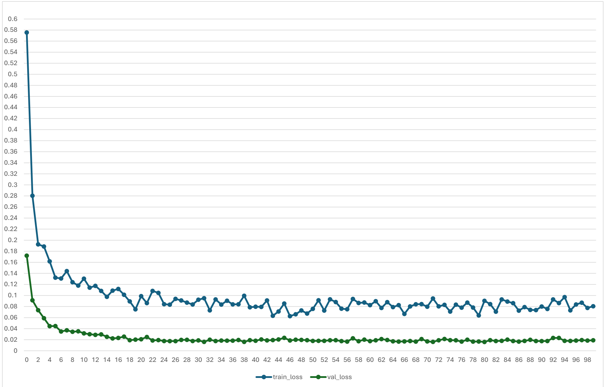
EfficientNetV2(Phase 2)
