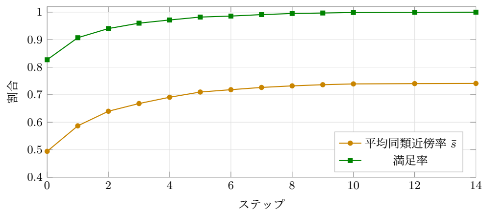
図7 基準実行の軌道 ( L = 50 , v = 0.10 , 50:50 , \tau = 0.30 , シード 42). 14 ステップで収束し, 平均同類近傍率は 0.494 から 0.741 へ上昇する.
