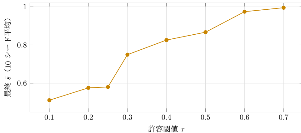
図 2 許容閾値 \tau と最終的な平均同類近傍率の関係． \tau = 0.25 \rightarrow 0.30 で不連続に跳躍する．
