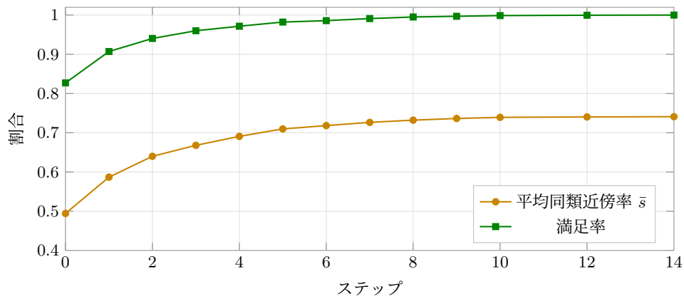
図1 基準実行の軌道 ( L = 50 , v = 0.10 , 50:50, \tau = 0.30 , シード 42). 14 ステップで収束し, 平均同類近傍率は 0.494 から 0.741 へ上昇する.
