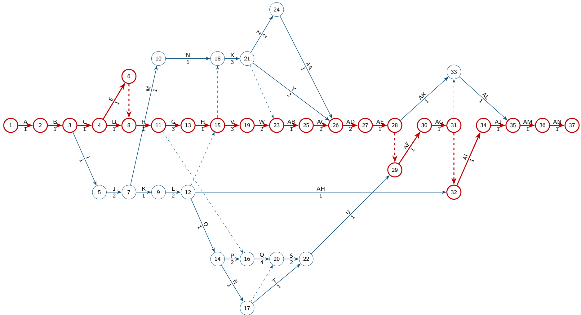
FIGURA I: REDE DE ATIVIDADES DO TIPO AOA. EM VERMELHO, O CAMINHO CRÍTICO; TRACEJADAS, AS ATIVIDADES FANTASMA.
