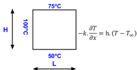
Figure 1: Configuração da placa metálica
