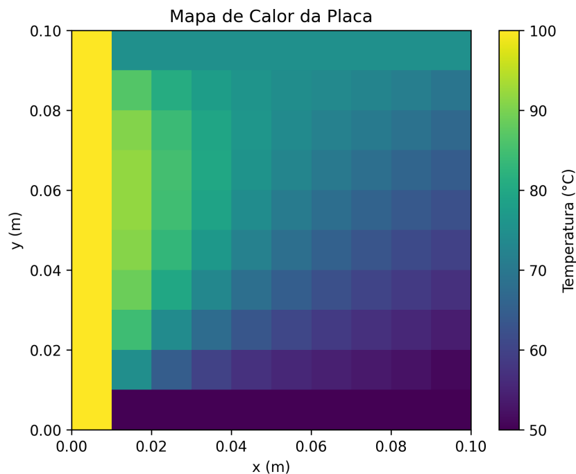
Figure 2: Mapa de calor da distribuição de temperatura na placa
