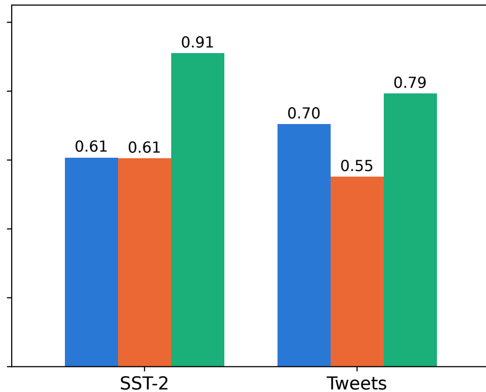
Macro-F1
