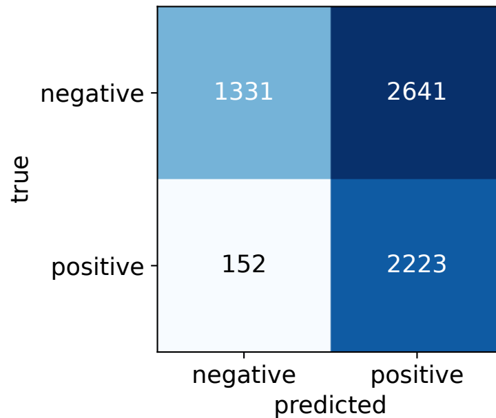
Tweets: TextBlob
