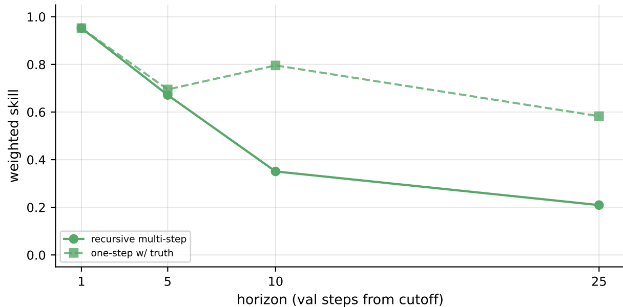
most stable: GRU/target_only
