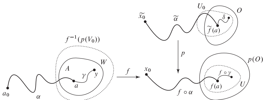
Figura 9.4: Continuidad del levantamiento \tilde{f} .
