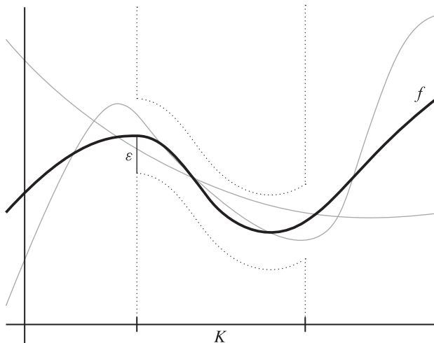
Figura 11.3: El conjunto B(K, f, \varepsilon) .
