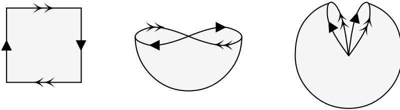
Figura 4.5: Identificación e imagen de un Plano Proyectivo.
