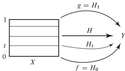
Figura 8.1: Homotopía entre f y g .
