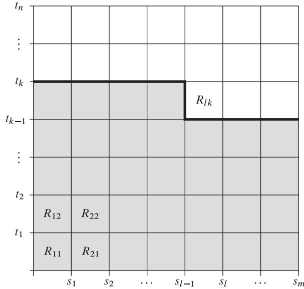
Figura 8.13: Partición de I \times I .
