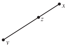
Figura 1.1: Interpretación geométrica del punto z entre los puntos x y y .
