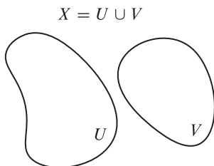
Figura 7.1: (U, V) desconexión de X .
