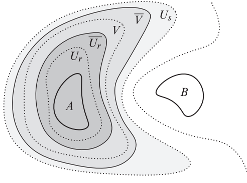
Figura 5.7: Las vecindades U_r
