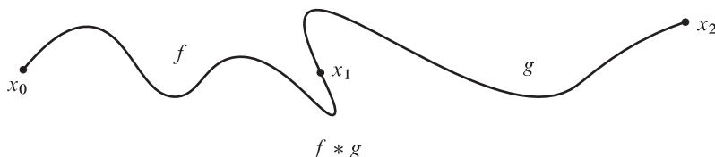
Figura 8.4: Producto de trayectorias.
