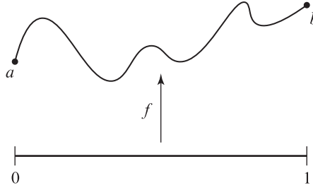
Figura 7.3: Trayectoria entre a y b .
