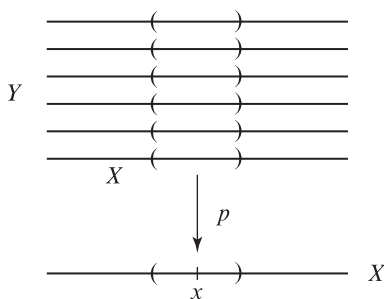
Figura 9.2: Vecindad admisible del punto x en X .
