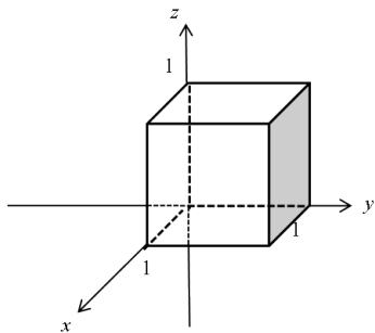
Figura 1.12: \mathbb{I}^3 , cubo unitario de \mathbb{R}^3 .
