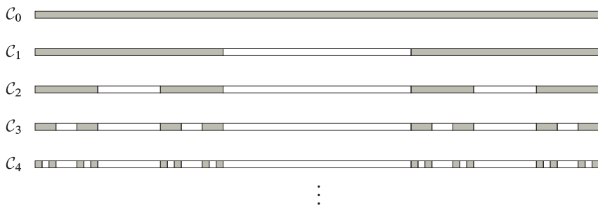
Figura 6.1: Cinco iteraciones de la construcción del conjunto de Cantor.
