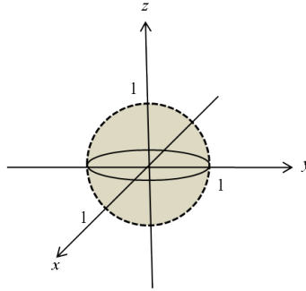
Figura 1.10: \mathbb{B}^3 , bola unitaria de \mathbb{R}^3 .
