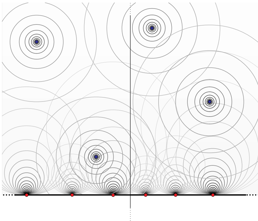
Figura 2.6: El Plano de Niemytzki
