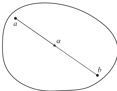
Figura 7.4: El convexo K es conexo por trayectorias.
