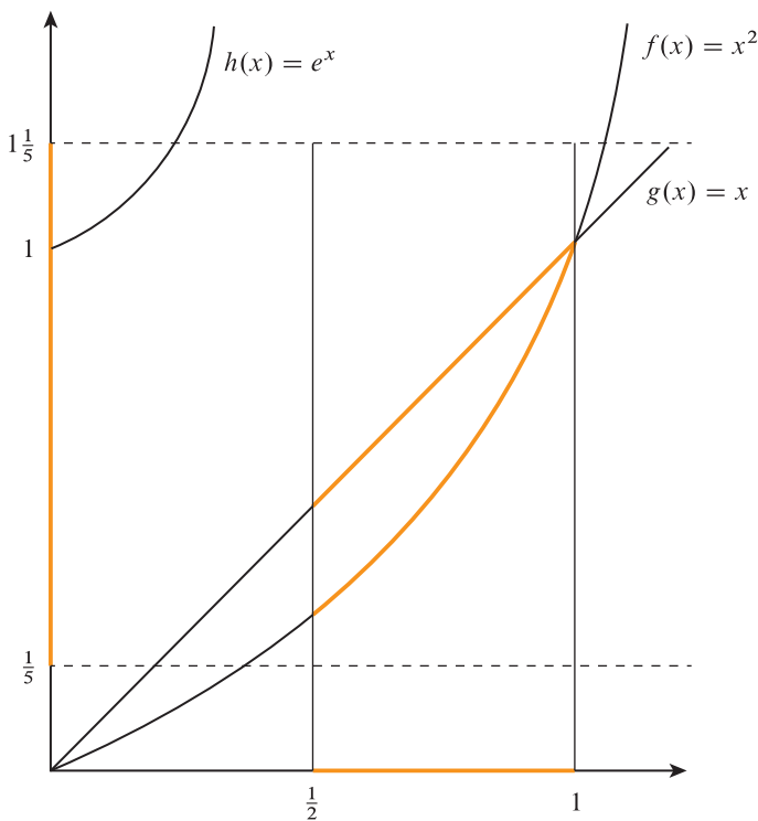
Figura 11.2: Las funciones f y g pertenecen a M(K, W) , mientras que h no.
