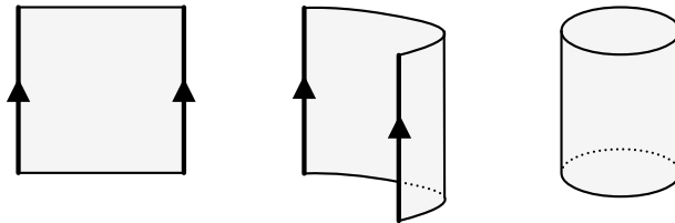
Figura 4.1: Identificación e imagen de un cilindro.
