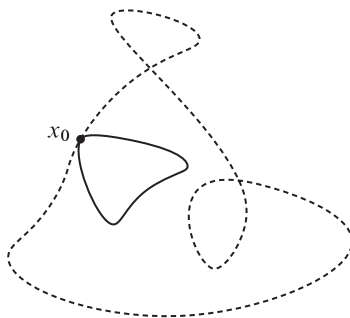
Figura 8.10: Lazos basados en x_0 .
