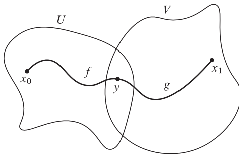
Figura 8.16: X conexo por trayectorias.
