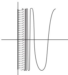
Figura 7.5: Seno del topólogo.
