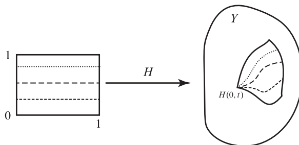
Figura 8.2: Homotopía relativa a A = \{0\} .
