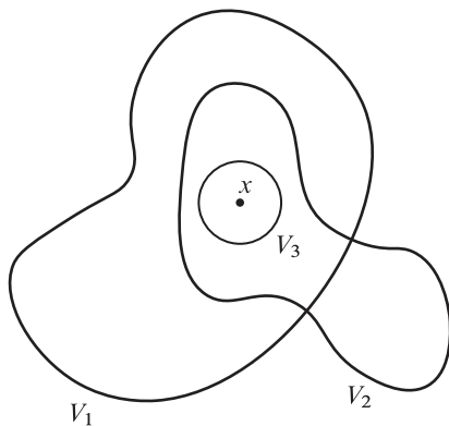
Figura 2.1: Propiedades de una base
