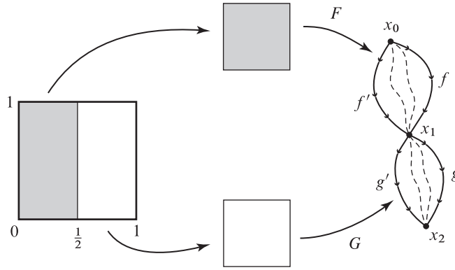
Figura 8.5: Homotopía de productos.
