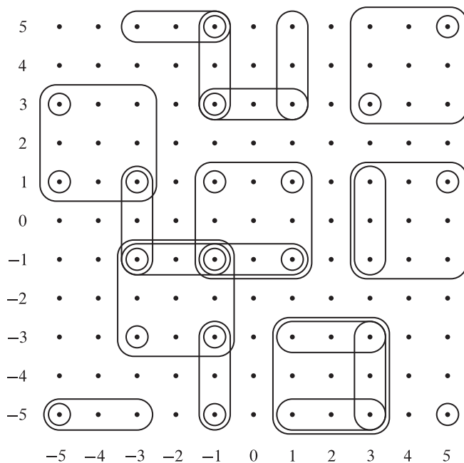
Figura 2.3: El Plano Digital
