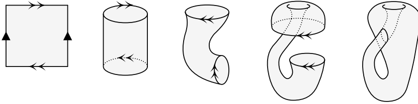
Figura 4.4: Identificación e imagen de una Botella de Klein.
