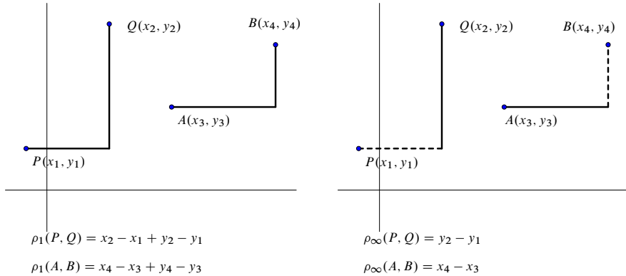
Figura 1.2: Métricas \rho_1 y \rho_\infty
