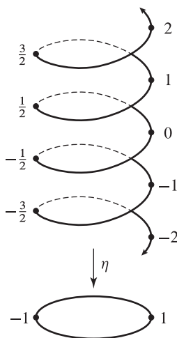
Figura 8.12: Función cubriente de \mathbb{S}^1 .
