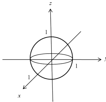
Figura 1.11: \mathbb{S}^2 , esfera unitaria de \mathbb{R}^3 .
