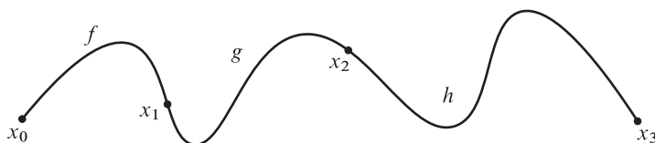
Figura 8.7: Producto de trayectorias asociativo (salvo homotopía).
