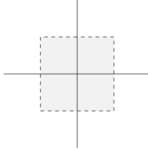
Figura 1.8: Bola abierta con la métrica del supremo de \mathbb{R}^2 .
