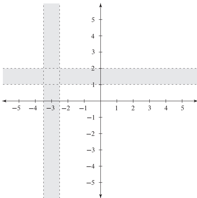
Figura 2.4: Una subbase para \mathbb{R}^2
