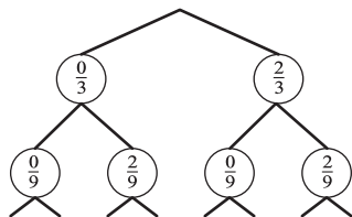
Figura 6.2: Representación diagramal del conjunto de Cantor y de los números binarios.
