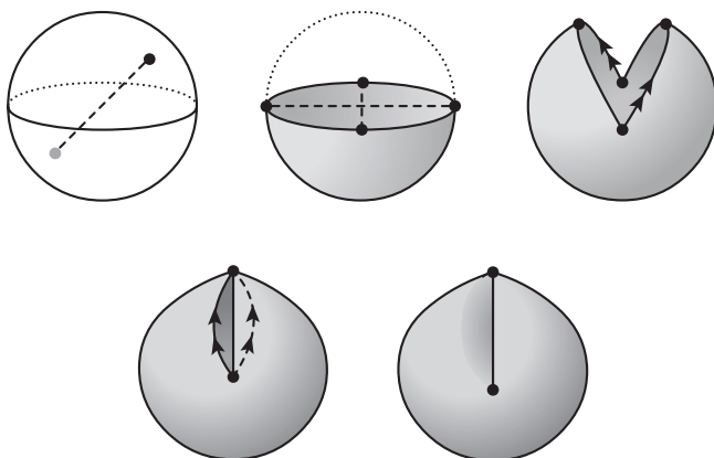
Figura 4.6: Identificación e imagen de un Plano Projectivo.
