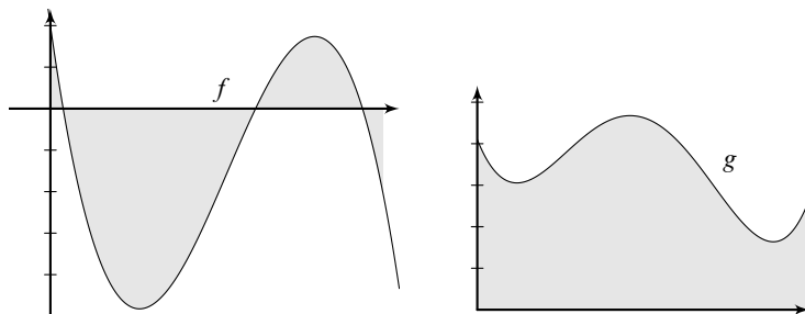
Figura 1.3: Significado geométrico de \|\cdot\|_1 : área de la región sombreada.
