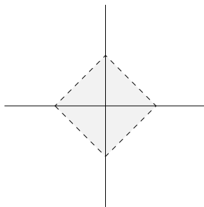
Figura 1.7: Bola abierta con la métrica del taxista de \mathbb{R}^2 .
