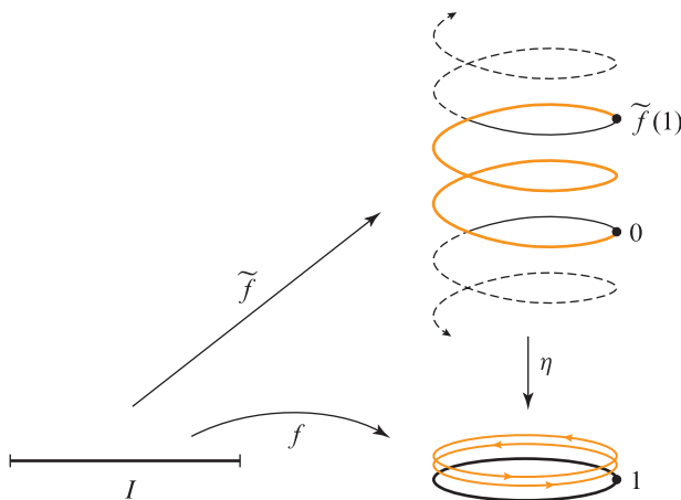
Figura 8.14: Levantamiento de f: I \rightarrow \mathbb{S}^1 .
