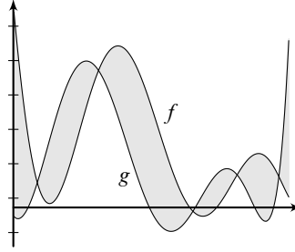
Figura 1.4: El significado geométrico de la métrica \rho_1 : \rho_1(f, g) es el área de la región sombreada.
