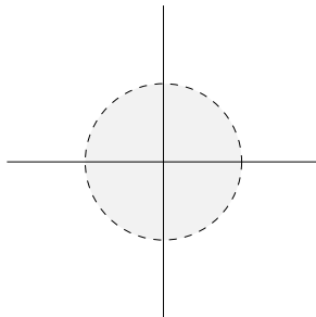
Figura 1.6: Bola abierta con la métrica usual de \mathbb{R}^2 .
