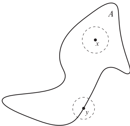
Figura 1.9: Conjunto A con un punto interior x y un punto que no es interior y .
