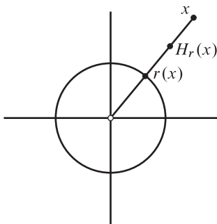
Figura 8.3: Equivalencia homotópica entre \mathbb{R}^n \setminus \{0\} y \mathbb{S}^{n-1} .
