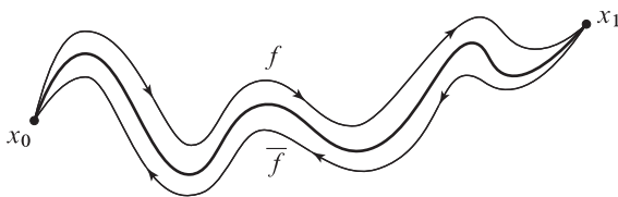
Figura 8.9: f y \bar{f} .
