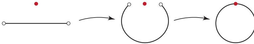
Figura 6.3: Compactación de Alexandroff de (0, 1)
