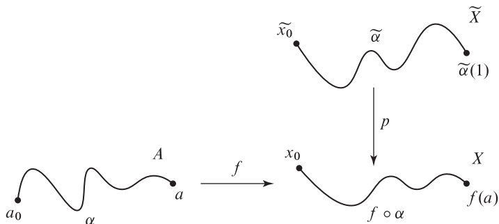
Figura 9.3: Construcción del levantamiento \tilde{f} .
