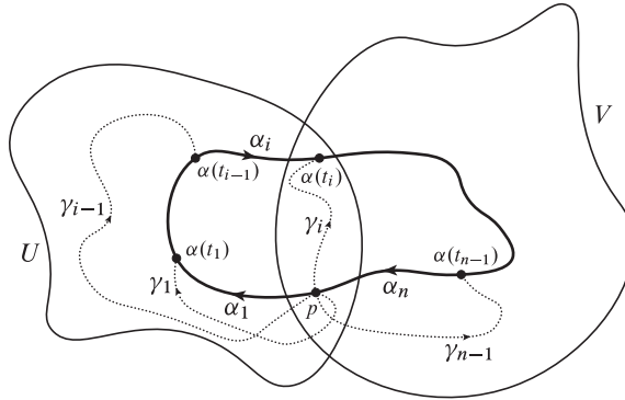
Figura 8.17: La trivialidad de \alpha .
