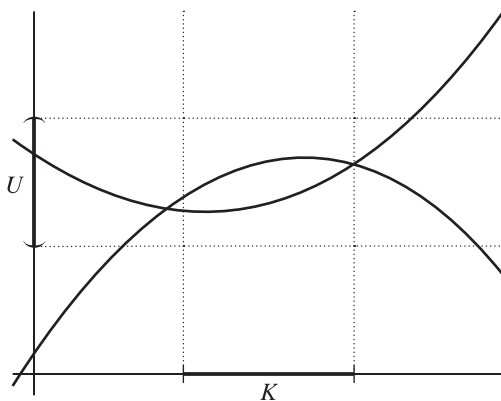
Figura 11.1: Dos funciones del conjunto M(K, U) .
