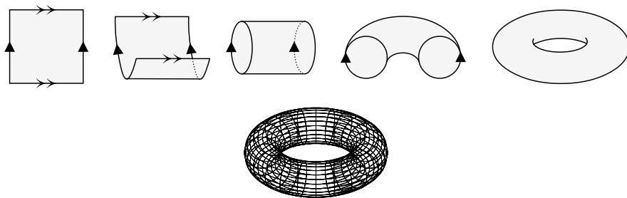
Figura 4.3: Identificación e imagen de un Toro.
