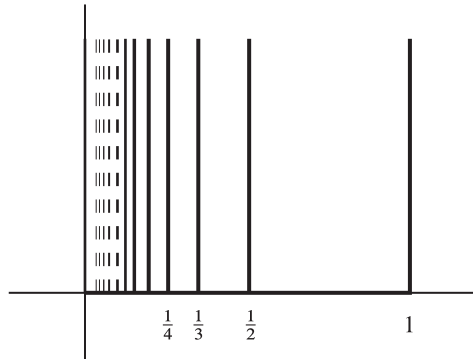
Figura 7.6: Peine del topólogo.
