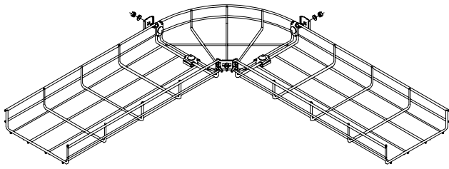
90° bend
