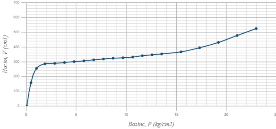
DÜZELTİLMİŞ PRESİYOMETRE EĞRİSİ / Corrected Pressuremeter Curve
