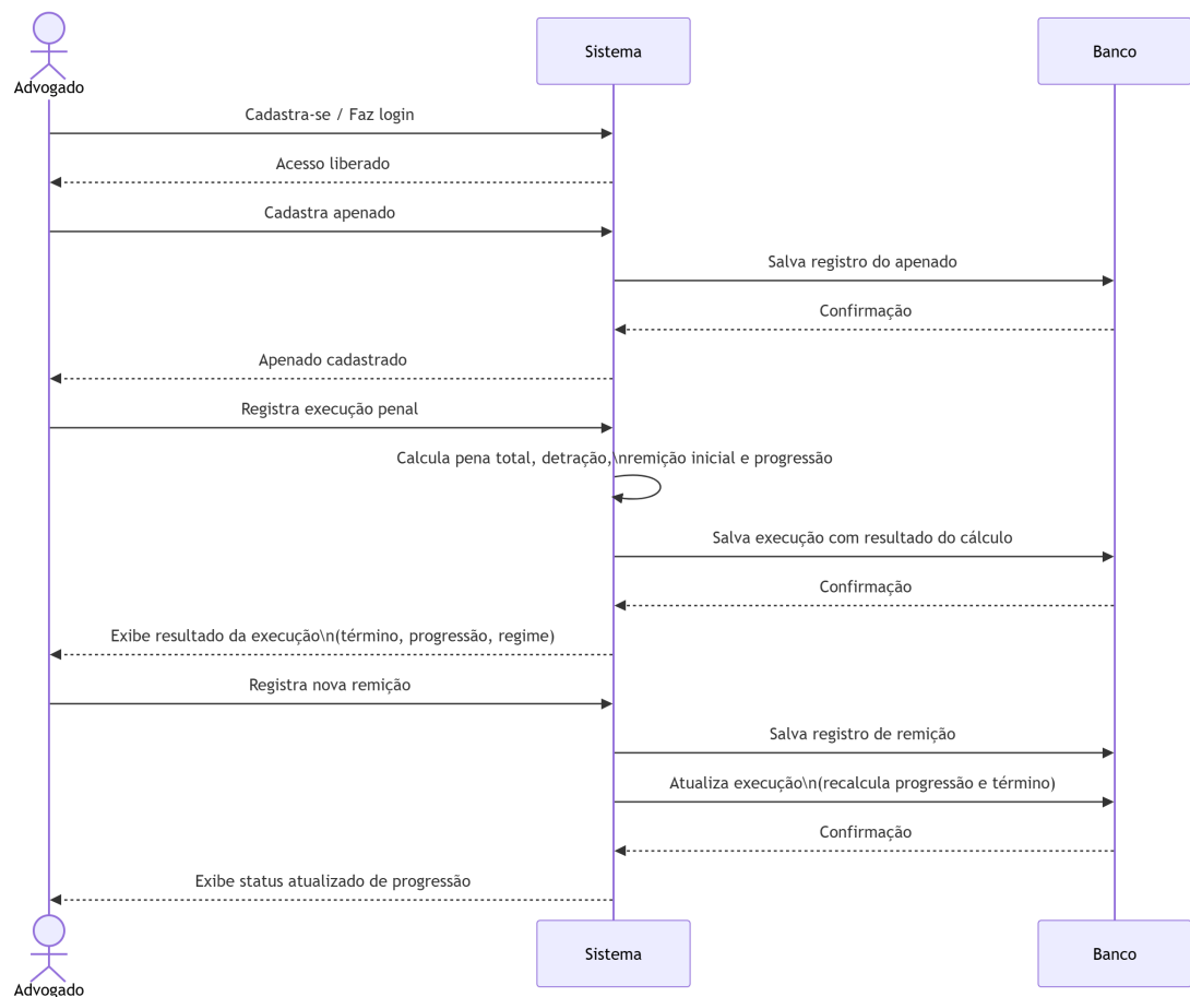
Figura 3 – Diagrama de Sequência.
