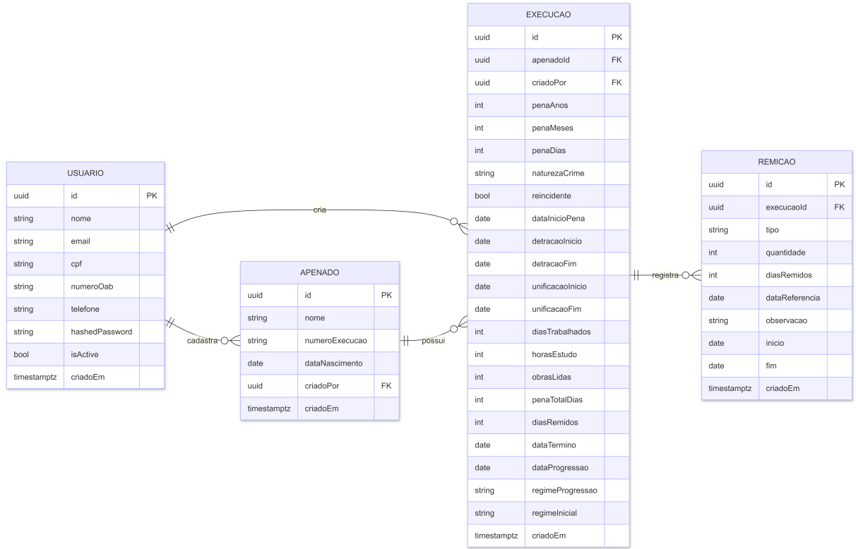
Figura 4 – Diagrama Entidade-Relacionamento.
