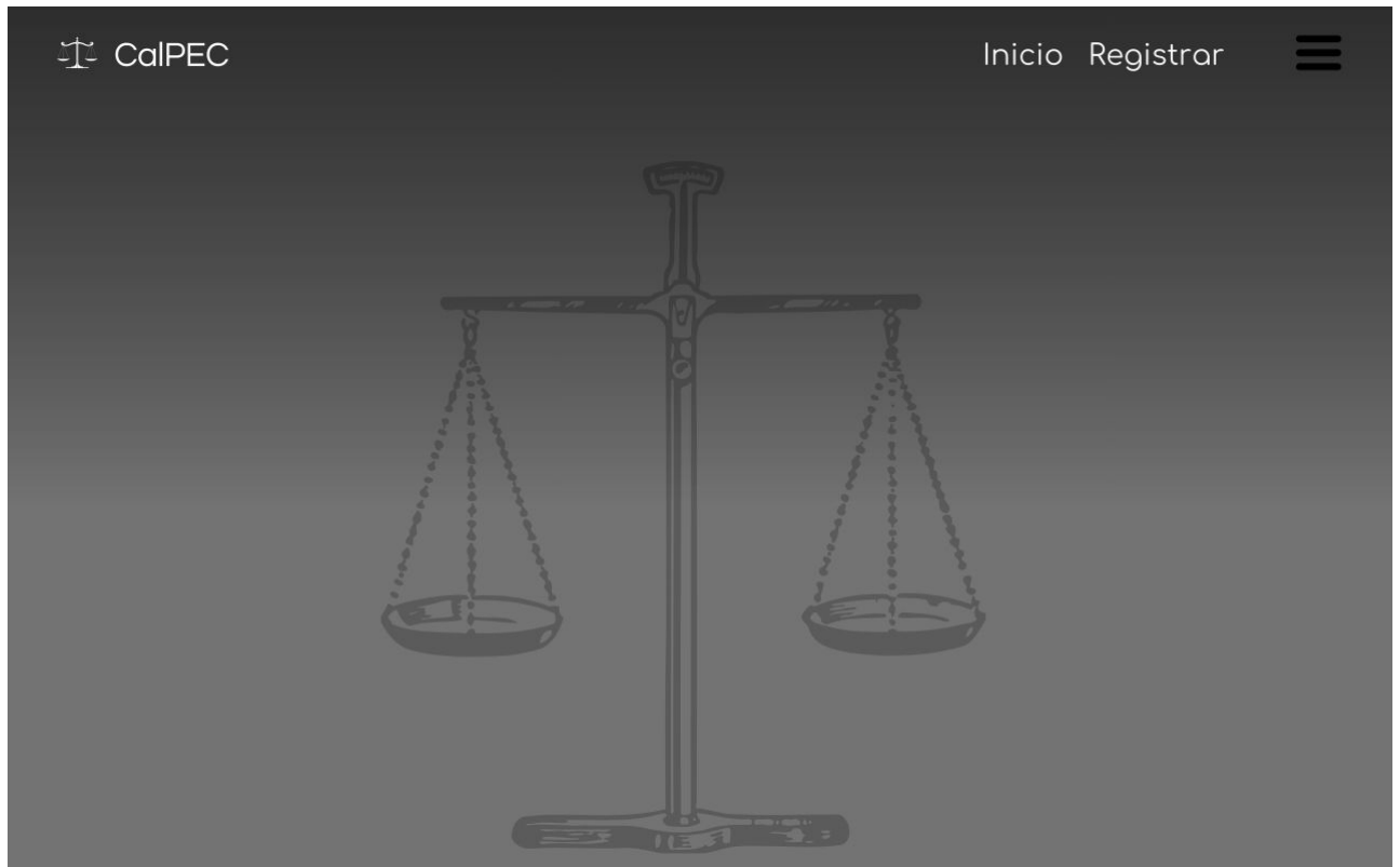
Figura 2 – Tela Inicial.
