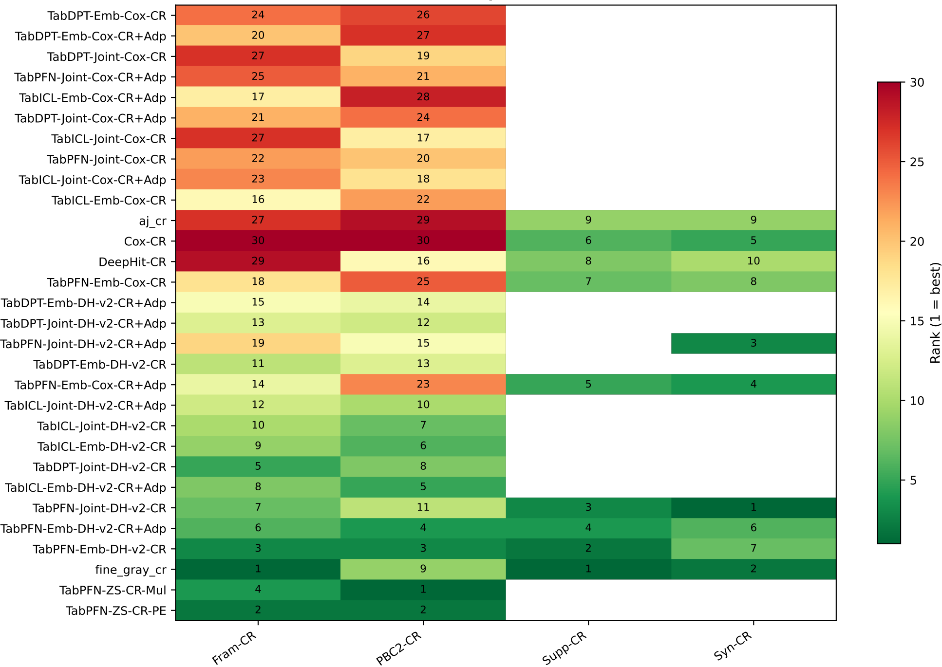
Model Rank per Dataset (CR)
