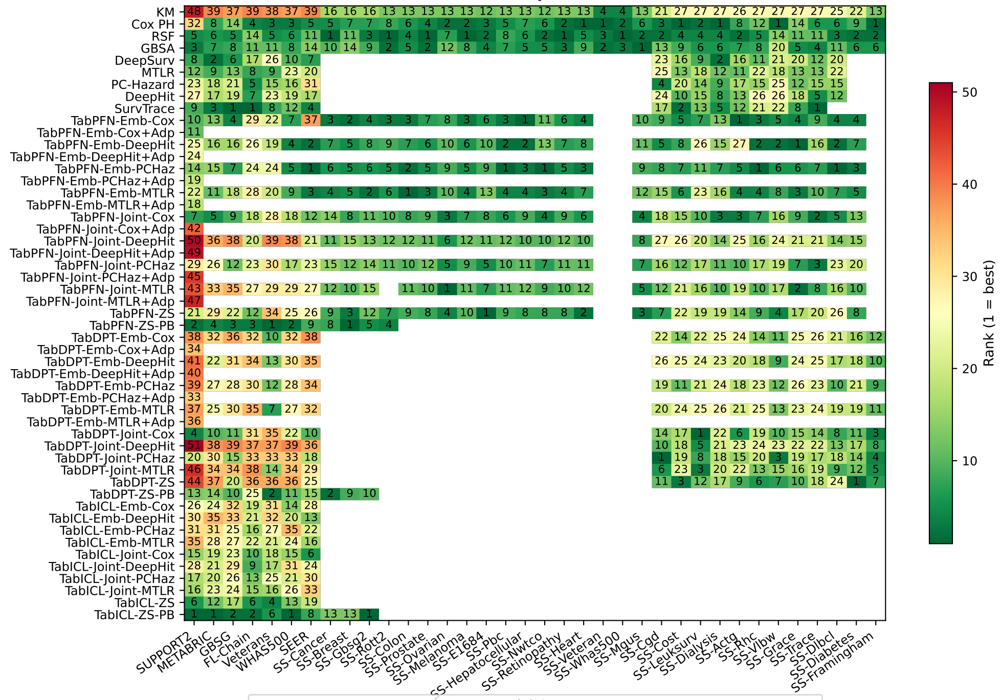
Model Rank per Dataset
