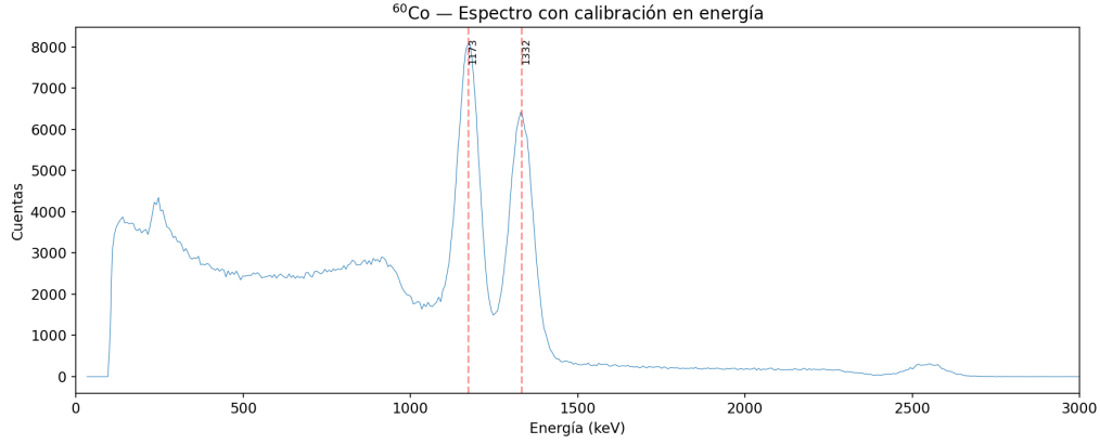
Figura 10: Espectro de ^{60}\text{Co} calibrado en energ a. Las l neas rojas se alan las posiciones esperadas de 1173.2 keV y 1332.5 keV.
