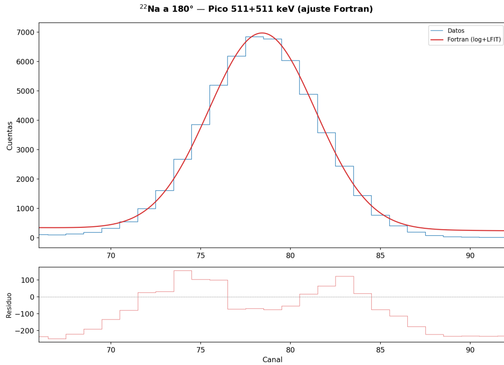
Figura 5: Ajuste gaussiano del pico de 511 keV (511+511) en ^{22}\text{Na} a 180^\circ .
