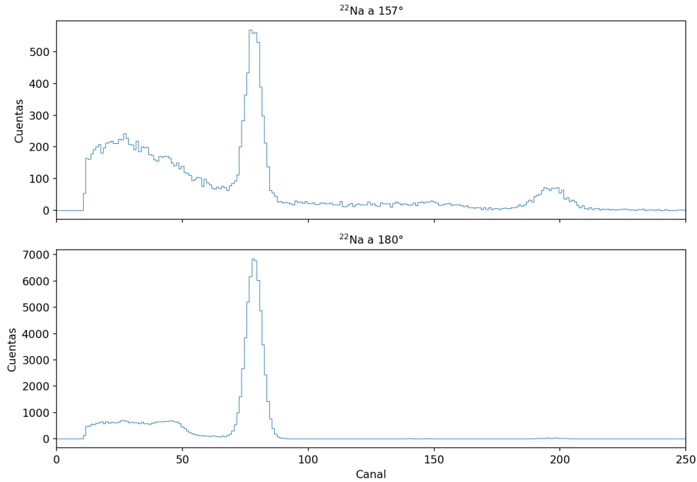
Figura 6: Comparación de los espectros de ^{22}\text{Na} a 157° y 180°.
