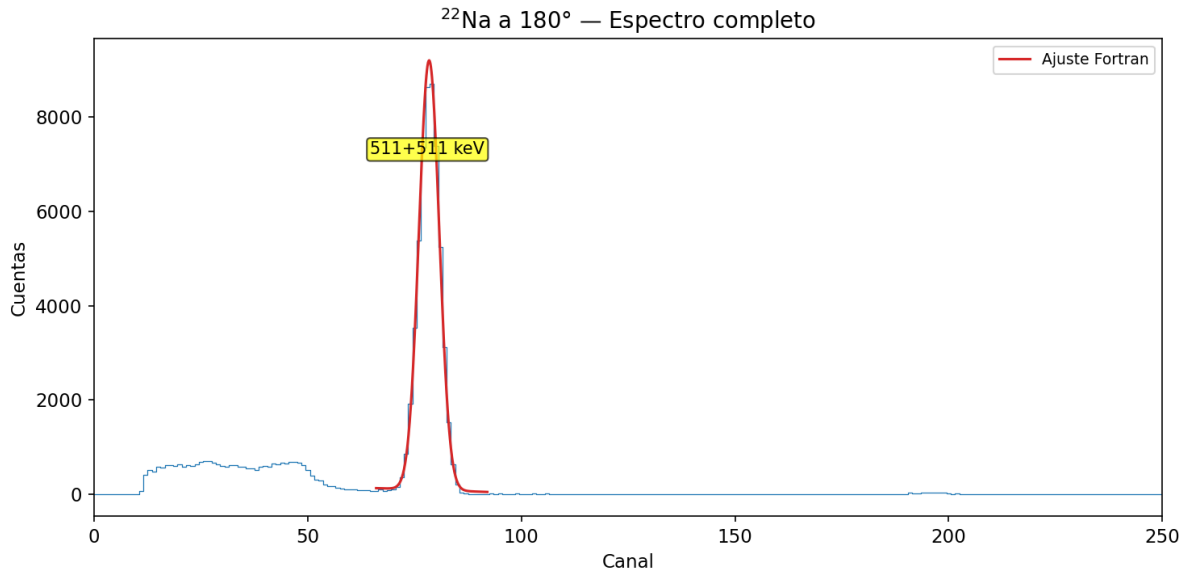
Figura 4: Espectro completo de coincidencias de ^{22}\text{Na} a 180°.
