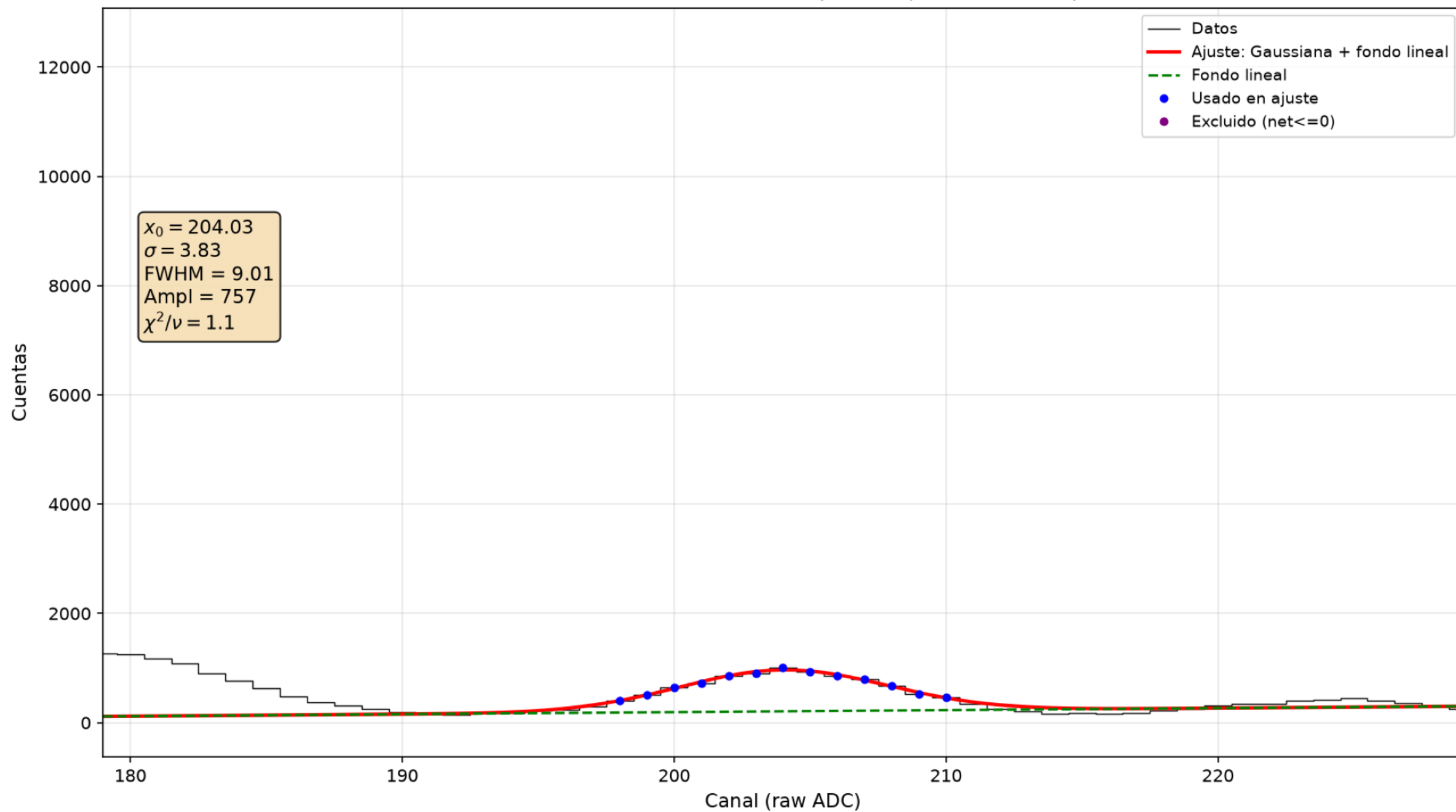
60-Co-90-coin — Pico 1332 keV (MCAch1, detector móvil)
