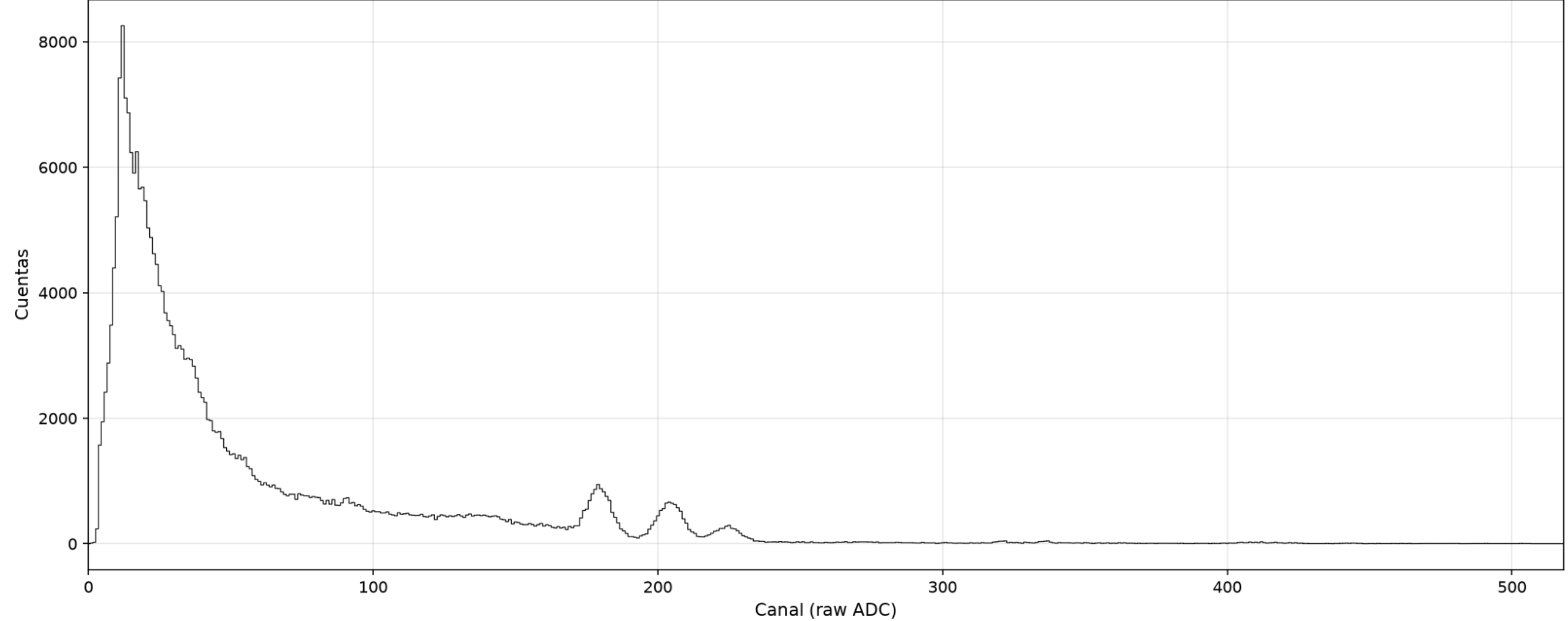
60-Co-67,5-coin — MCAch1 (detector móvil)
