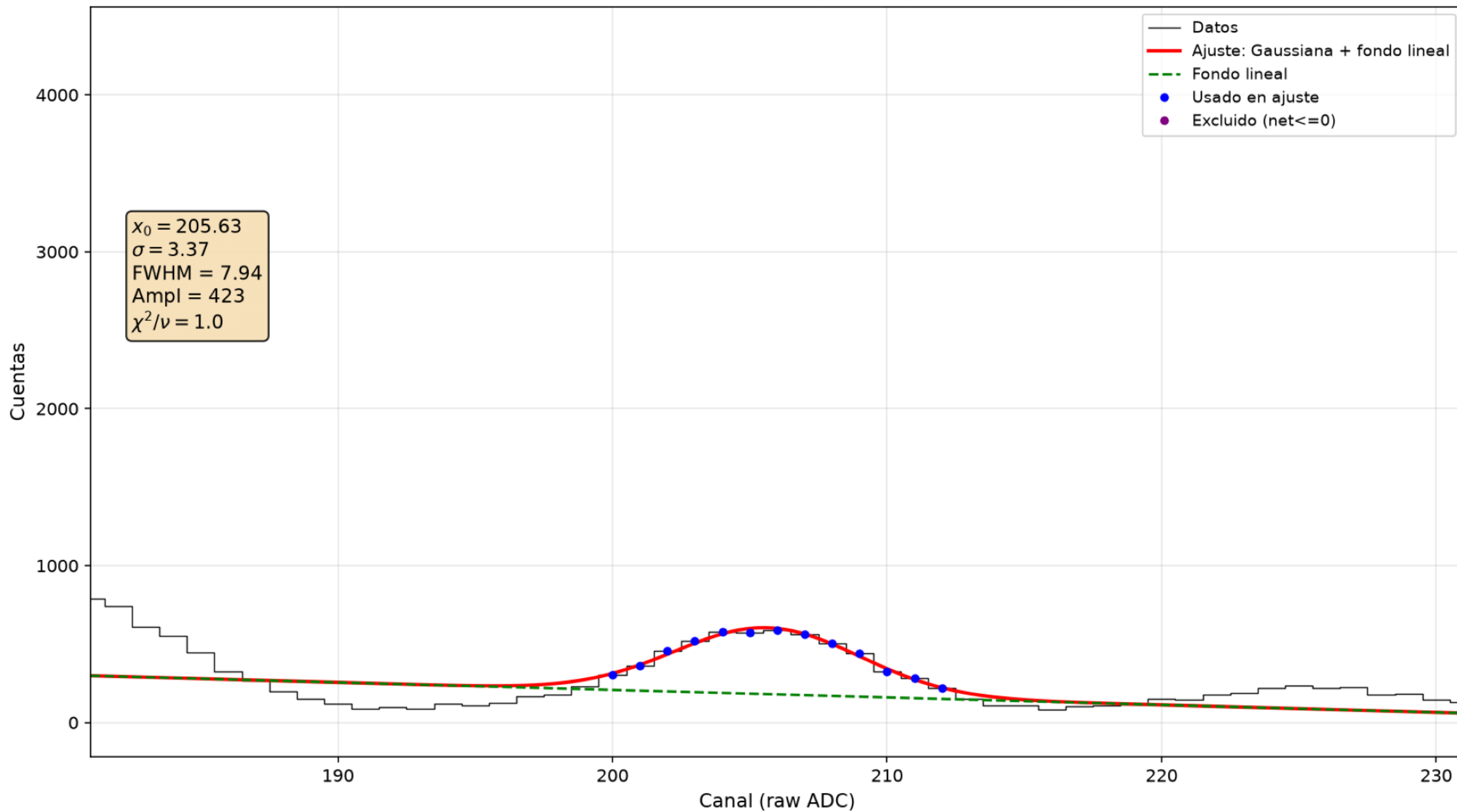
60Co-180-coin — Pico 1332 keV (MCAch1, detector móvil)
