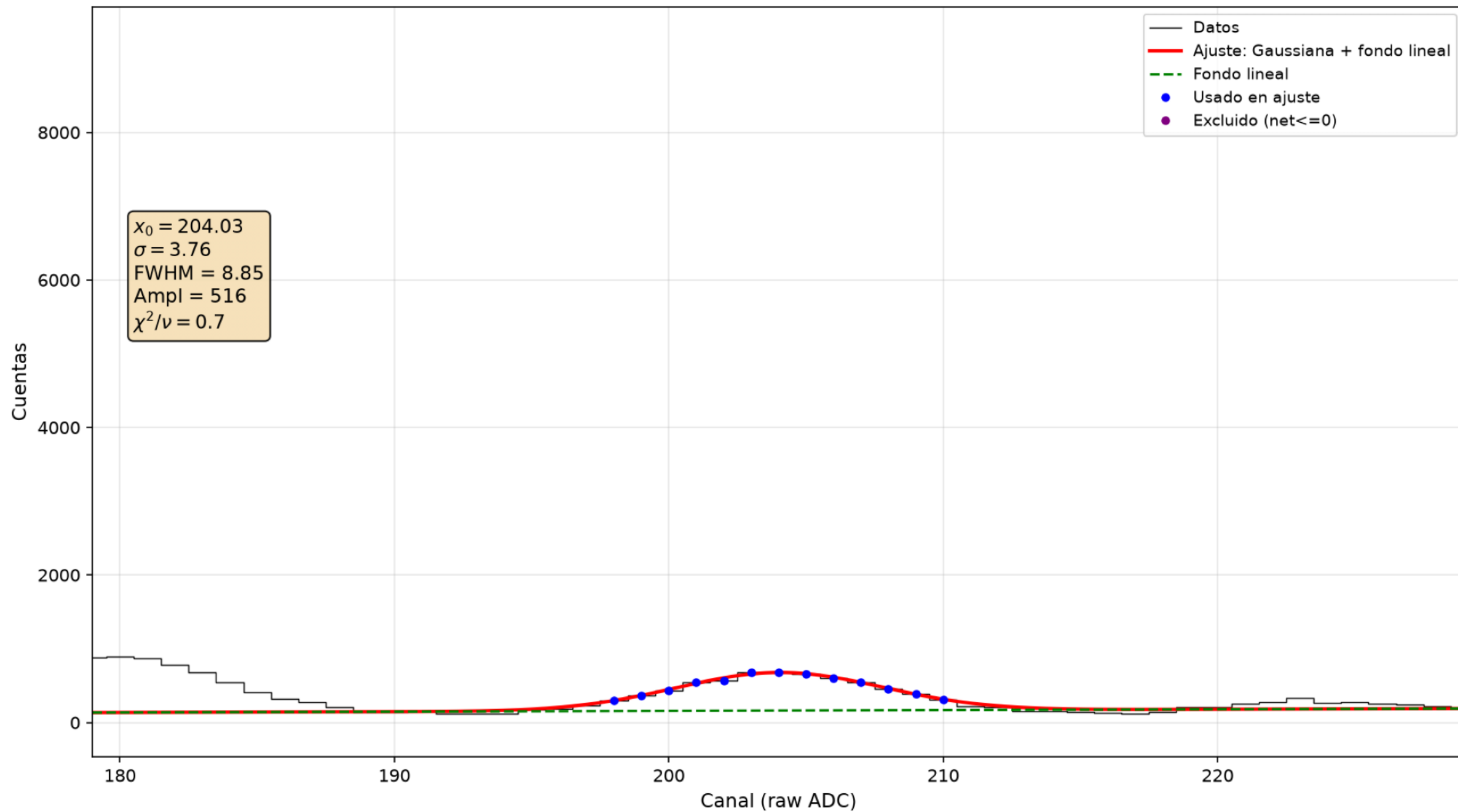
60-Co-135-coin — Pico 1332 keV (MCAch1, detector móvil)
