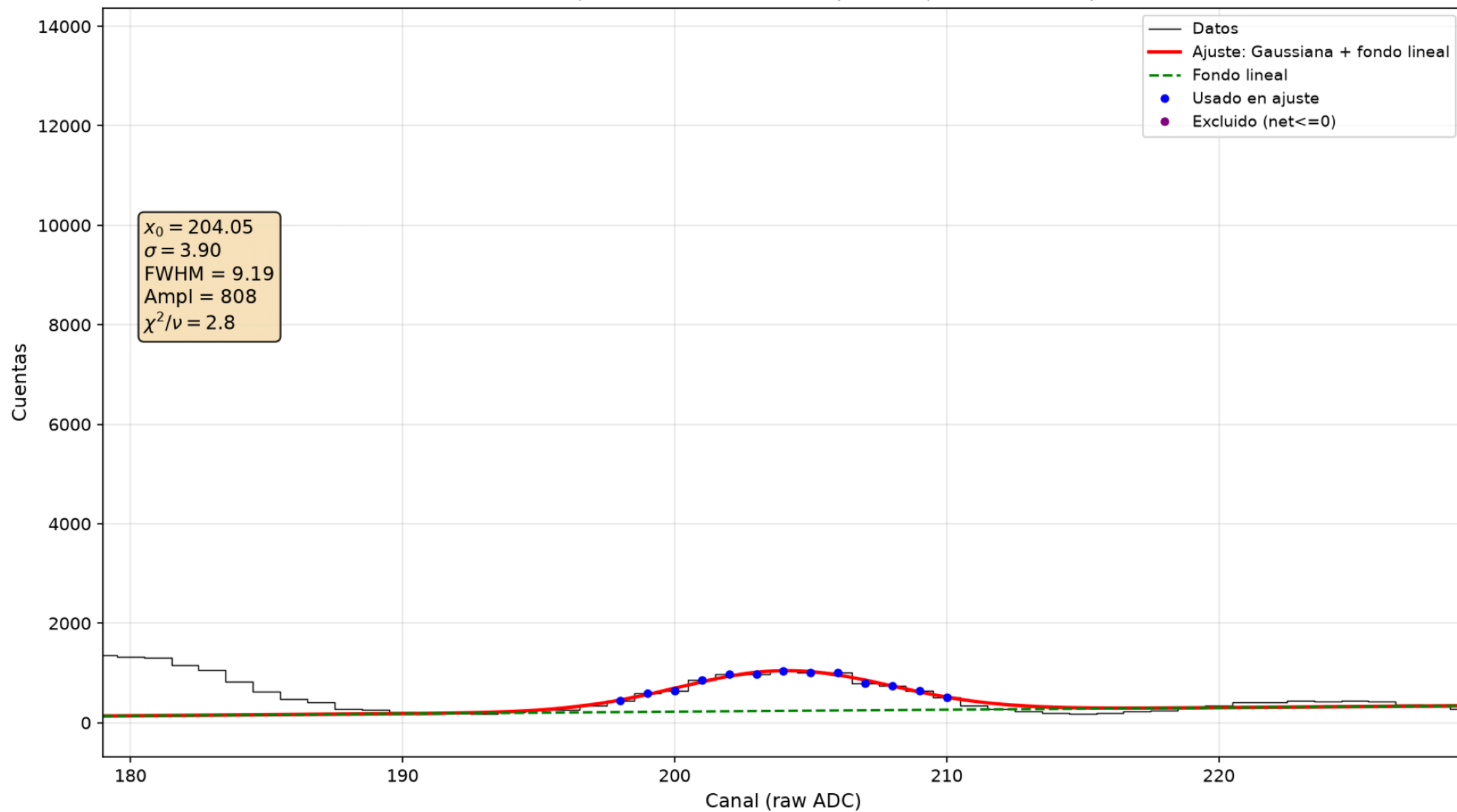
60-Co-157,5-coin — Pico 1332 keV (MCAch1, detector móvil)
