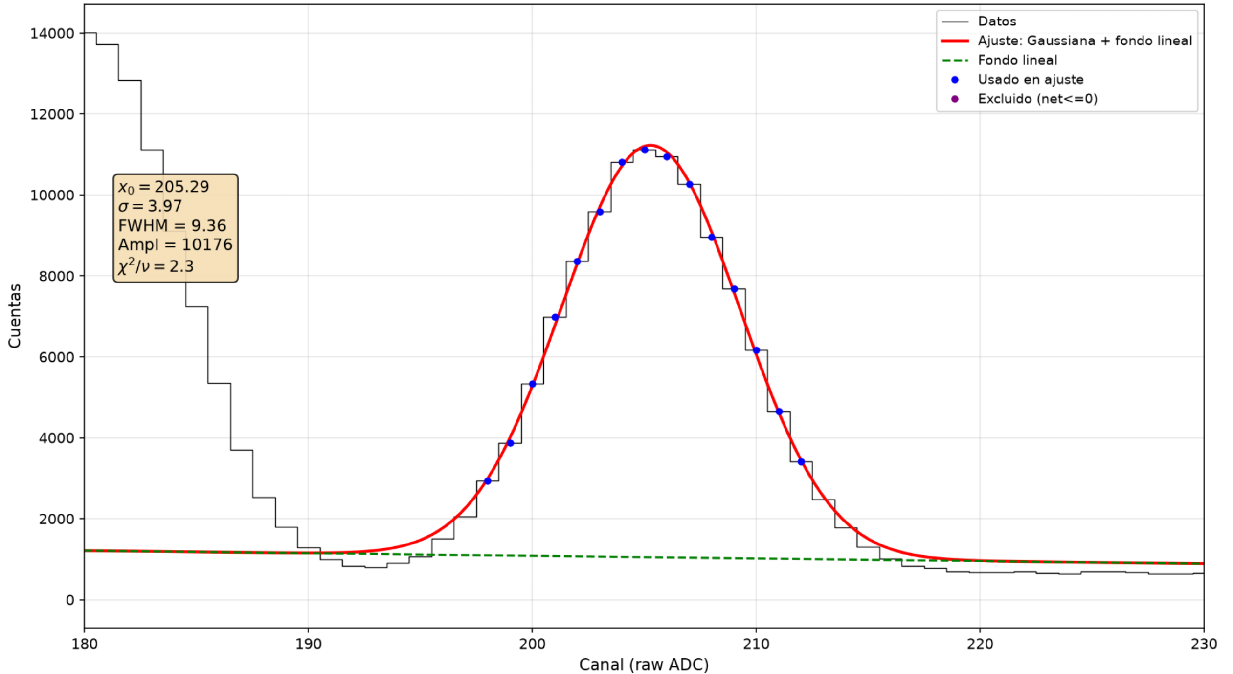
60-Co-caracterización — Pico 1332 keV (MCAch1, detector móvil)
