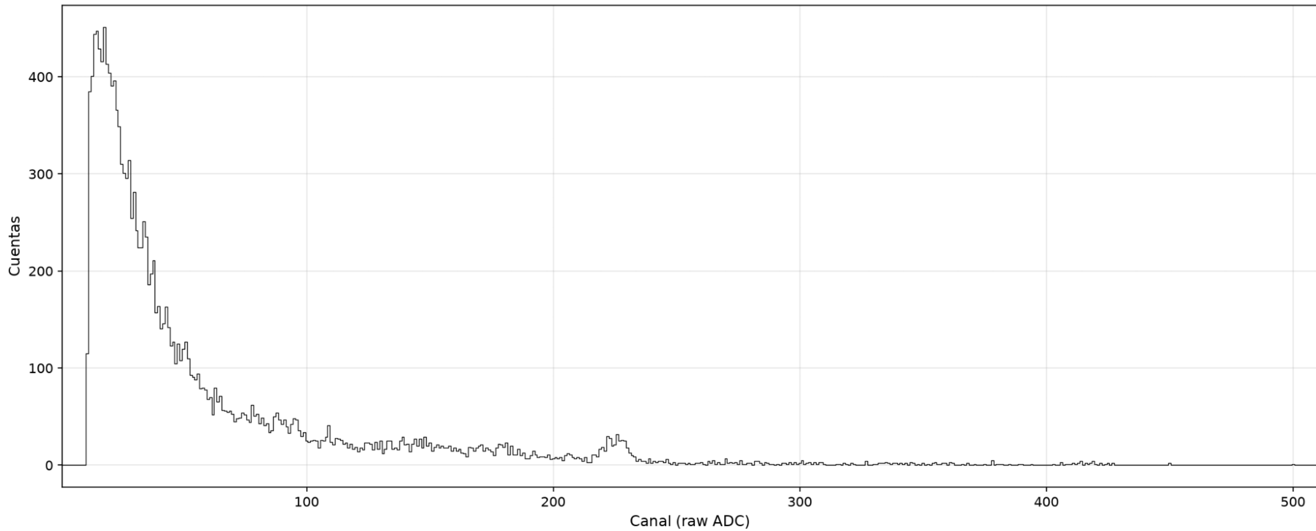
60Co-F-coin — MCAch1 (detector móvil)
