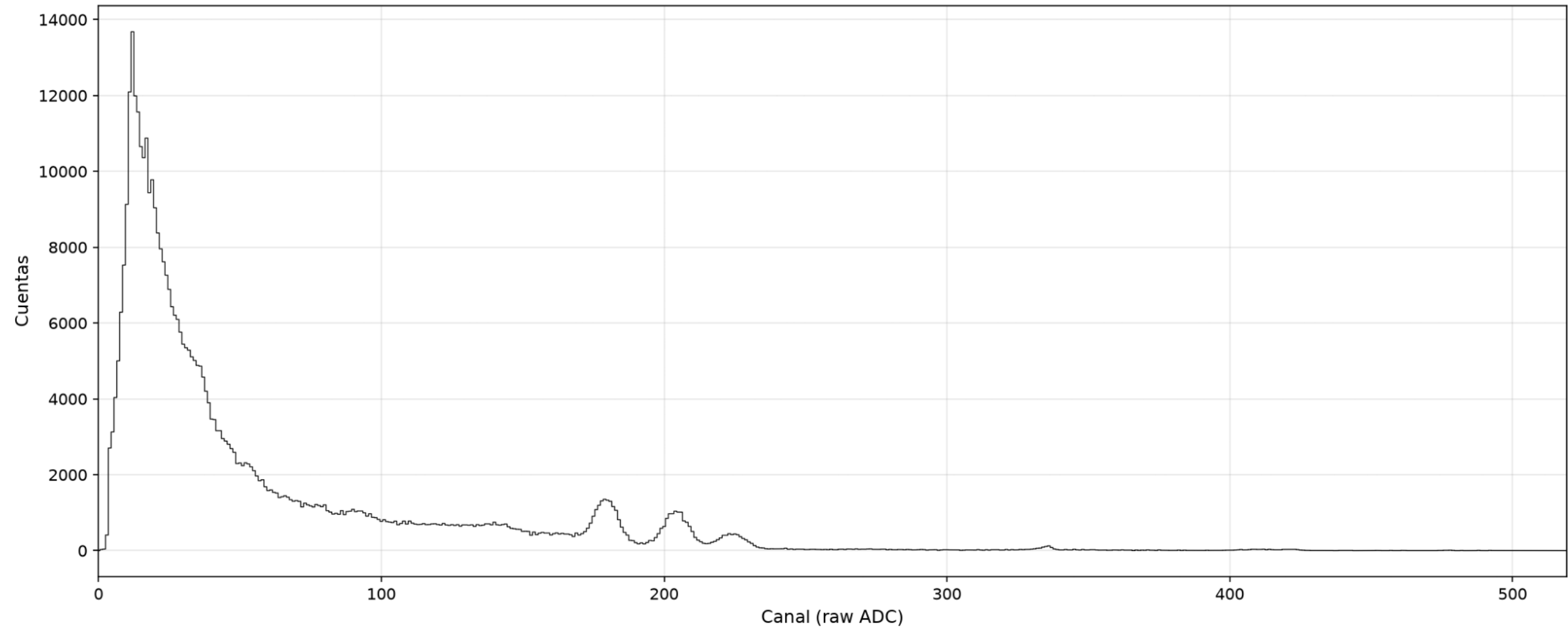
60-Co-157,5-coin — MCAch1 (detector móvil)
