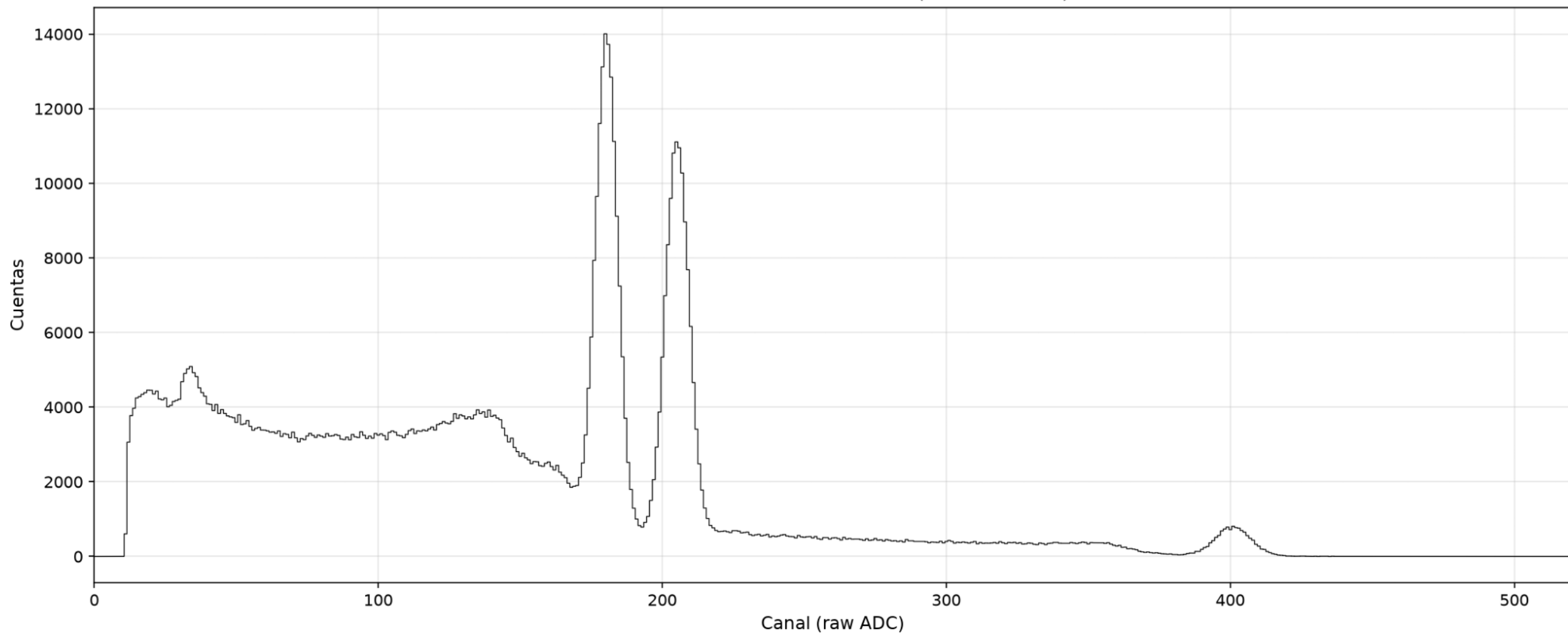
60-Co-caracterización — MCACH1 (detector móvil)
