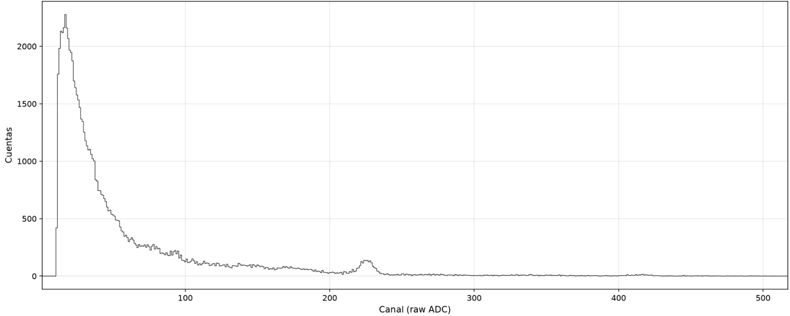
F-F-coin — MCAch1 (detector móvil)
