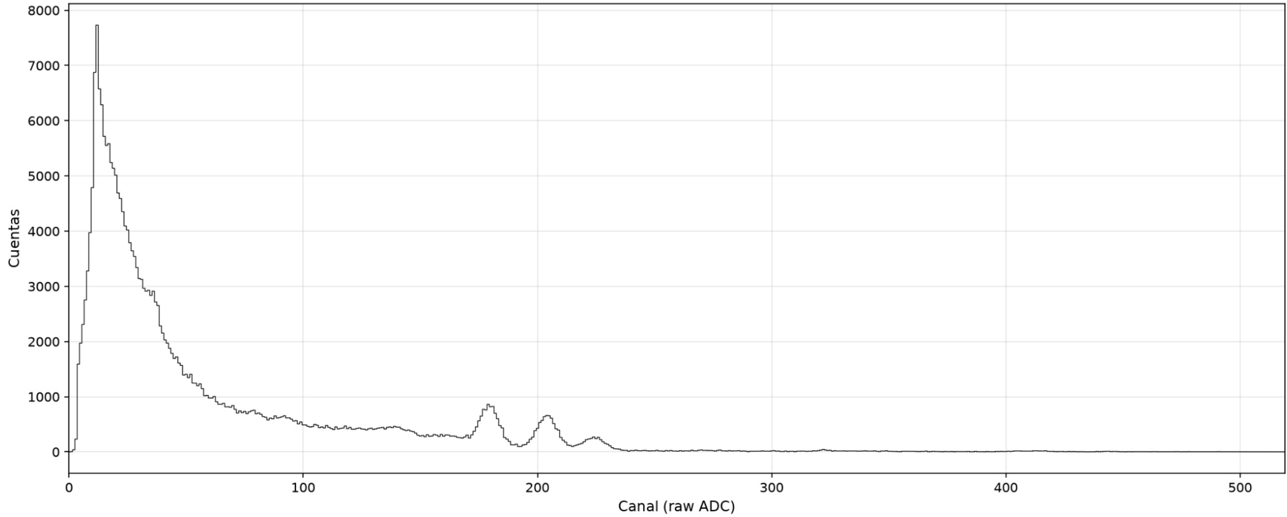
60-Co-112,5-coin — MCAch1 (detector móvil)
