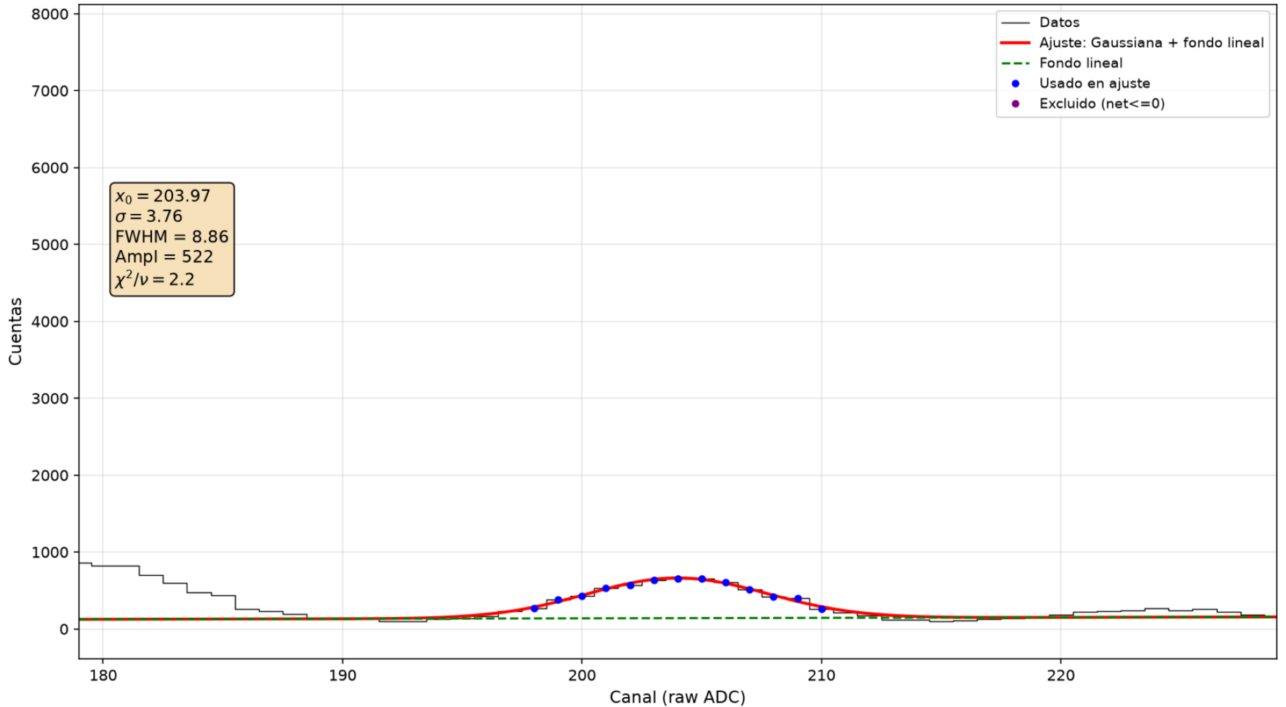
60-Co-112,5-coin — Pico 1332 keV (MCAch1, detector móvil)
