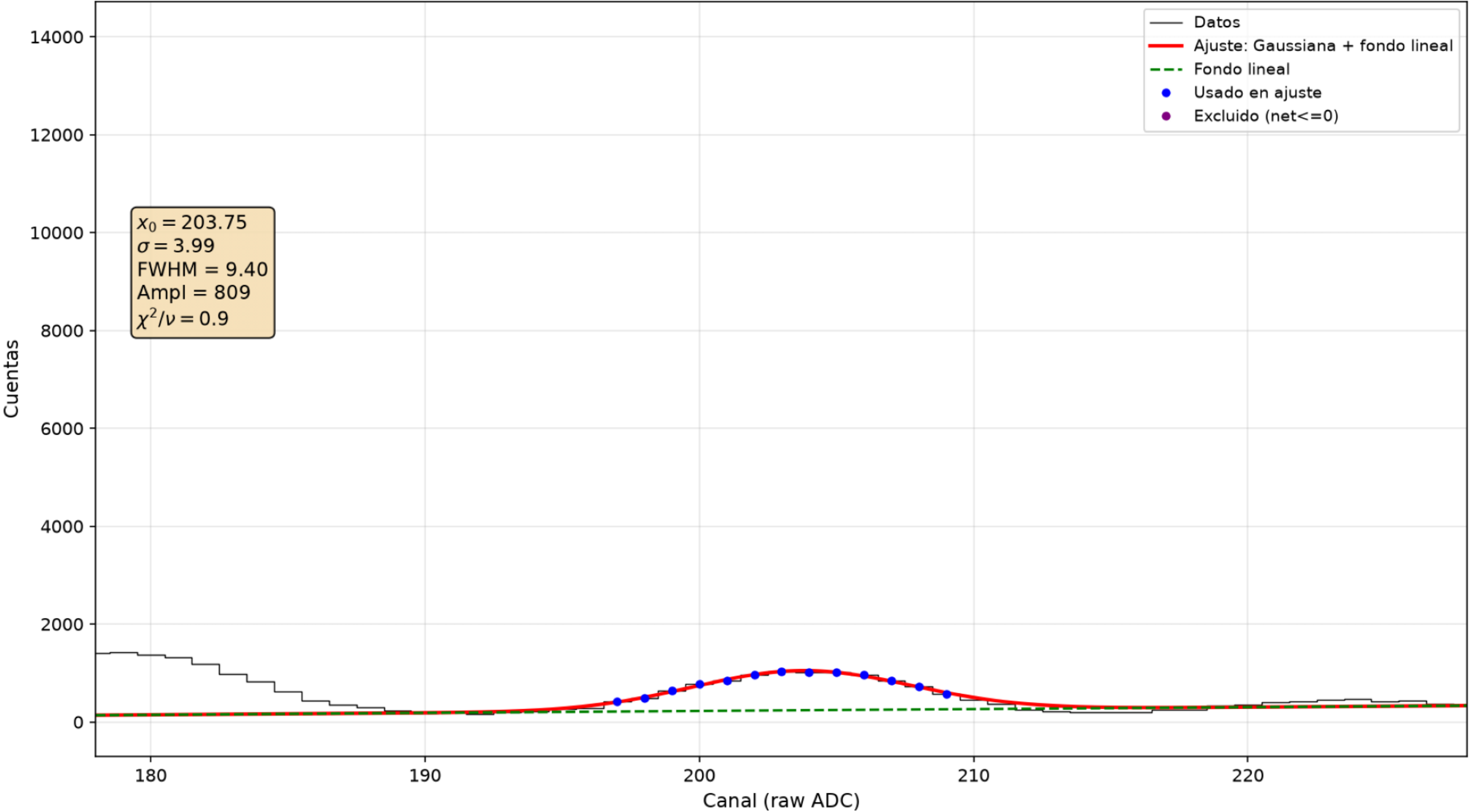
60-Co-22,5-coin — Pico 1332 keV (MCACH1, detector móvil)
