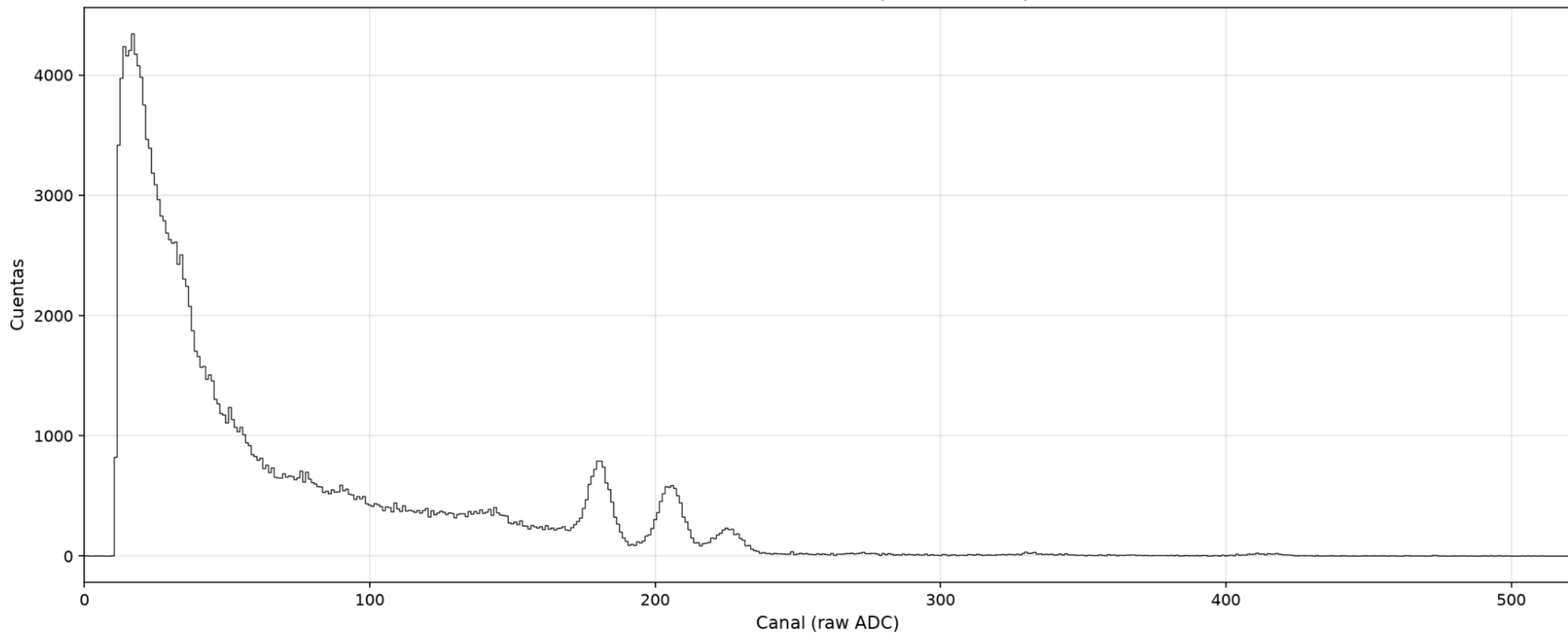
60Co-180-coin — MCACH1 (detector móvil)
