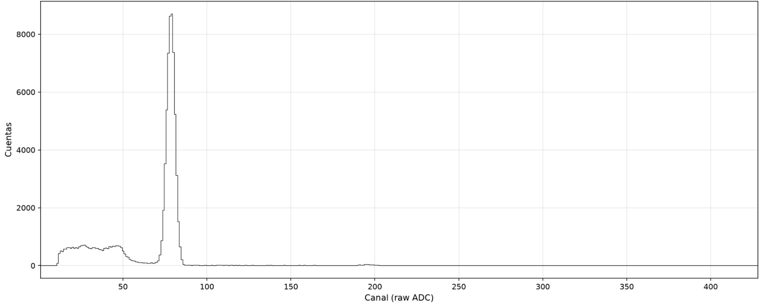
^{22}\text{Na} -180-coin — MCACH1 (detector móvil)
