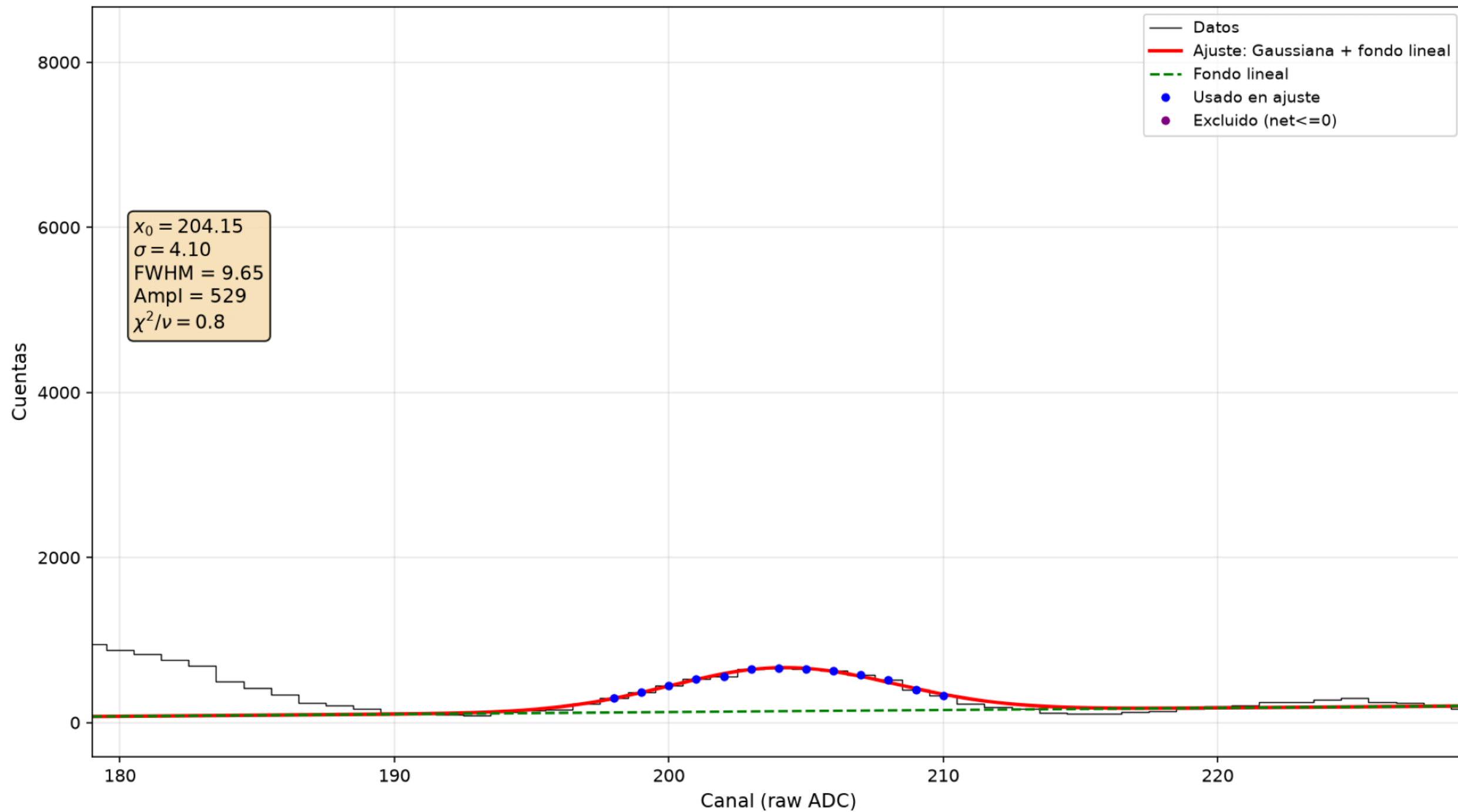
60-Co-67,5-coin — Pico 1332 keV (MCAch1, detector móvil)
