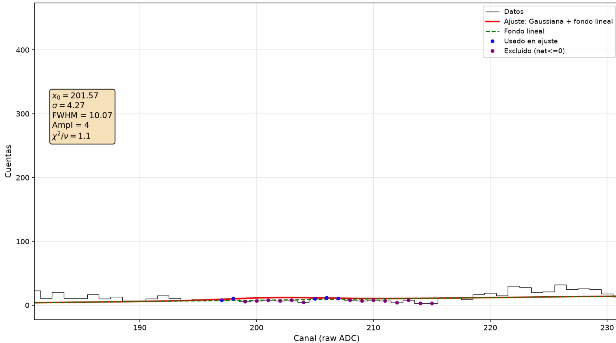
60Co-F-coin — Pico 1332 keV (MCAch1, detector móvil)
