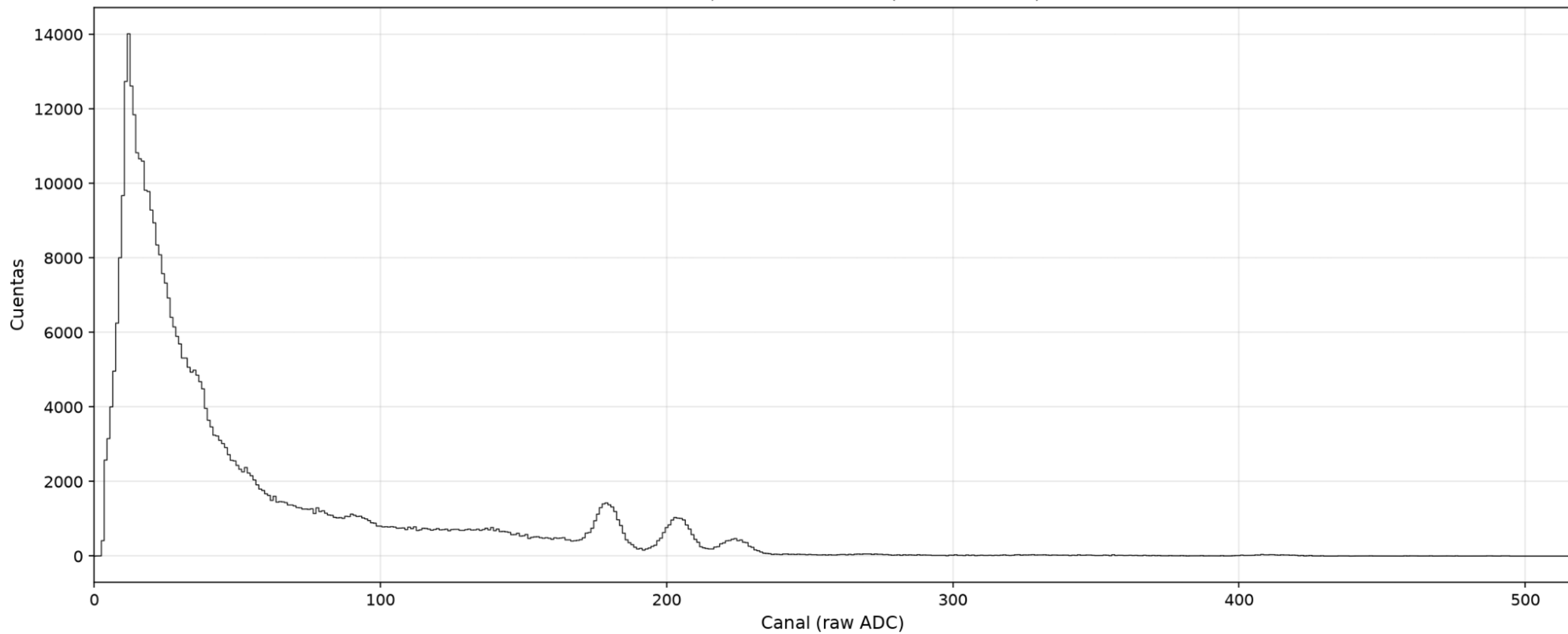
60-Co-22,5-coin — MCAch1 (detector móvil)
