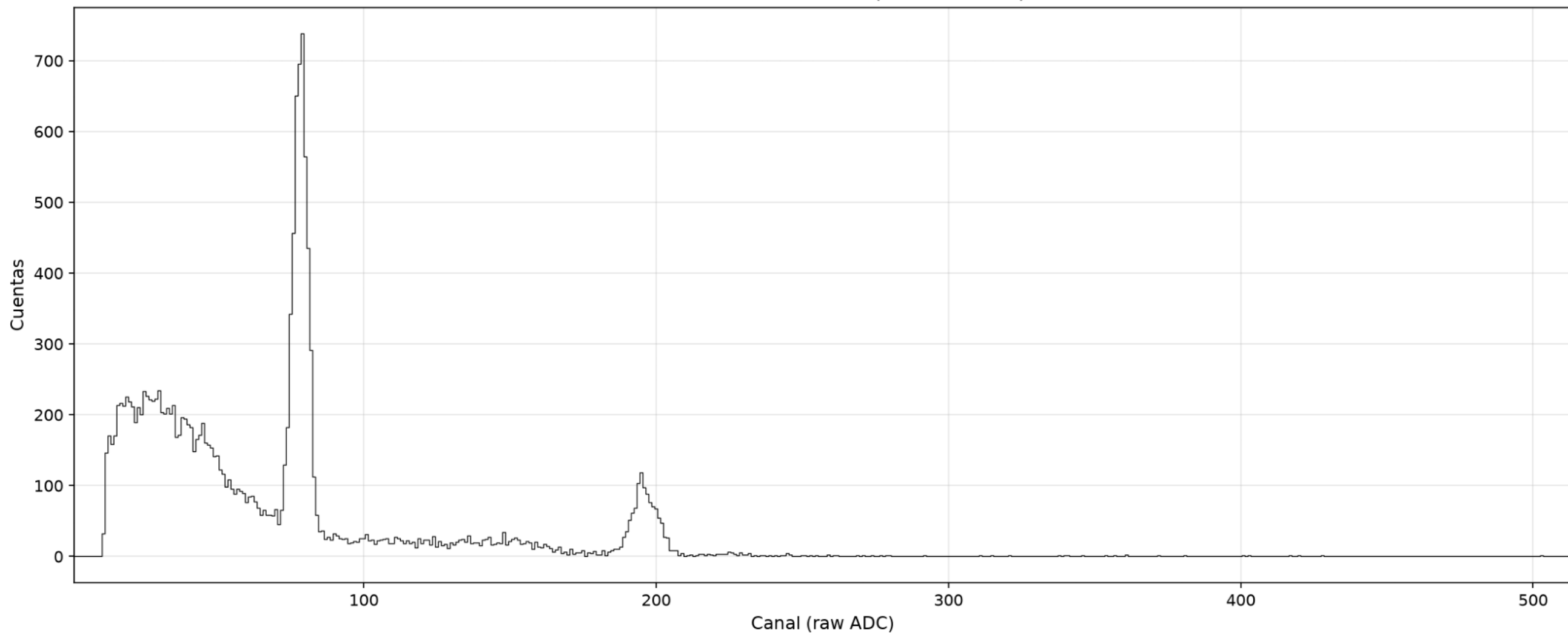
^{22}\text{Na} -157-coin — MCACH1 (detector móvil)
