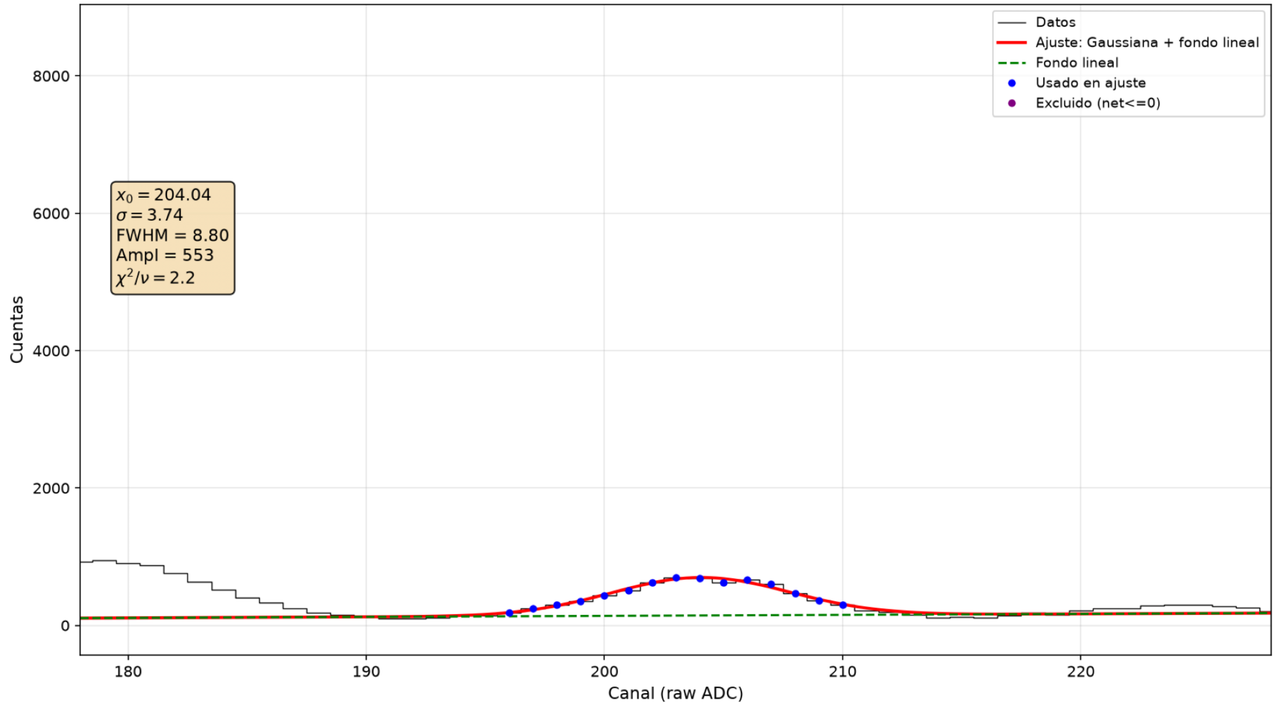
60-Co-45-coin — Pico 1332 keV (MCAch1, detector móvil)
