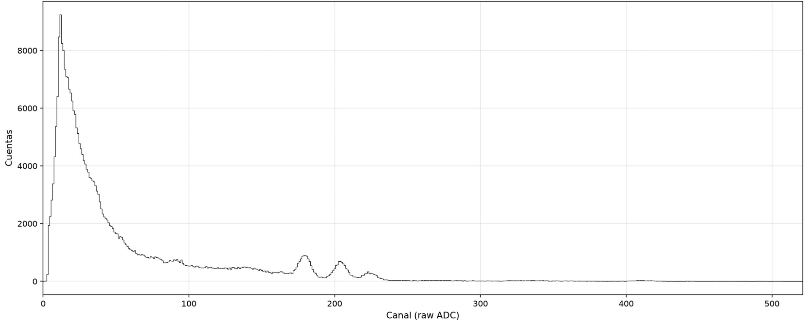
60-Co-135-coin — MCAch1 (detector móvil)
