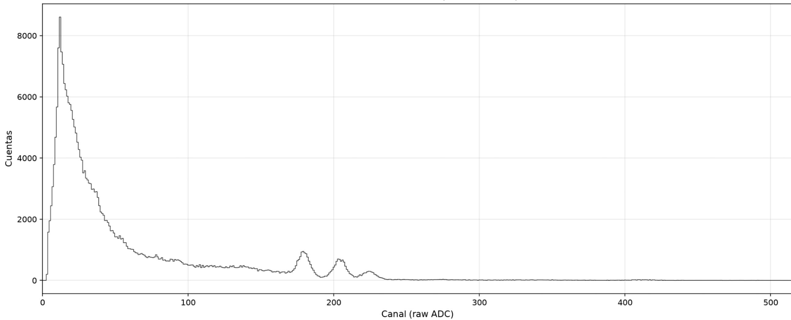
60-Co-45-coin — MCAch1 (detector móvil)
