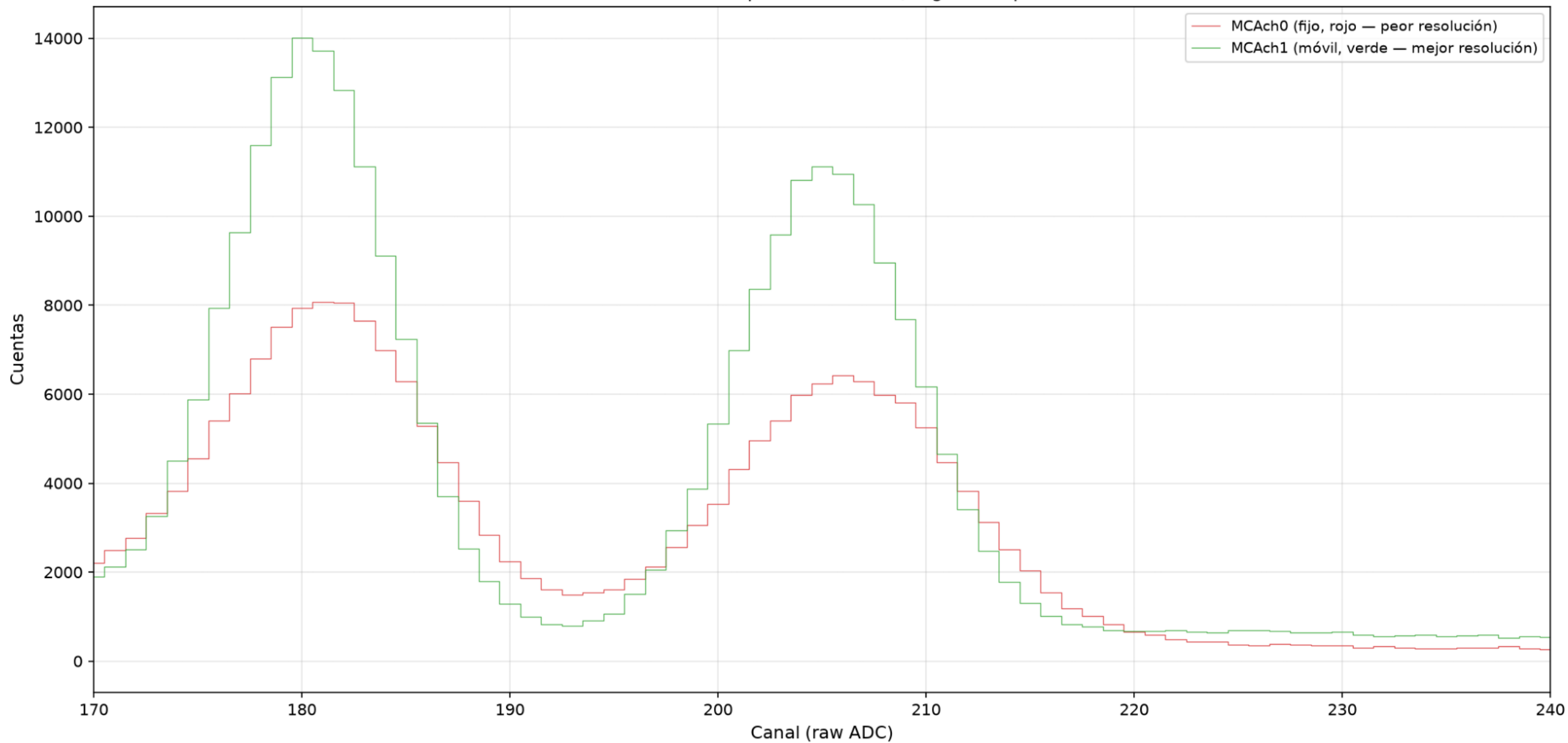
60-Co-caracterización — Comparación directa, región del pico de 1332 keV
