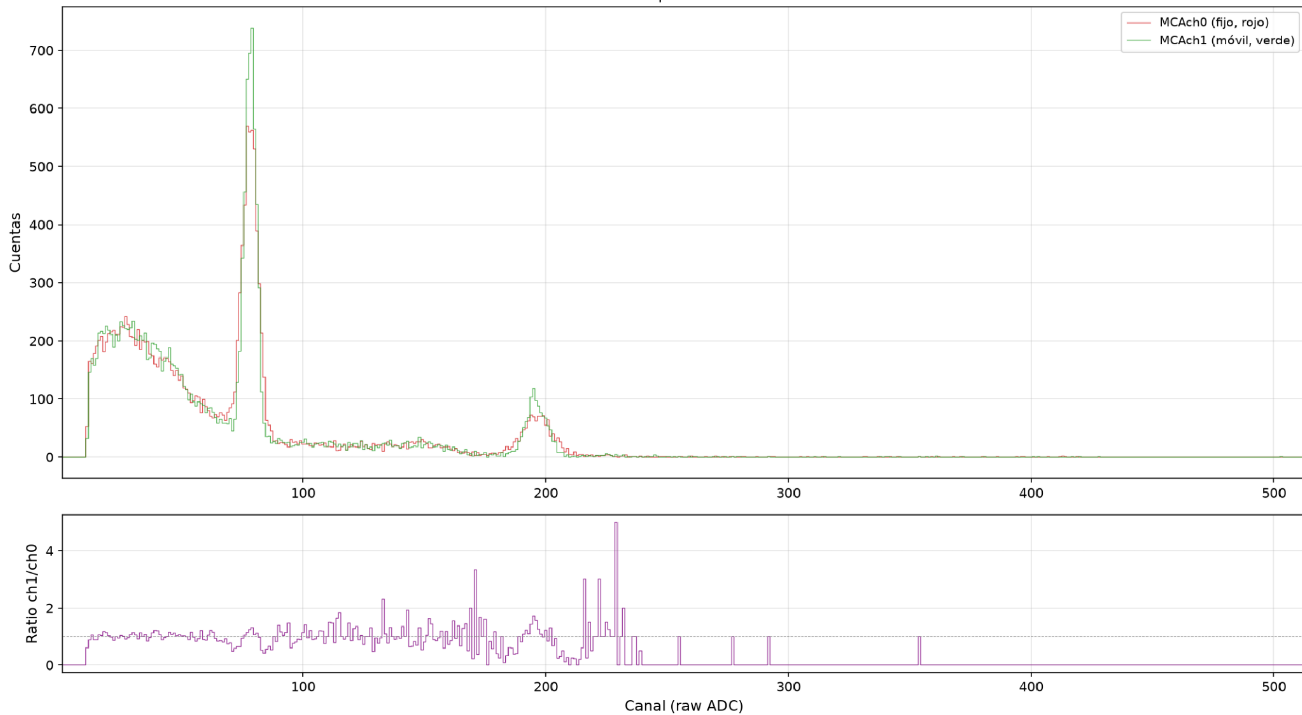
22Na-157-coin — Comparación MCACH0 vs MCACH1
