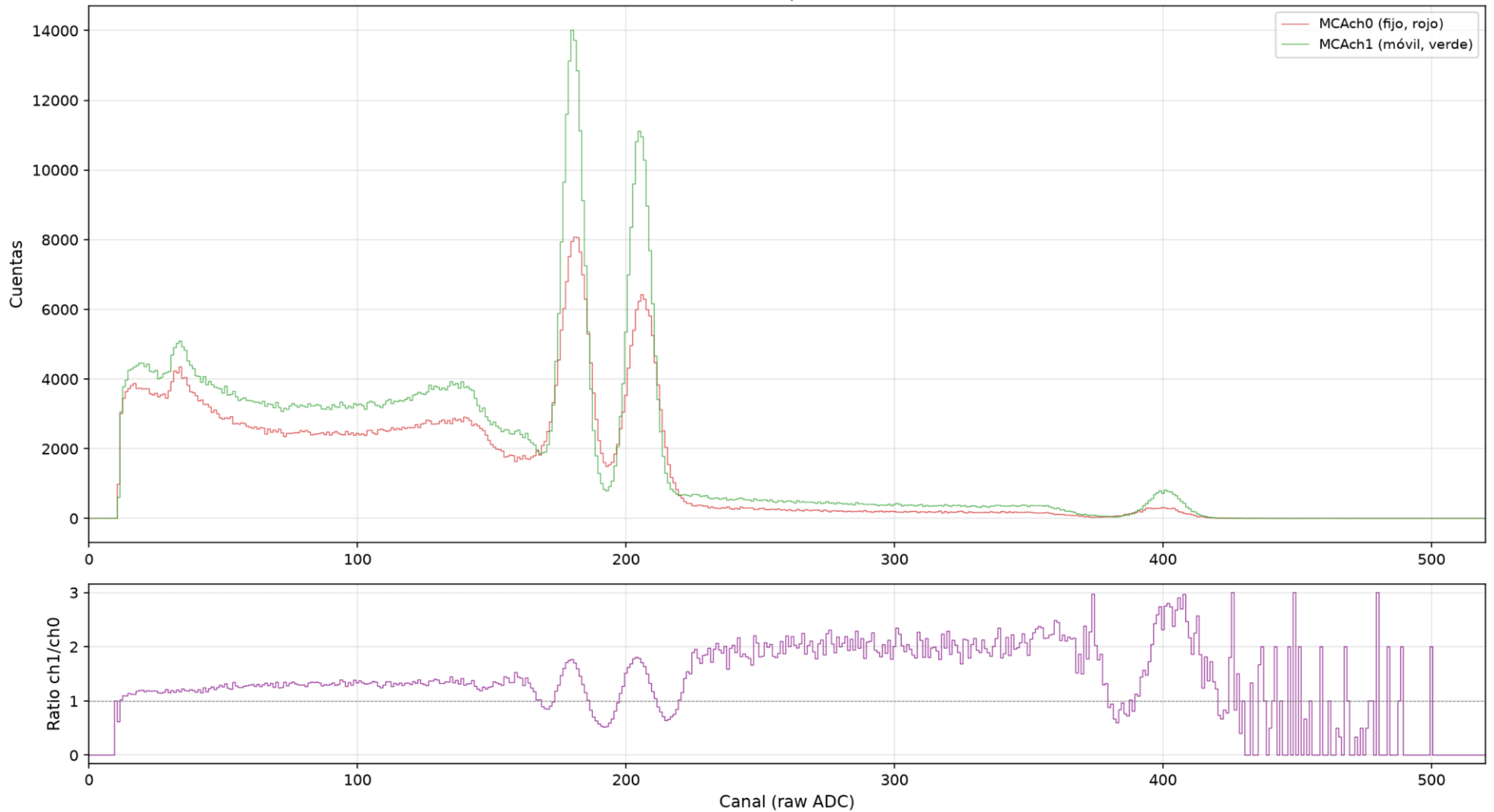
60-Co-caracterización — Comparación MCACH0 vs MCACH1
