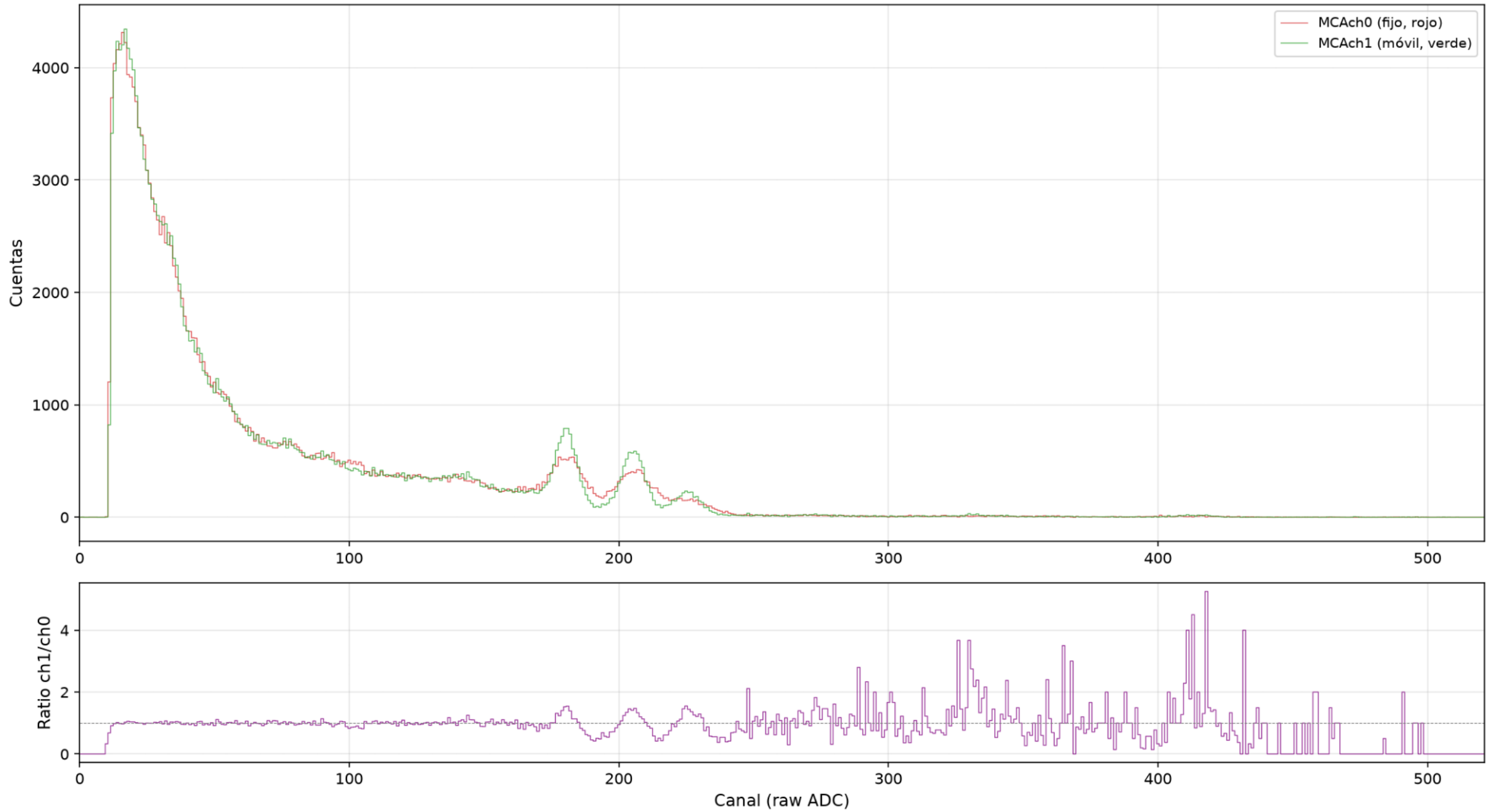
60Co-180-coin — Comparación MCAch0 vs MCAch1
