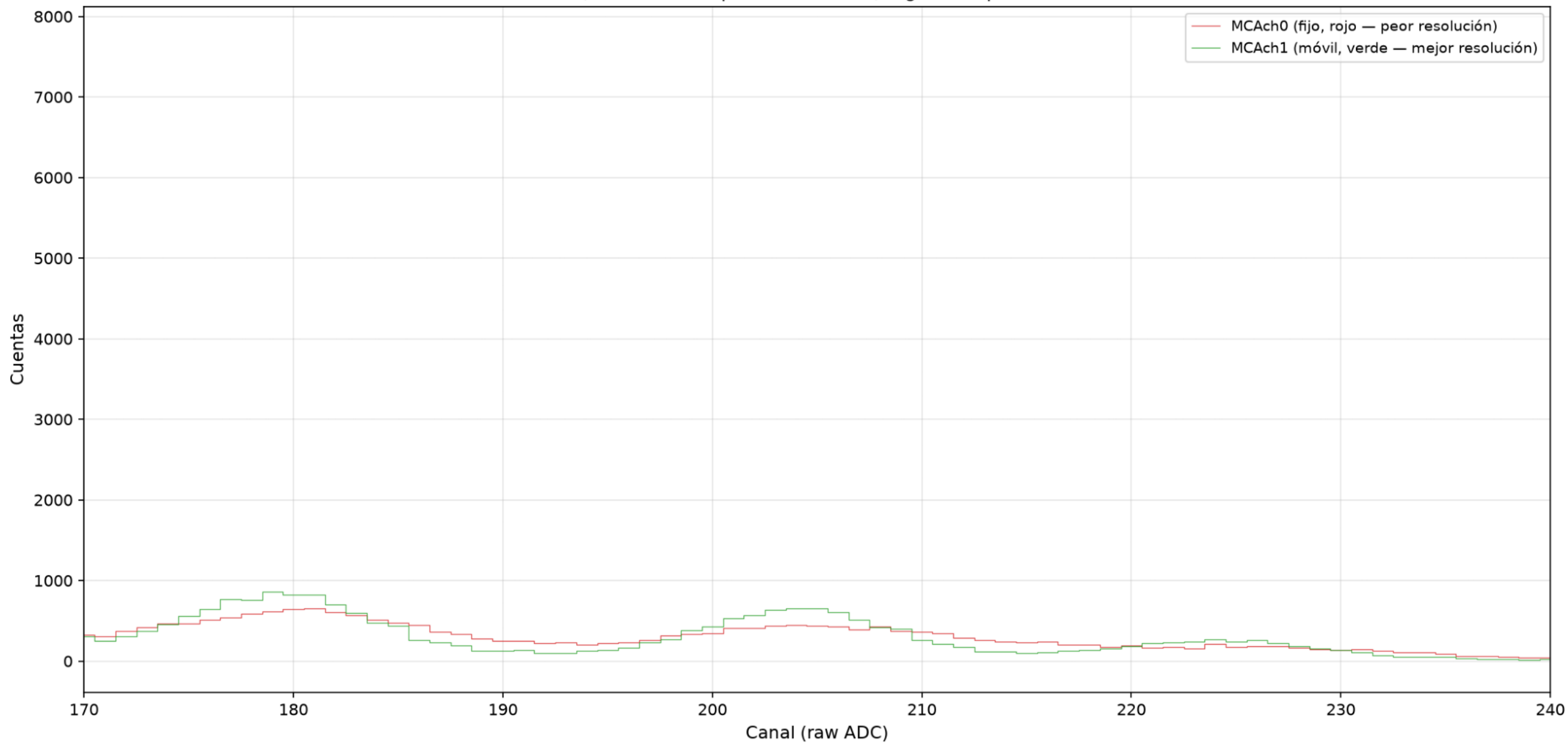
60-Co-112,5-coin — Comparación directa, región del pico de 1332 keV
