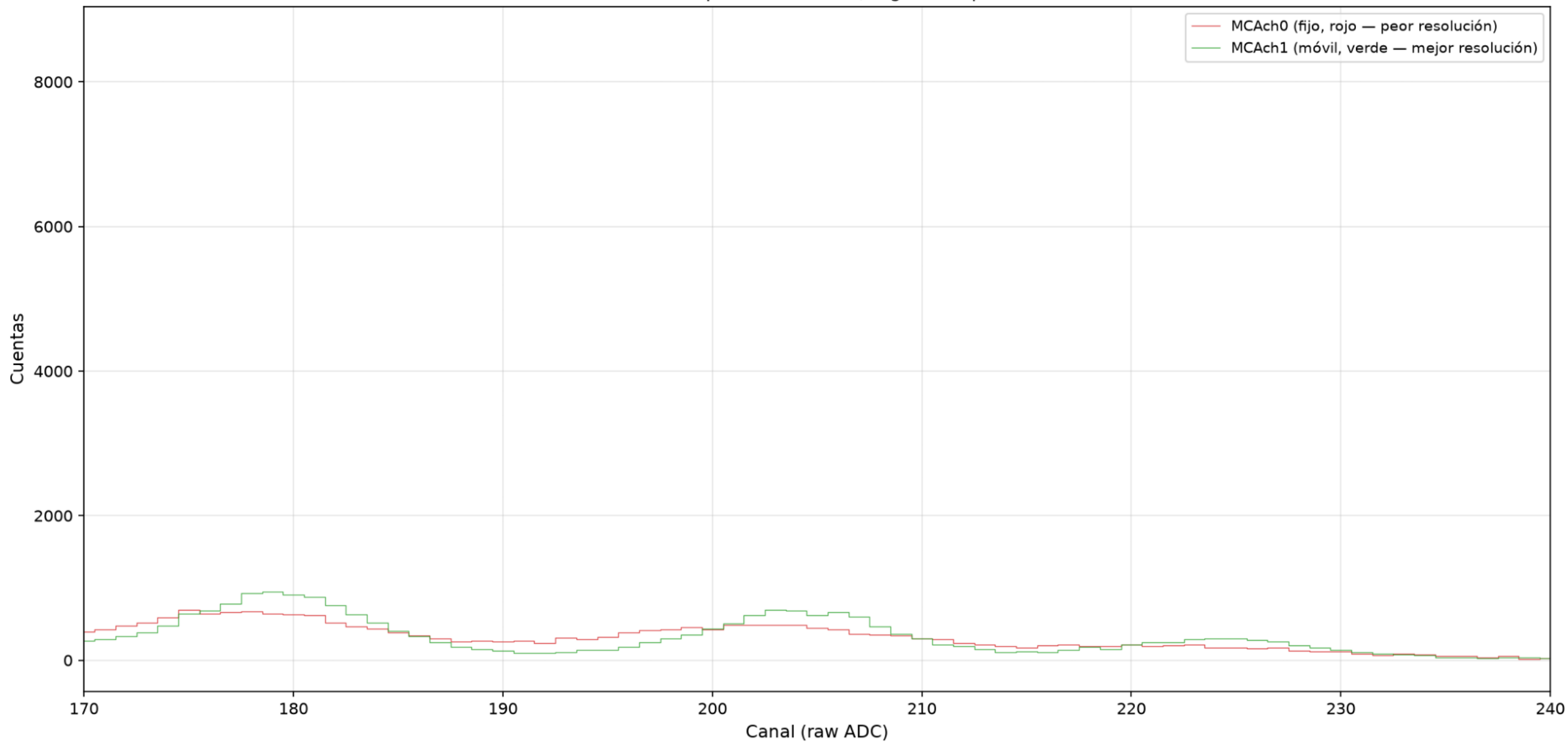
60-Co-45-coin — Comparación directa, región del pico de 1332 keV
