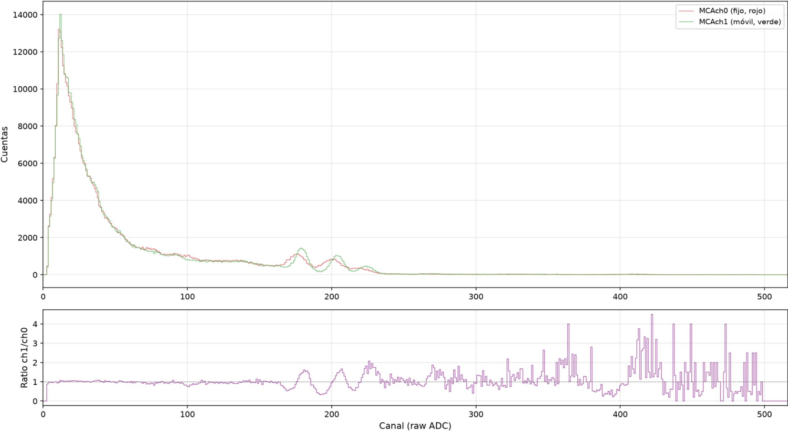
60-Co-22,5-coin — Comparación MCACH0 vs MCACH1
