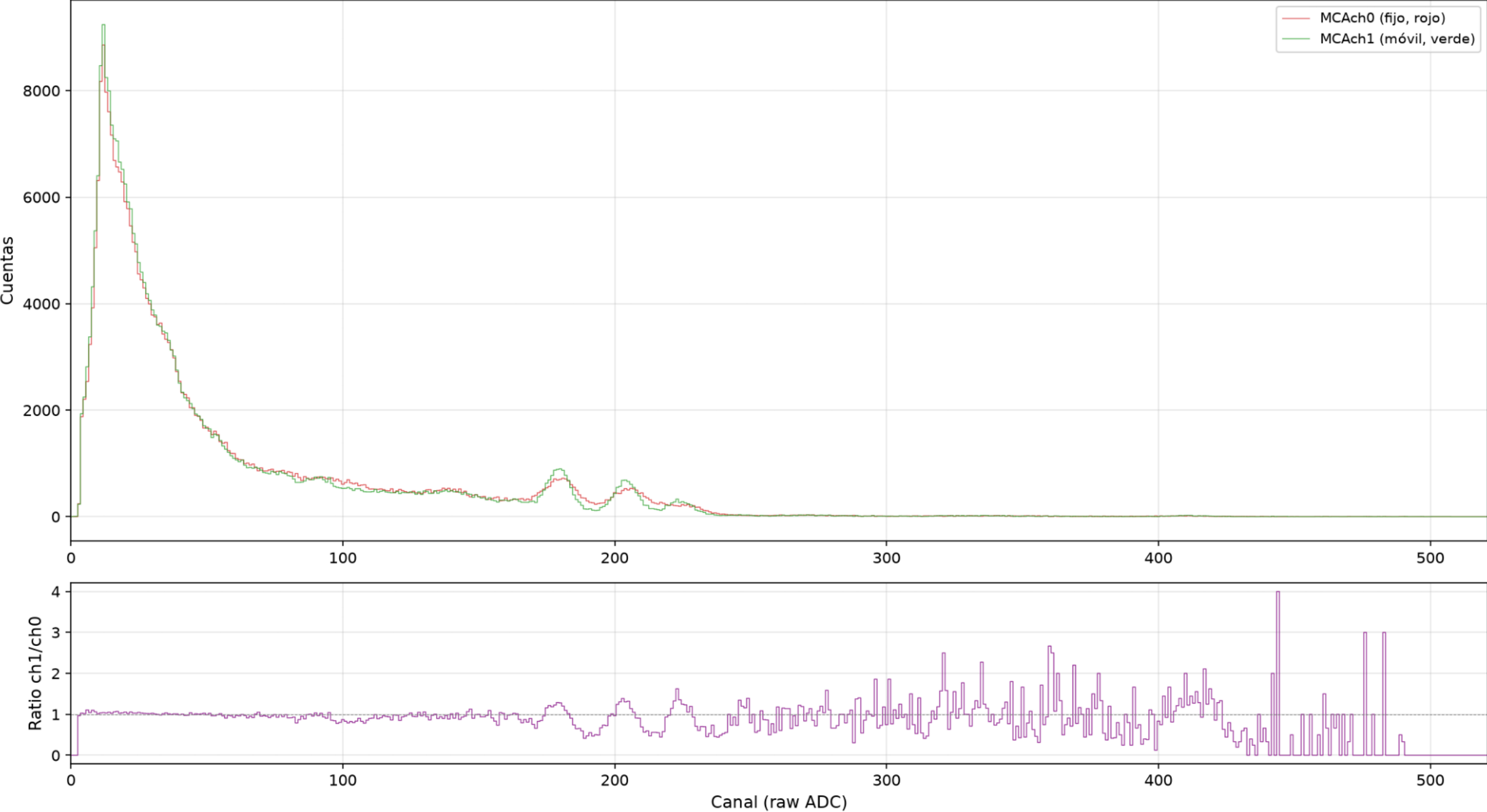
60-Co-135-coin — Comparación MCAch0 vs MCAch1
