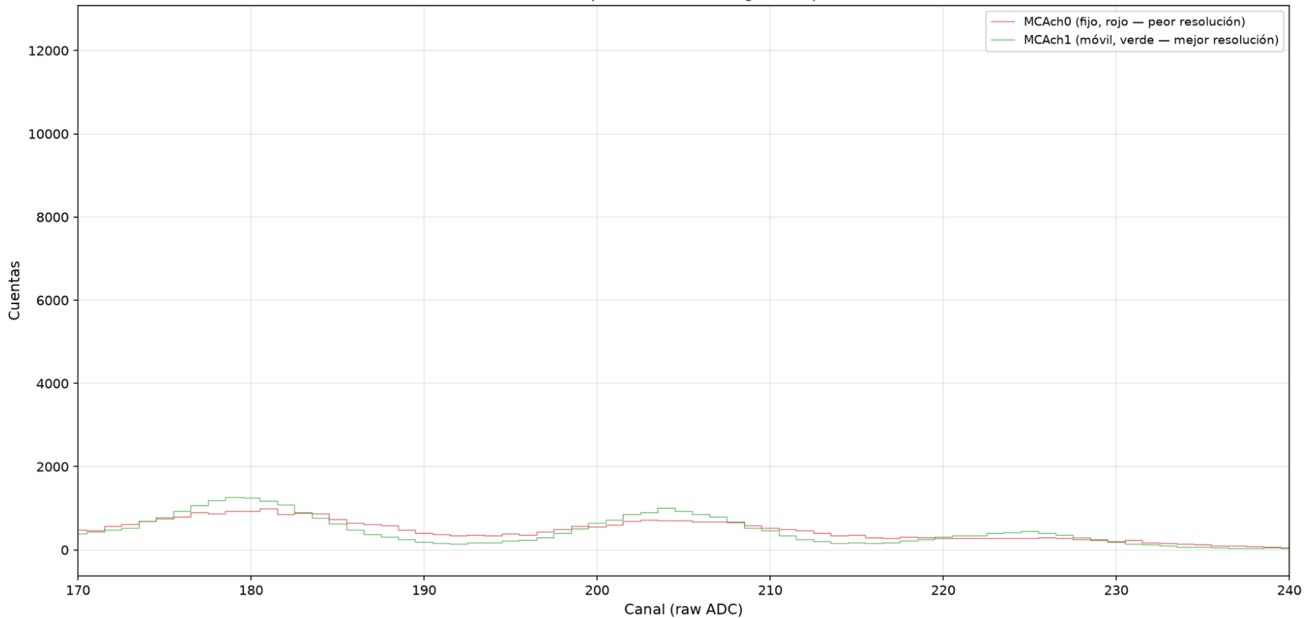
60-Co-90-coin — Comparación directa, región del pico de 1332 keV
