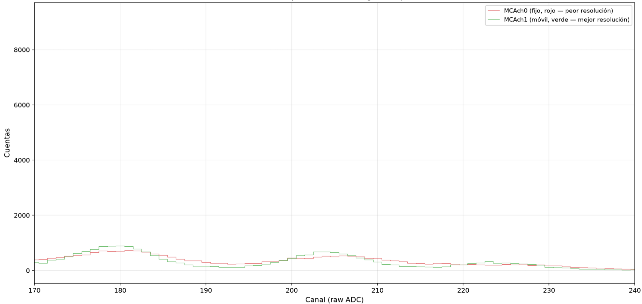
60-Co-135-coin — Comparación directa, región del pico de 1332 keV
