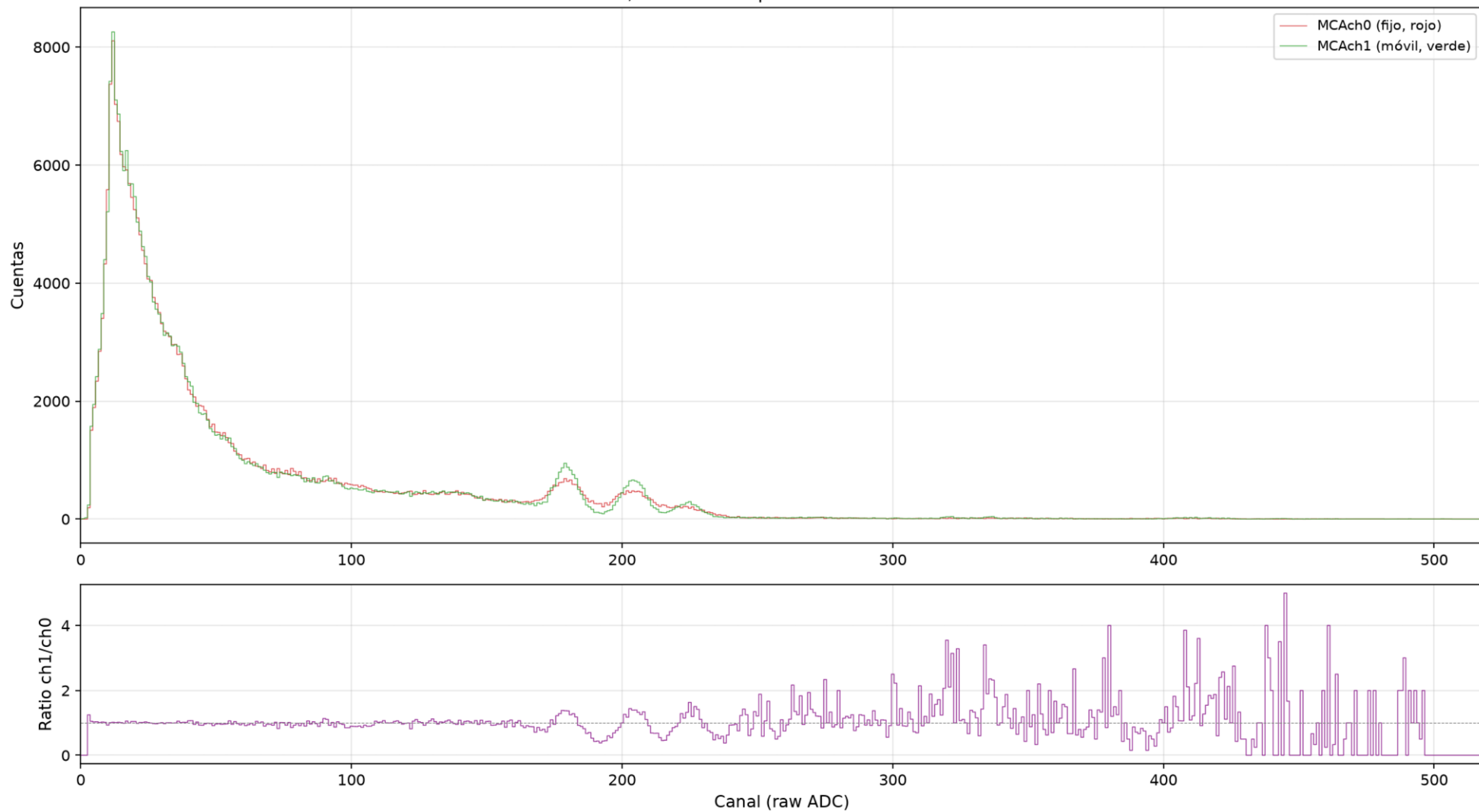
60-Co-67,5-coin — Comparación MCAch0 vs MCAch1
