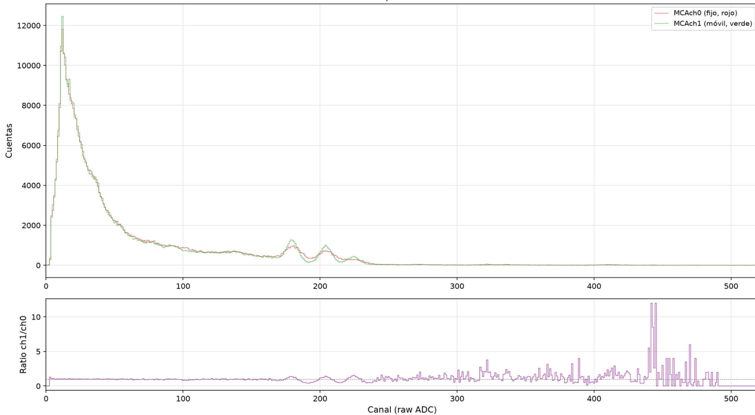
60-Co-90-coin — Comparación MCAch0 vs MCAch1
