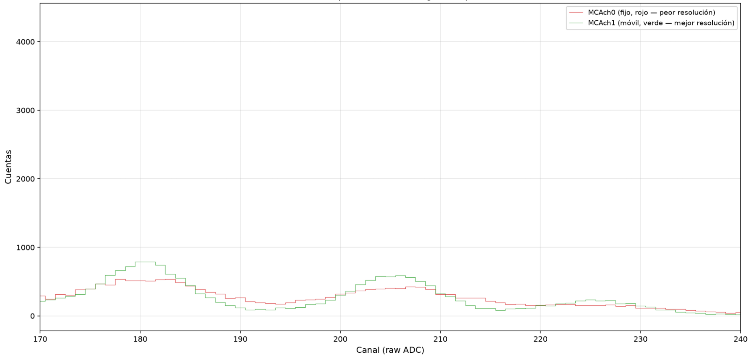
60Co-180-coin — Comparación directa, región del pico de 1332 keV
