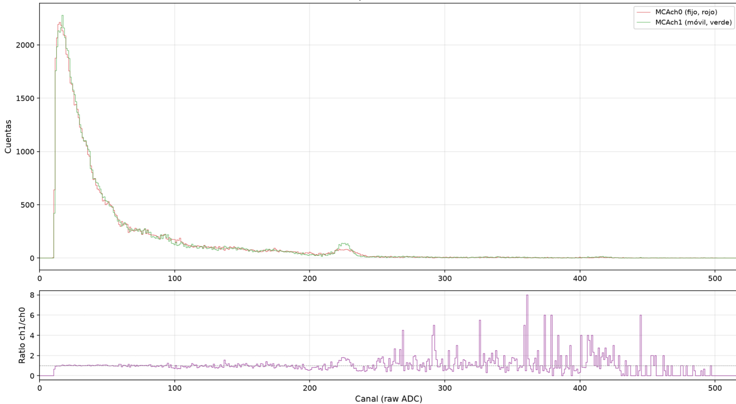
F-F-coin — Comparación MCAch0 vs MCAch1
