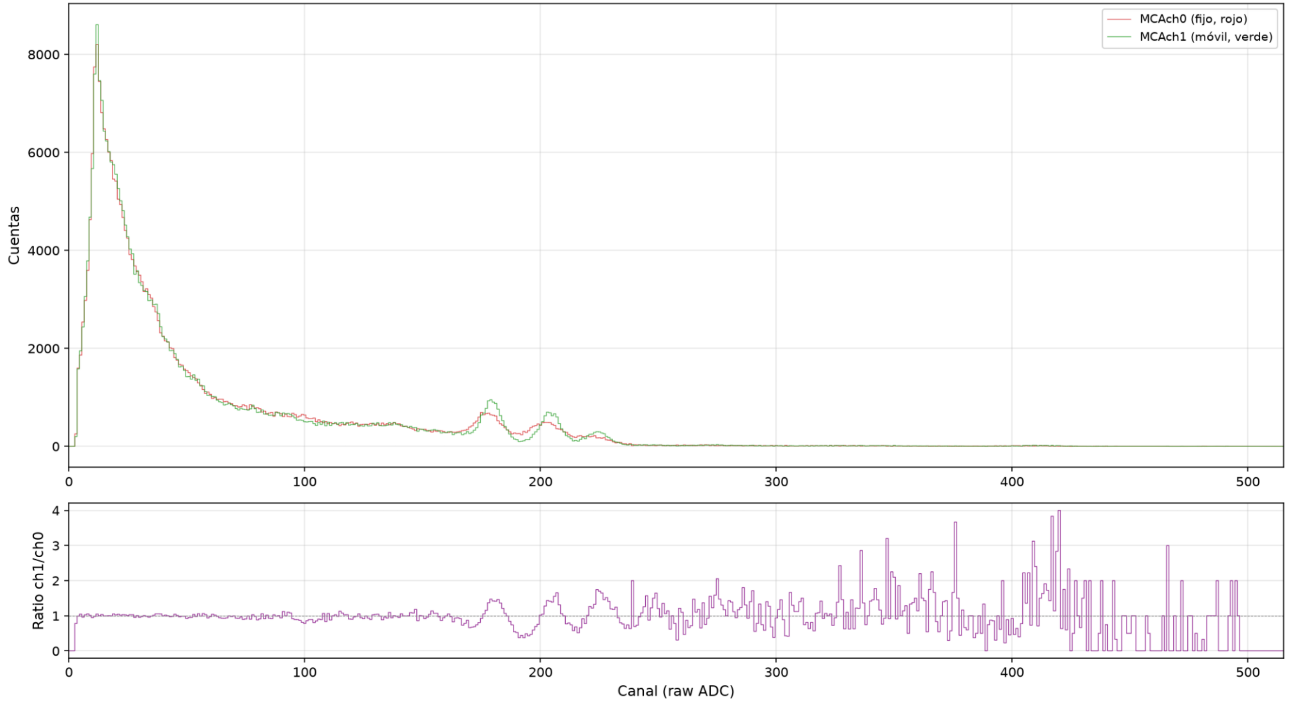
60-Co-45-coin — Comparación MCAch0 vs MCAch1
