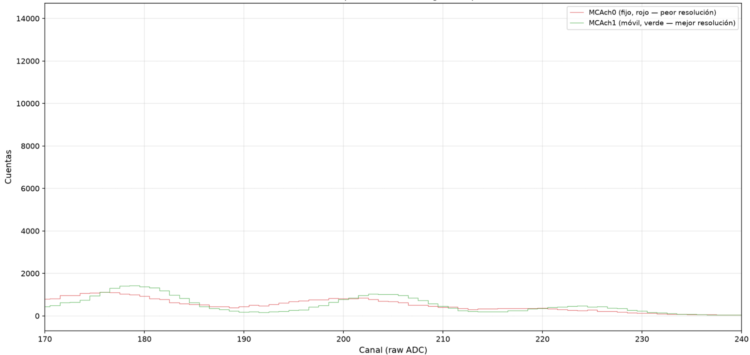
60-Co-22,5-coin — Comparación directa, región del pico de 1332 keV
