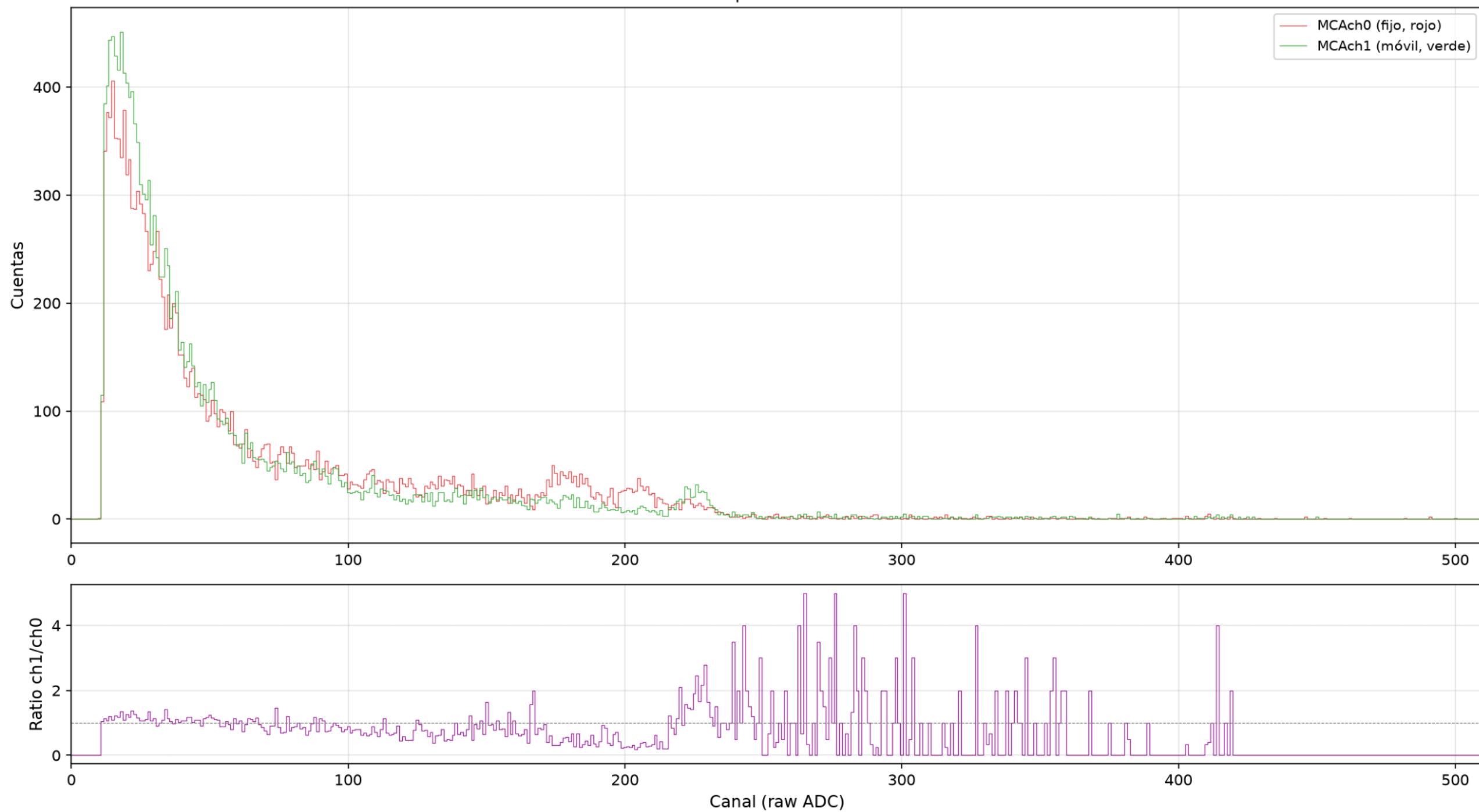
60Co-F-coin — Comparación MCAch0 vs MCAch1
