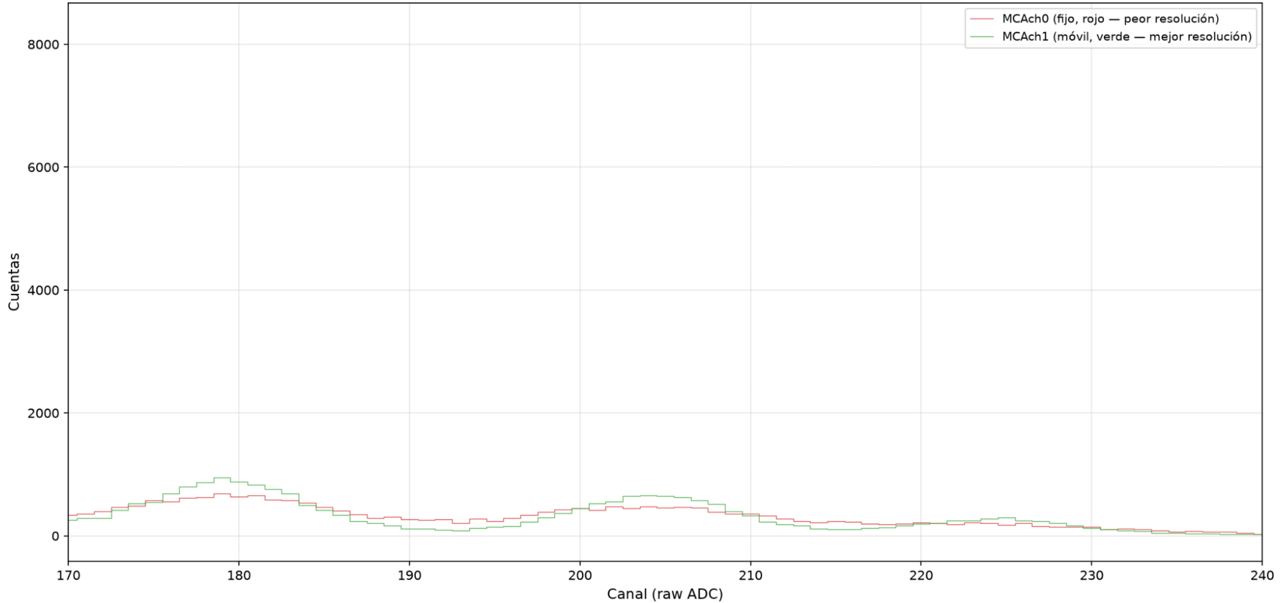
60-Co-67,5-coin — Comparación directa, región del pico de 1332 keV
