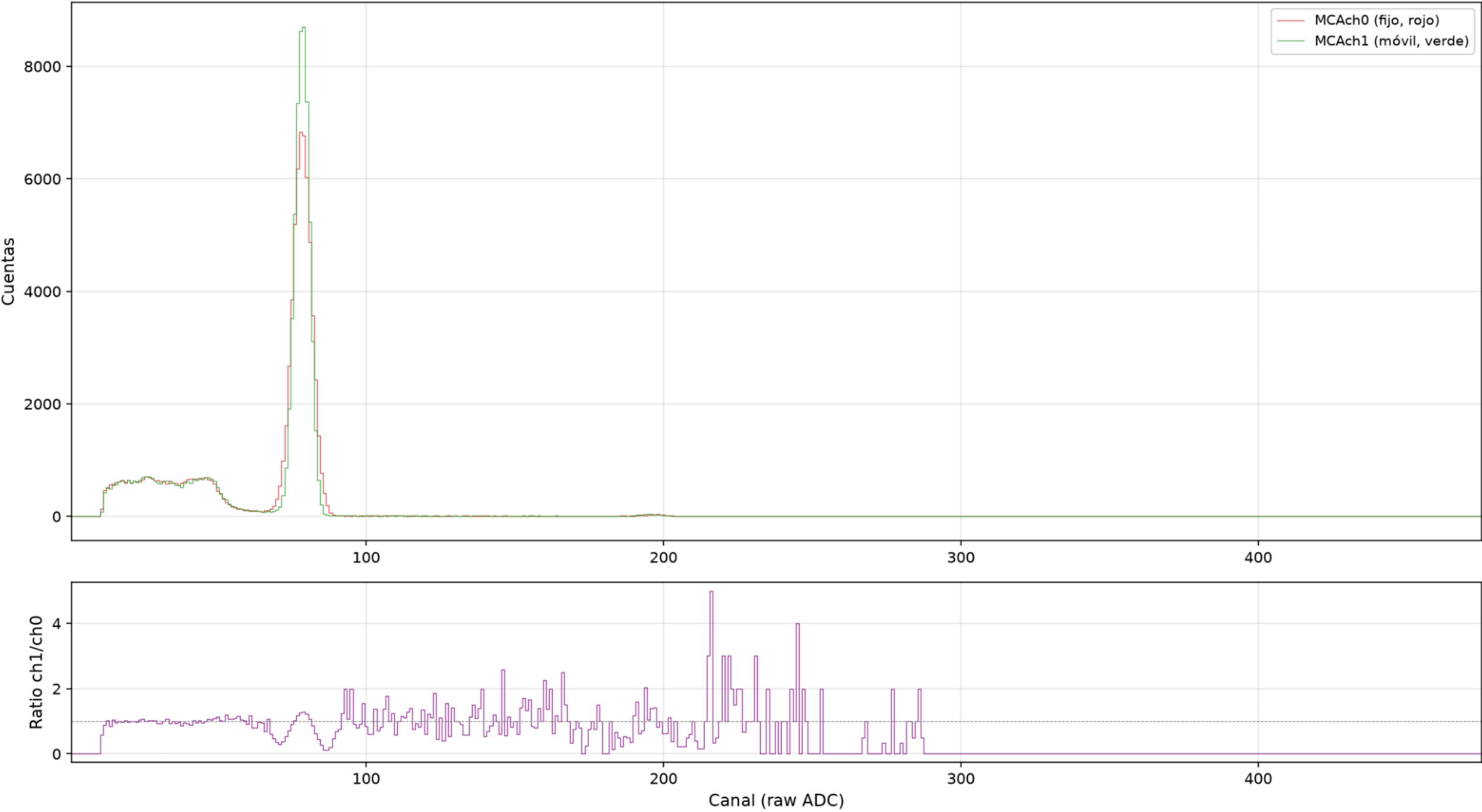
22Na-180-coin — Comparación MCAch0 vs MCAch1
