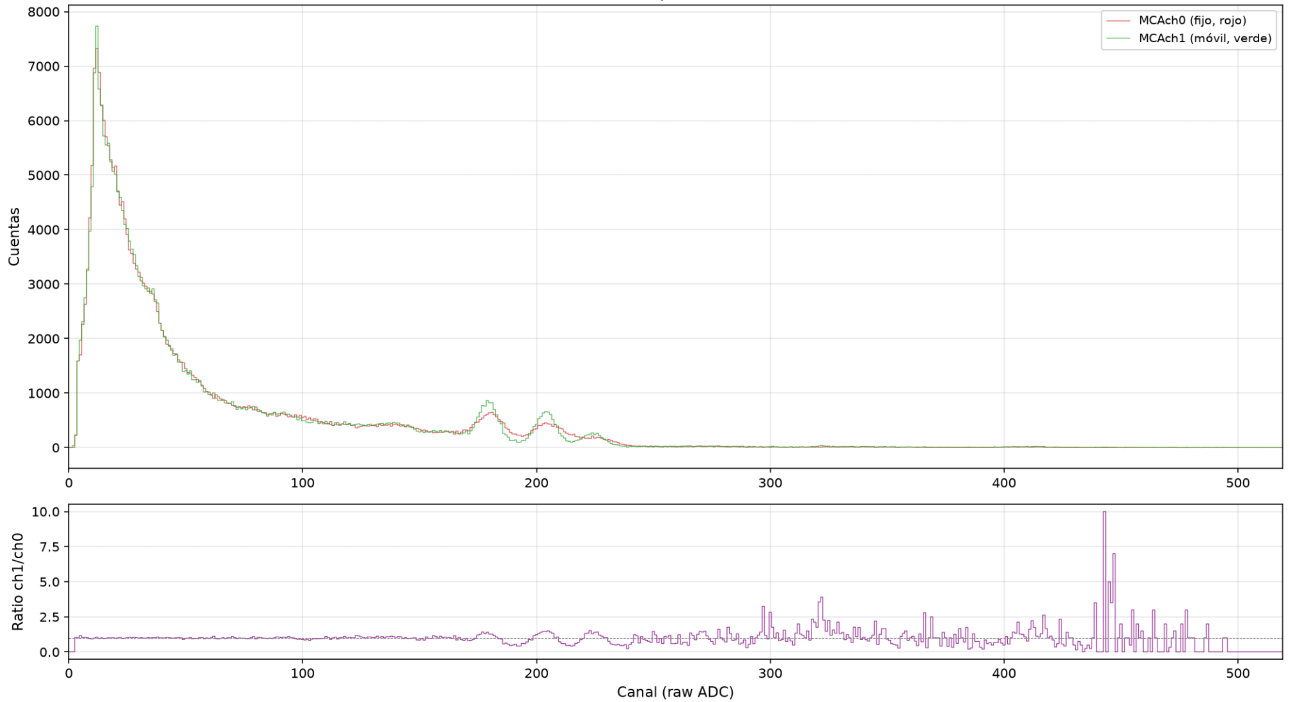
60-Co-112,5-coin — Comparación MCACH0 vs MCACH1
