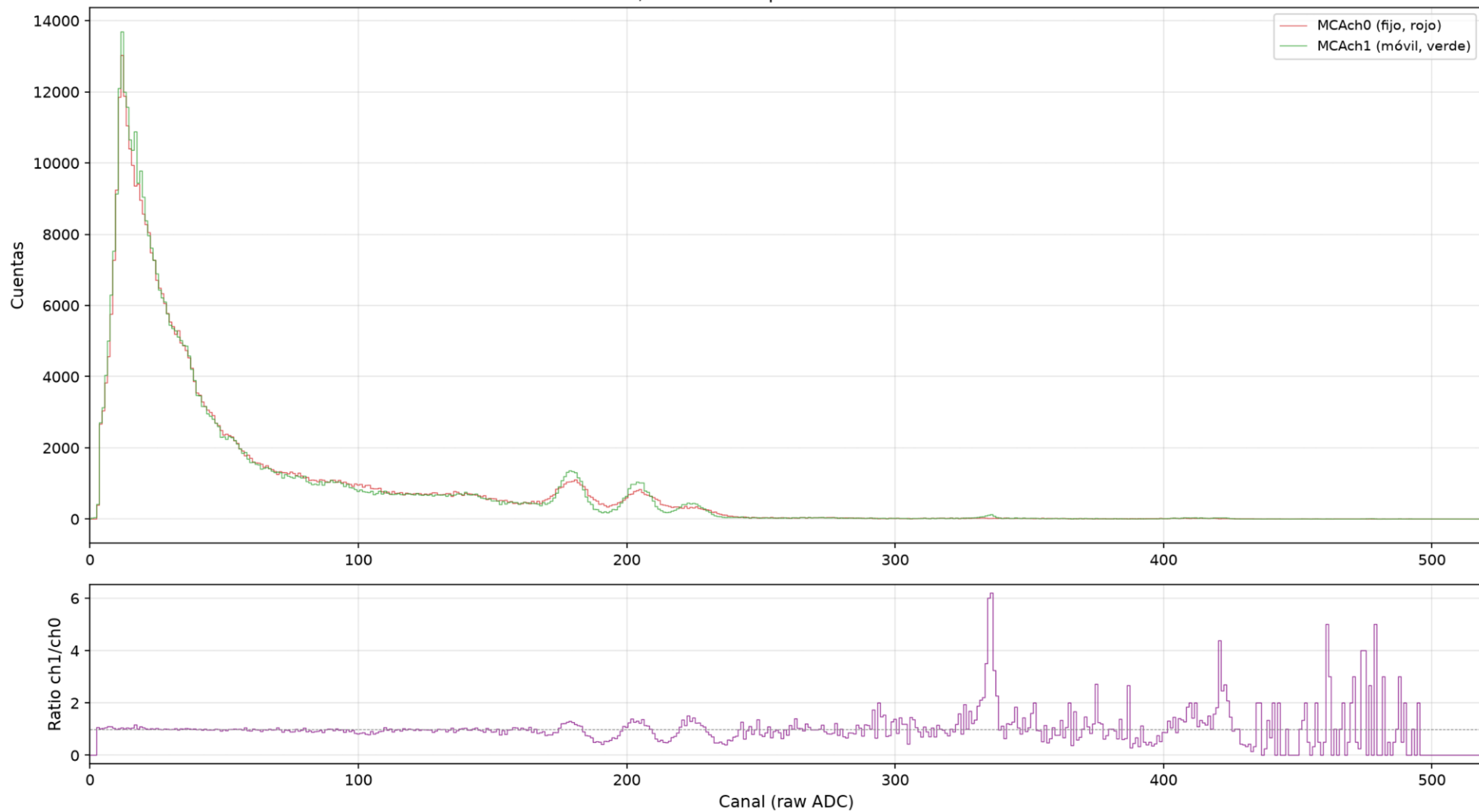
60-Co-157,5-coin — Comparación MCACH0 vs MCACH1
