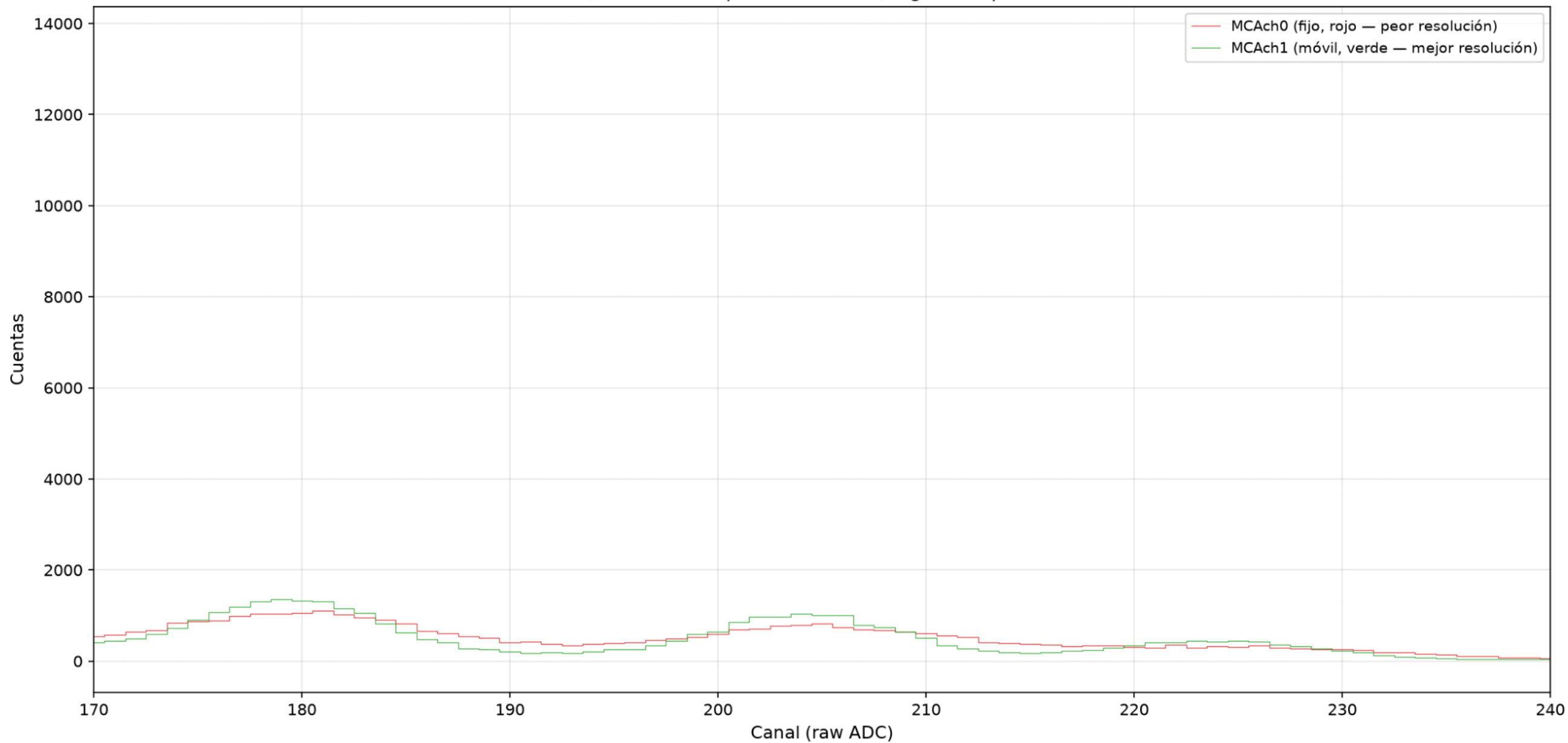
60-Co-157,5-coin — Comparación directa, región del pico de 1332 keV
