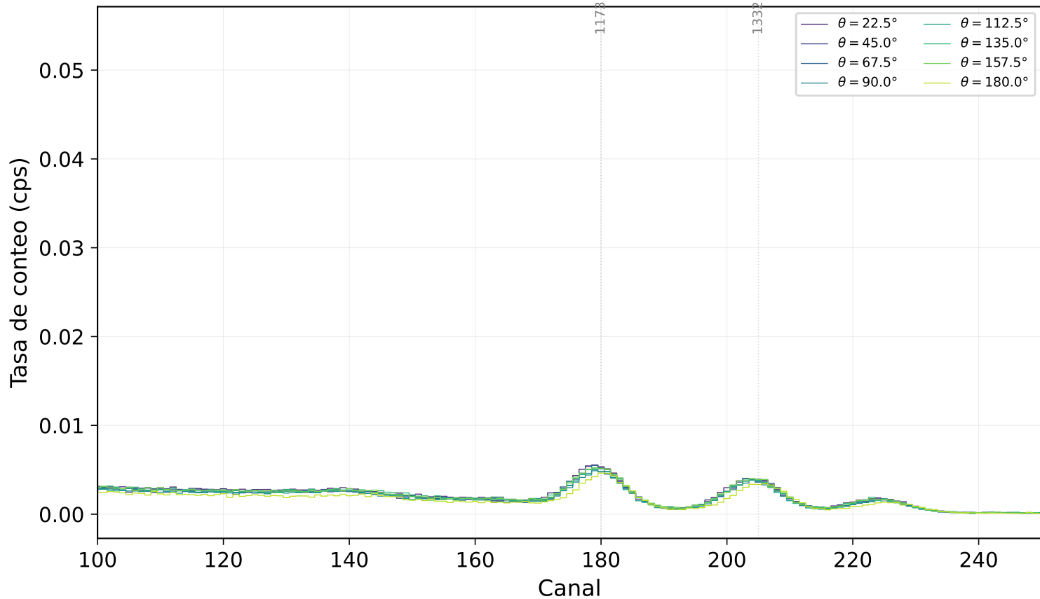
Espectros de coincidencia ^{60}\text{Co} a diferentes \angulos
