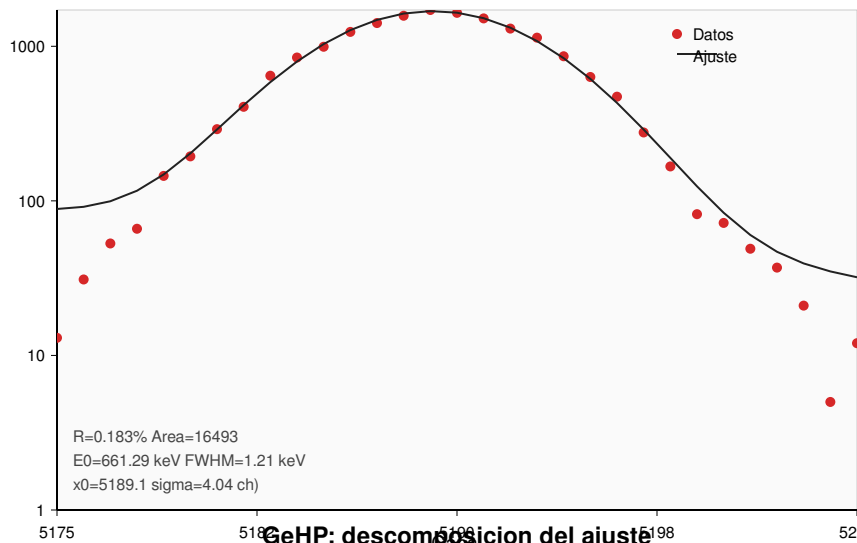
GeHP: descomposicion del ajuste
