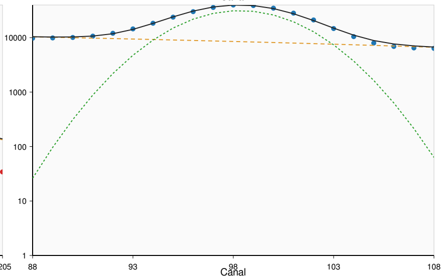
NaI(Tl): descomposicion del ajuste
