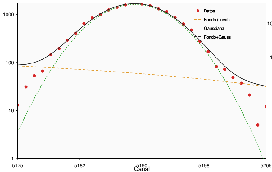
GeHP: descomposicion del ajuste
