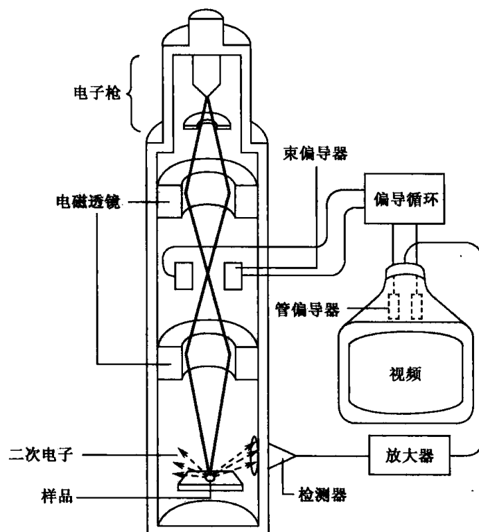
图 2-3 扫描电子显微镜的光学系统
