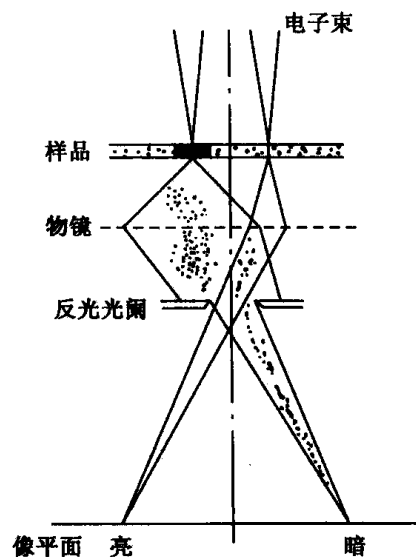
图 2-2 TEM 散射吸收(“质量-厚度反差成像原理”)(辛华, 2001)
