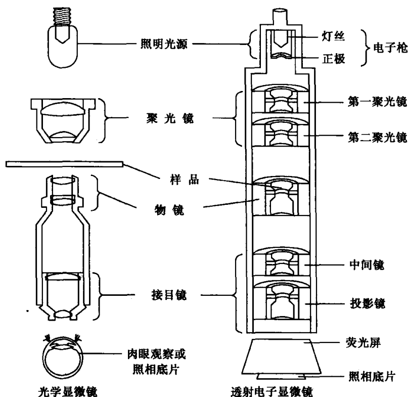
图 2-1 光学显微镜与透射电子显微镜（透射电镜）的结构比较
