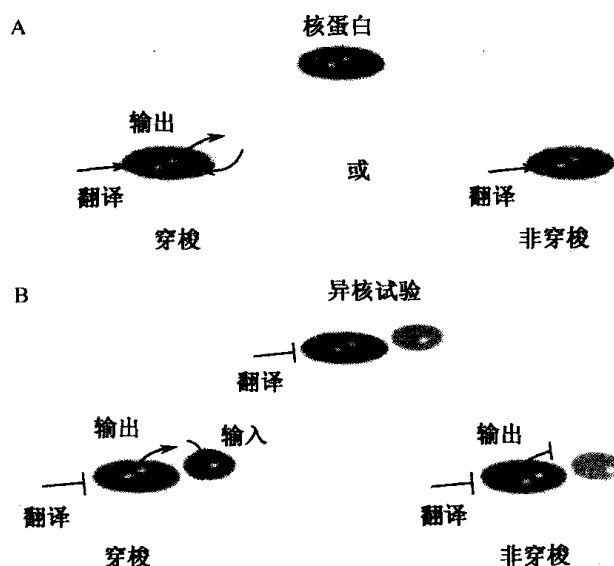
图 5-1 异核体测定法 (Celis, 2006)
